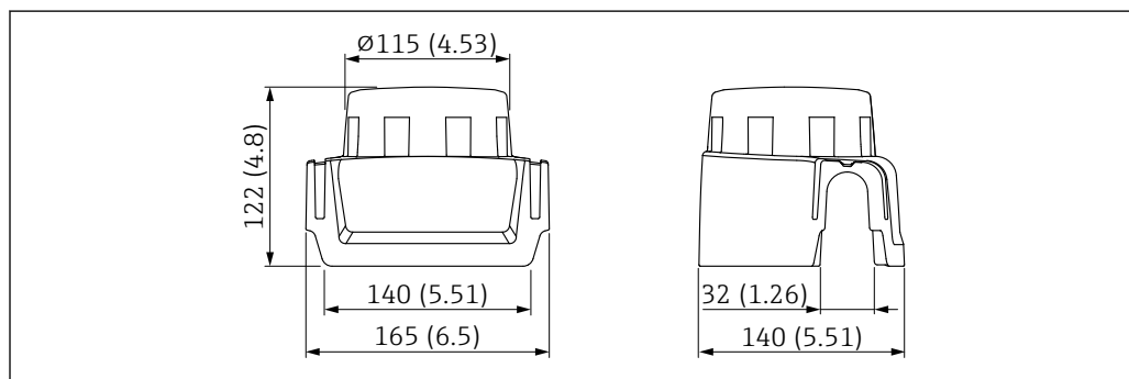
42 Dimensões da tampa de proteção contra tempo, plástico, XW111. Unidade de medida mm (in)
