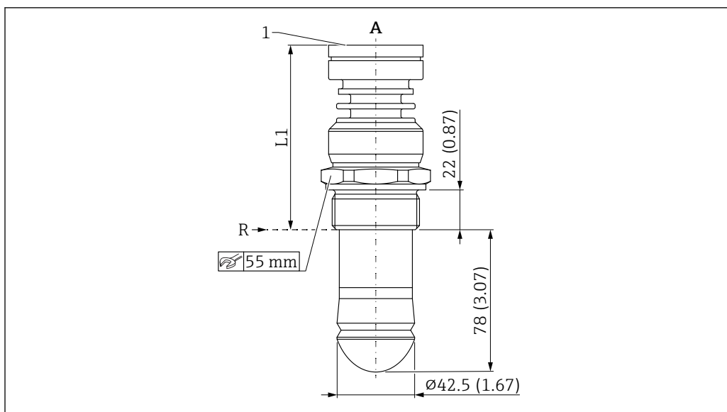
31 Dimensões da antena tipo drip-off 50 mm (2 in), conexão de processo de rosca
