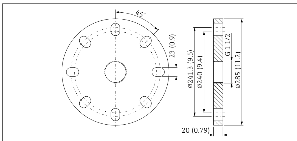
35 Dimensões da flange UNI 6"/DN150/150A. Unidade de medida mm (in)
