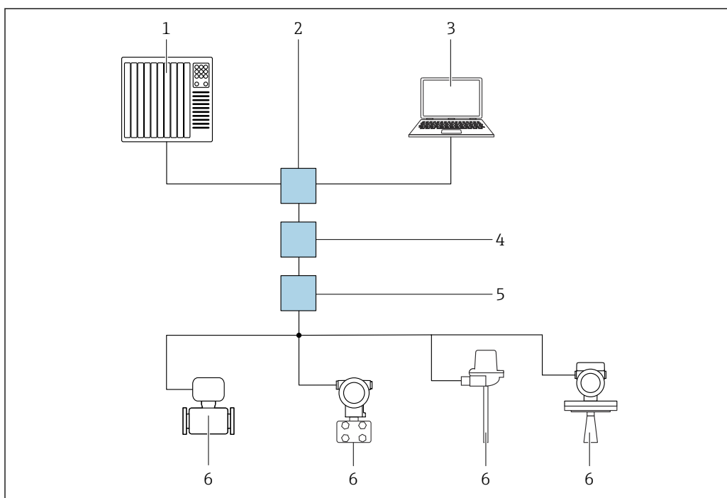
40 Opções para operação remota através da rede PROFIBUS com Ethernet-APL: topologia estrela
