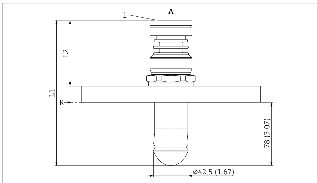
32 Dimensões da antena tipo drip-off 50 mm (2 in), conexão de processo de flange UNI. Unidade de medida mm (in)
