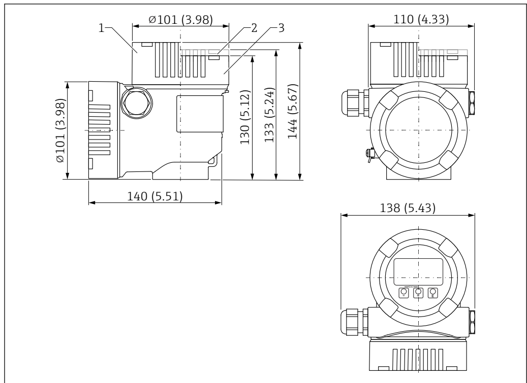
41 Dimensions ; boîtier à double compartiment en L, 316L ; avec raccord M20 et bouchon, plastique. Unité de mesure mm (in)
