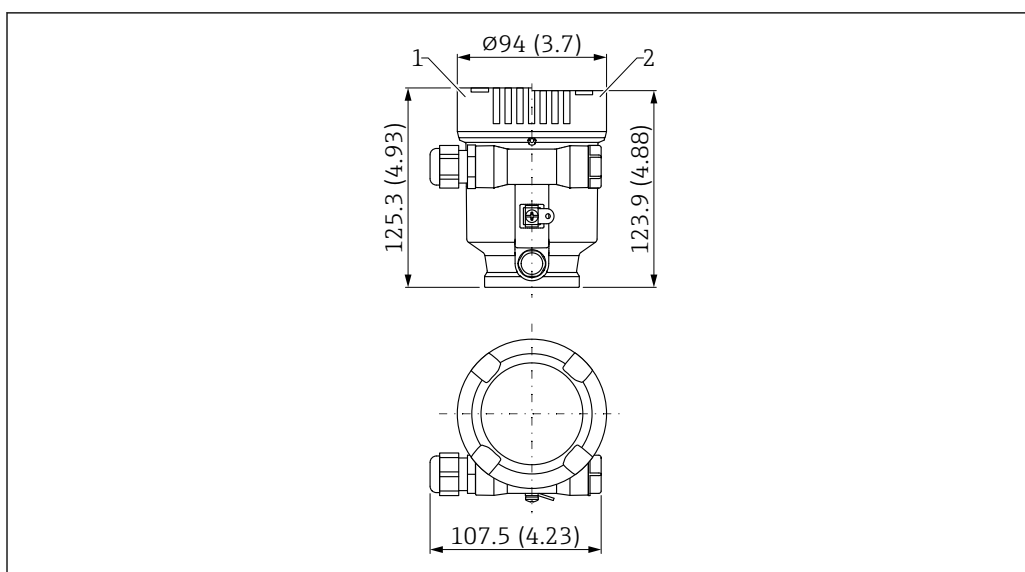
36 Dimensions ; boîtier à simple compartiment, plastique ; avec raccord M20 et bouchon, plastique. Unité de mesure mm (in)
