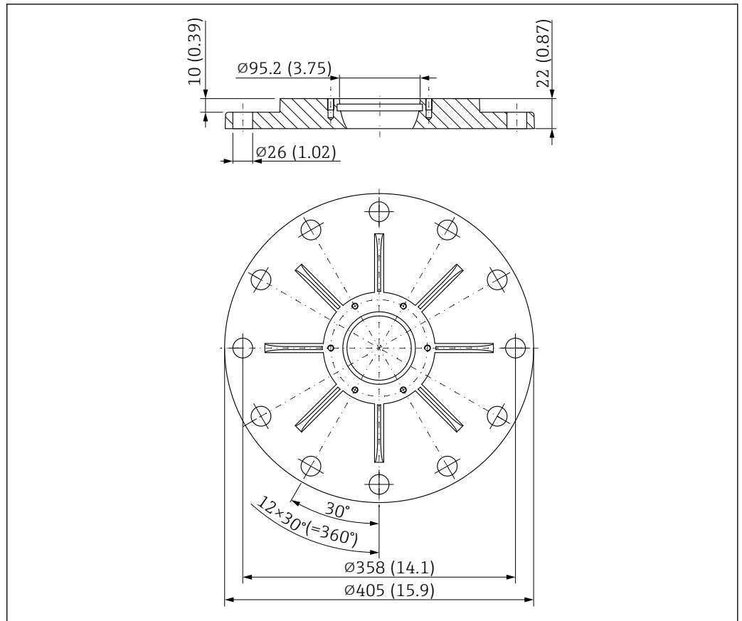
47 Dimensions de la bride UNI 10"/DN250/250A pour antennes avec dispositif d'orientation. Unité de mesure mm (in)
