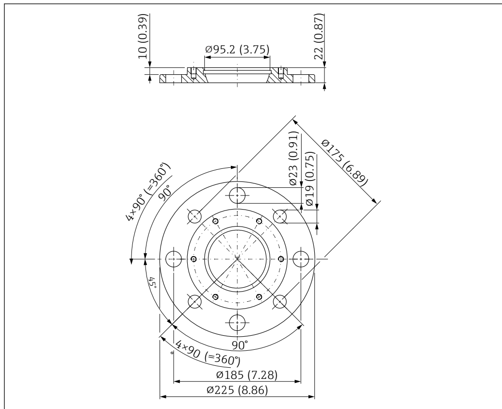
57 Dimensions de la bride UNI 4"/DN100/100A pour antennes avec dispositif d'orientation. Unité de mesure mm (in)
