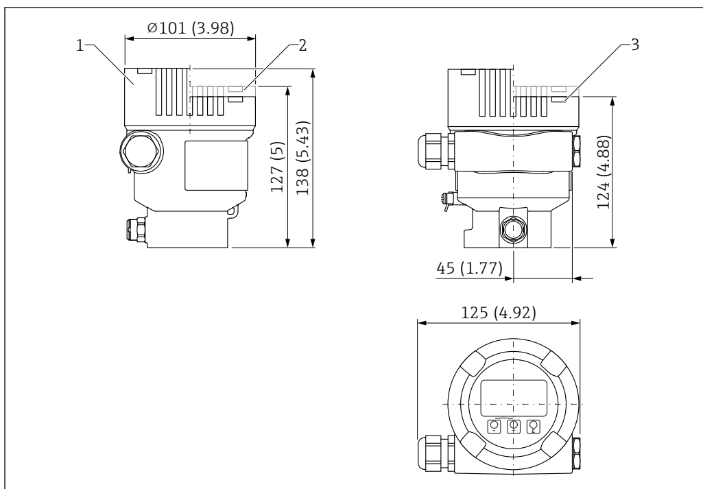
37 Dimensions ; boîtier à simple compartiment, aluminium, revêtu ; avec raccord M20 et bouchon, plastique. Unité de mesure mm (in)
