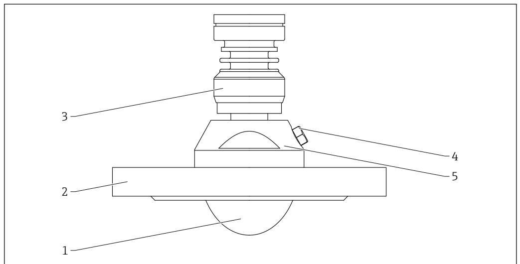
64 Material; antena, soporte para montaje enrasado, 80 mm (3 in), con brida y conexión de aire de purga. Unidad de medida mm (in)
