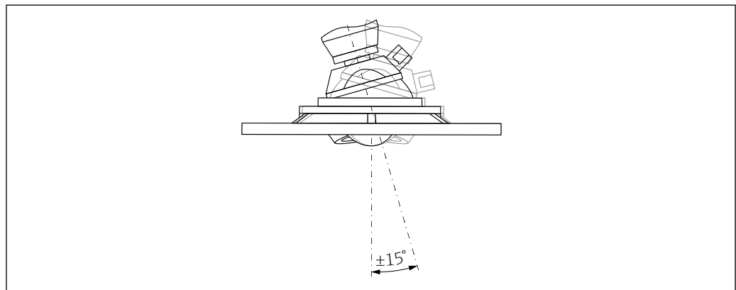
10 Soporte para montaje enrasado de la antena con unidad de alineación
