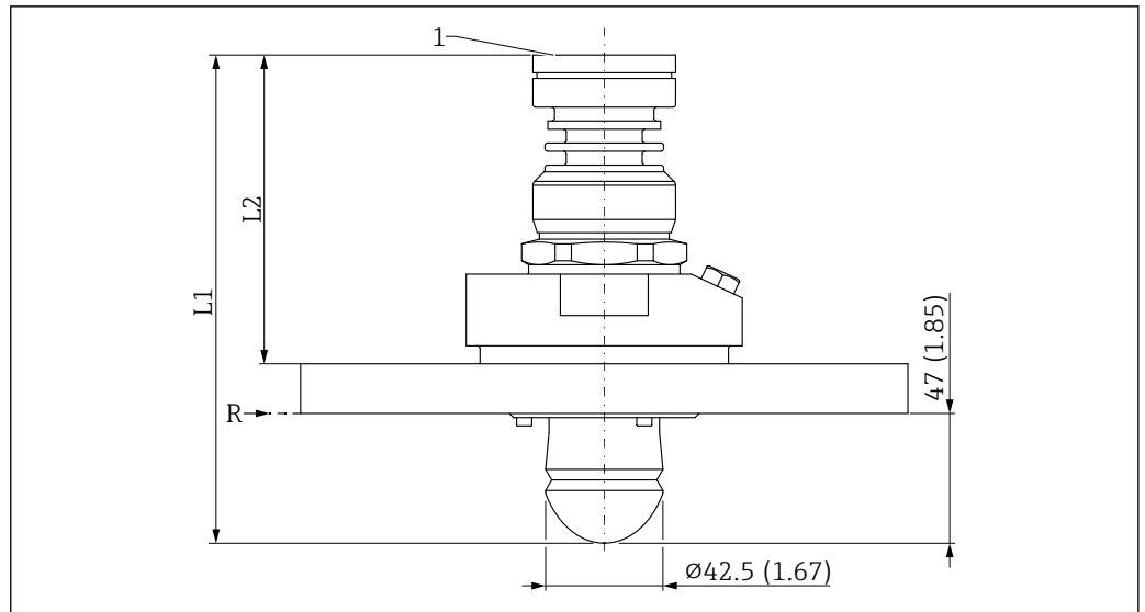
48 Medidas de la antena de goteo, PTFE, 50 mm (2 in), con brida UNI y conexión de aire de purga. Unidad de medida mm (in)
