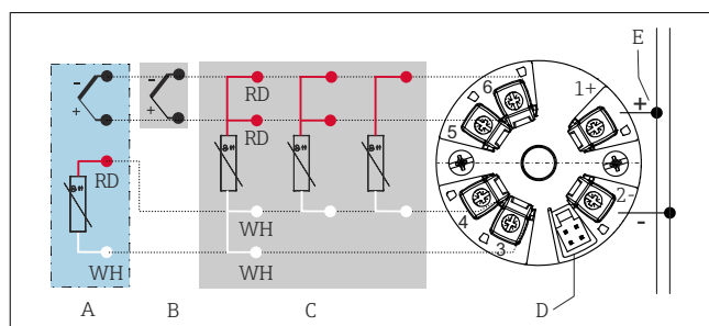
▣ 4 Klemmenbelegung Kopftransmitter
