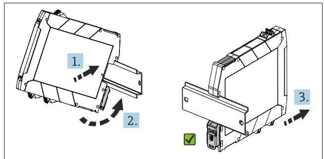
3 Montage Hutschienentransmitter
