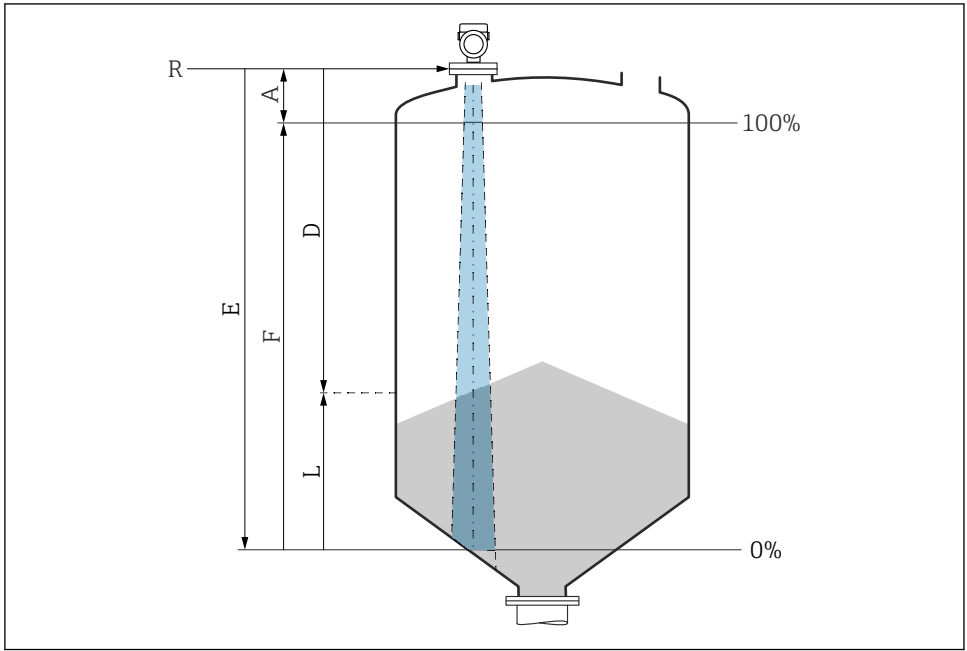
☐ 16 분체 레벨 측정 구성 파라미터
