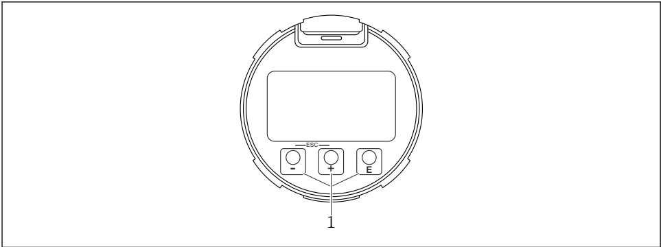
10 광학 작동 키(1)가 있는 그래픽 디스플레이
