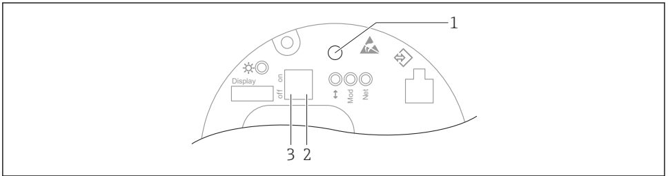
☐ 9 Ethernet-APL 전자 부속품의 작동 키 및 DIP 스위치
