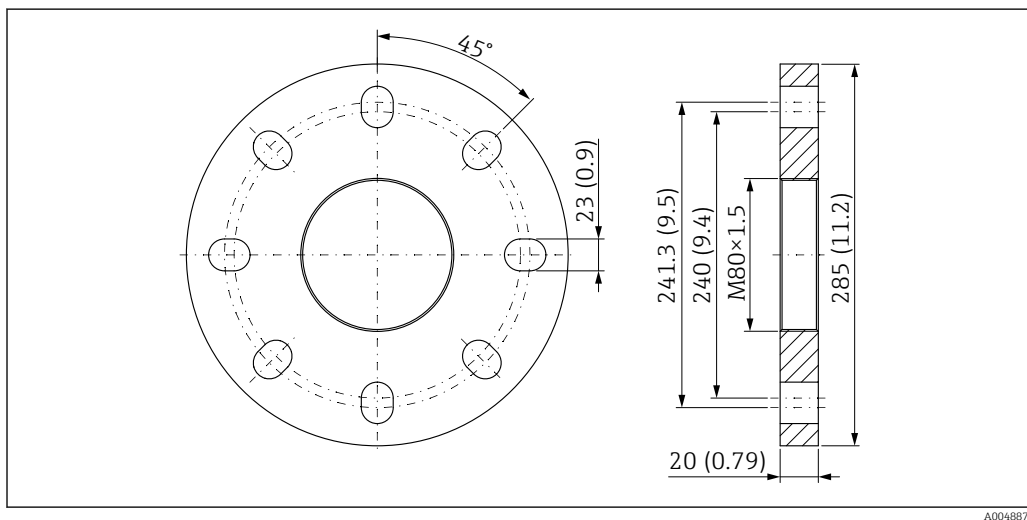
59 Flangia UNI 6"/DN150/150A per antenna drip-off, PTFE, 50 mm (2 in) con collegamento dell'aria di pulizia. Unità di misura mm (in)
