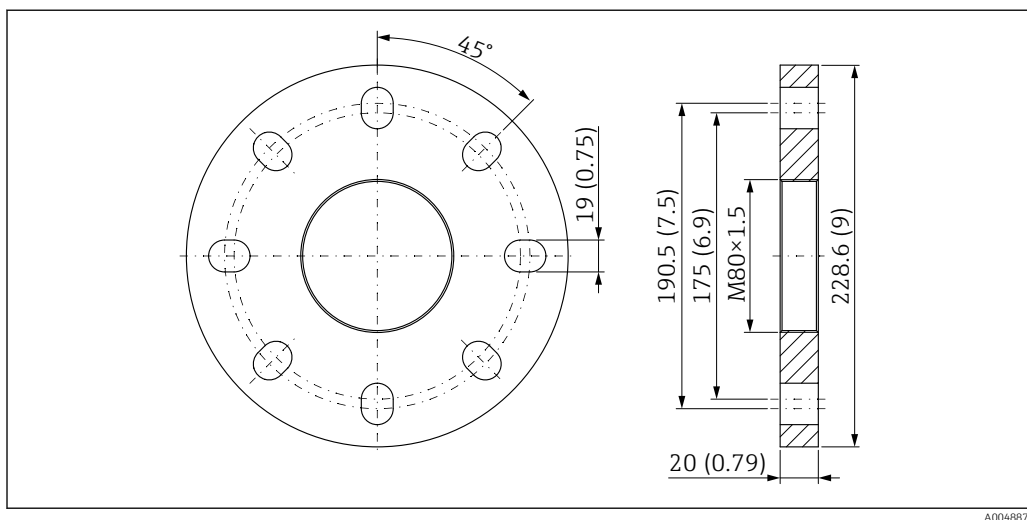
58 Flangia UNI 4"/DN100/100A per antenna drip-off, PTFE, 50 mm (2 in) con collegamento dell'aria di pulizia. Unità di misura mm (in)
