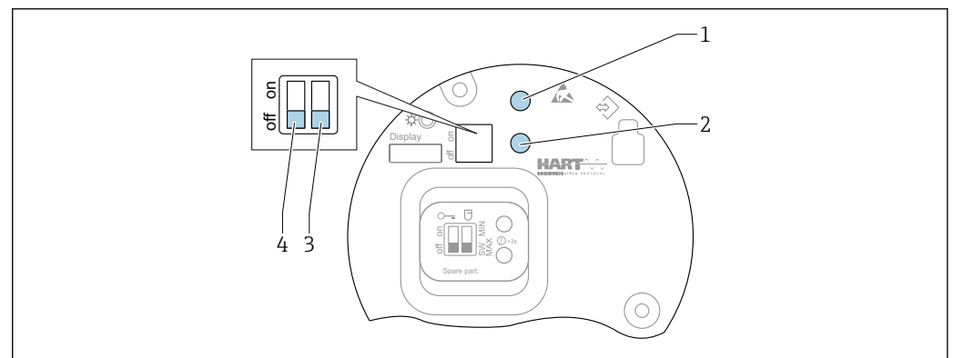
75 Tasti operativi e microinterruttori DIP sull'inserto elettronico HART
