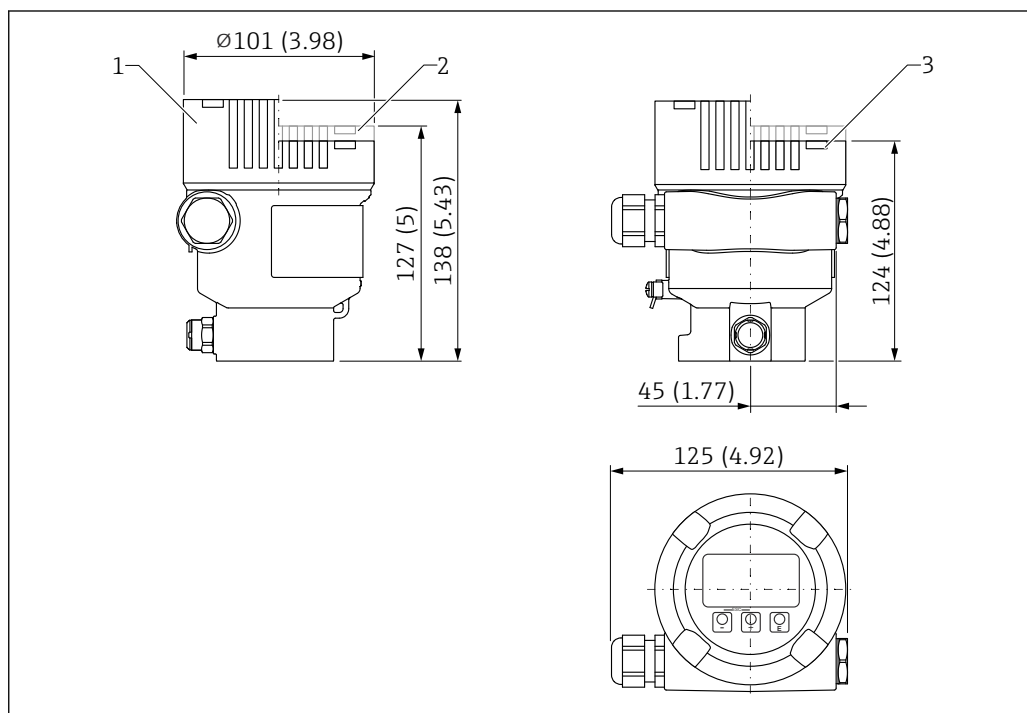
45 Dimensioni; custodia a vano unico, in alluminio, rivestita; completa di raccordo M20 e tappo in plastica. Unità di misura mm (in)
