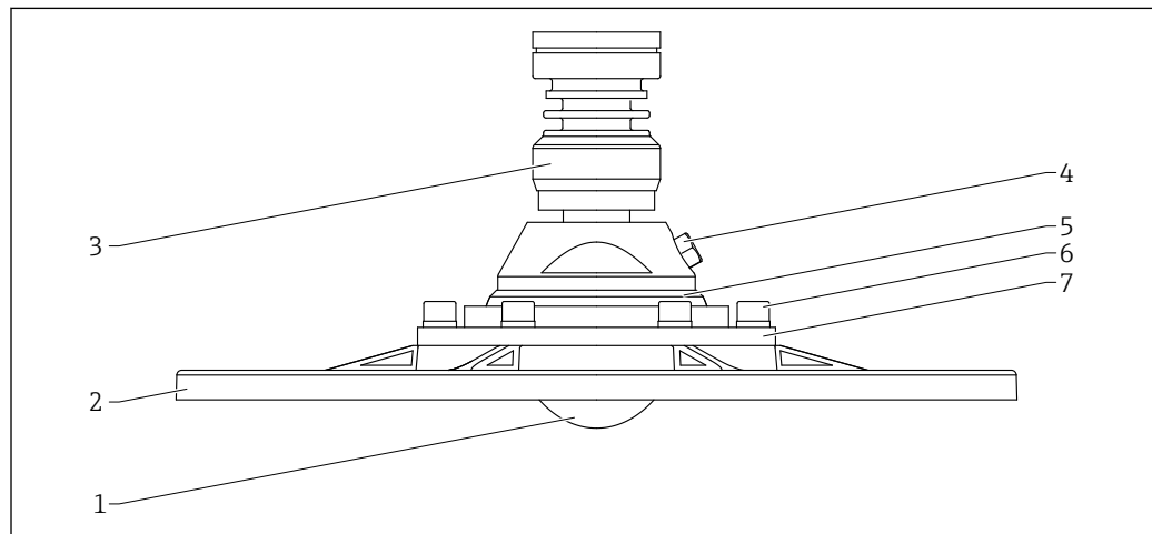
74 Materiale, antenna, flush mounted, 80 mm (3 in), con flangia UNI, unità di puntamento e collegamento dell'aria di pulizia
