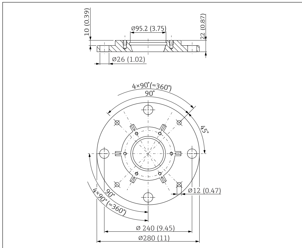
66 Dimensioni della flangia UNI 6"/DN150/150A per antenne con unità di puntamento. Unità di misura mm (in)
