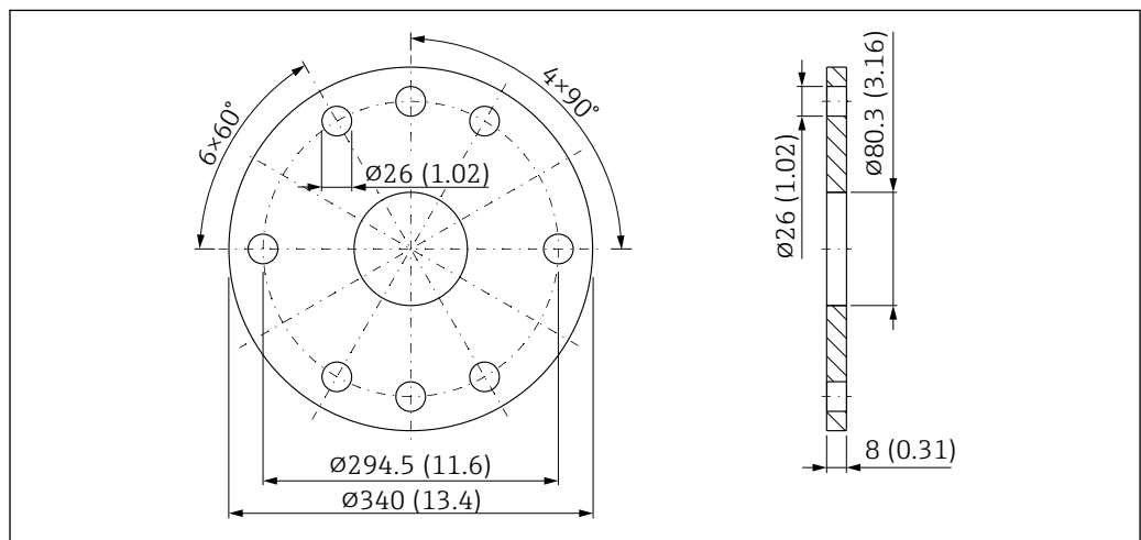
62 Dimensioni della flangia UNI 8"/DN200/200A per antenna DN80 con collegamento dell'aria di pulizia. Unità di misura mm (in)
