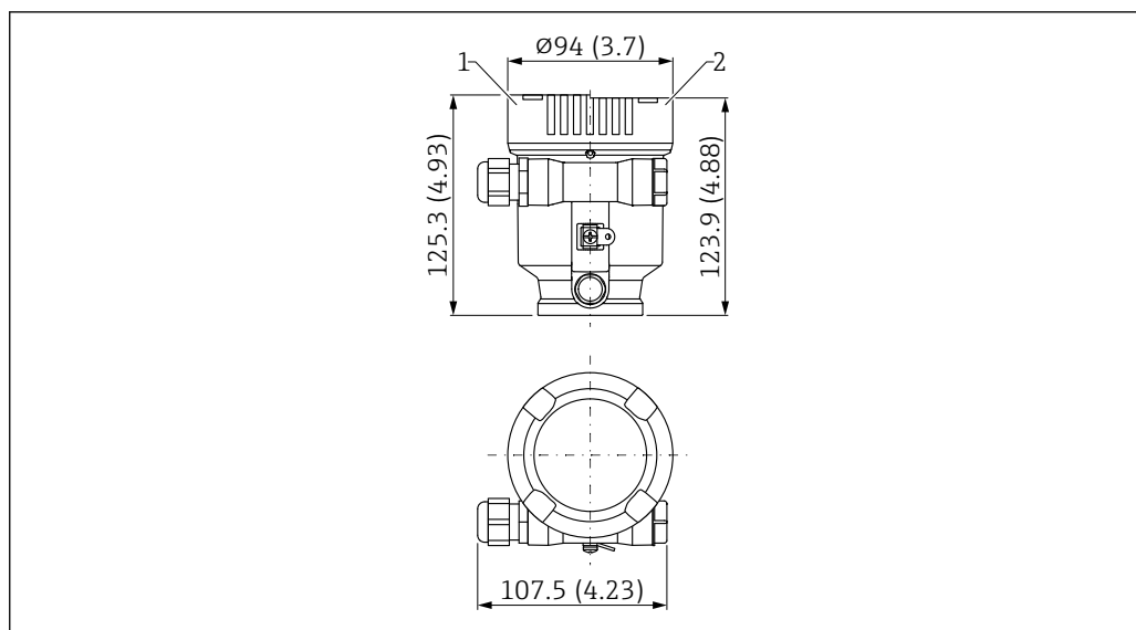
44 Dimensioni; custodia a vano unico, in plastica; completa di raccordo M20 e tappo in plastica. Unità di misura mm (in)
