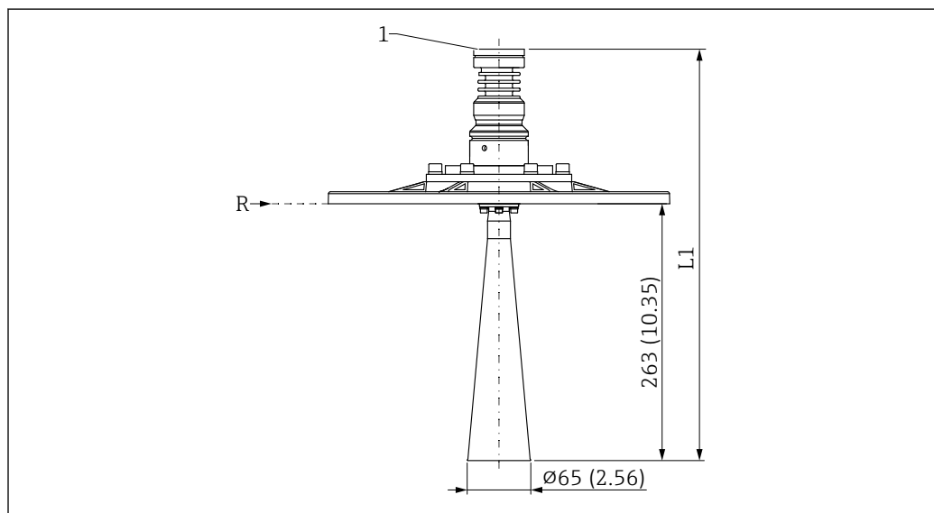
51 Dimensioni dell'antenna a cono DN65, con flangia UNI e unità di puntamento. Unità di misura mm (in)
