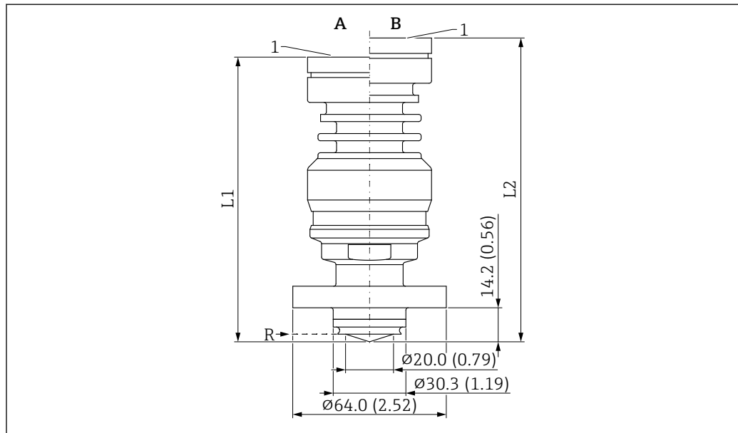
53 Medidas del soporte para montaje enrasado de la antena con revestimiento, PEEK, 20 mm (0,75 in), NEUMO BioControl D25. Unidad de medida mm (in)
