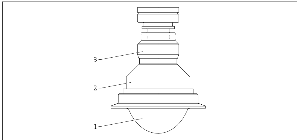
▣ 59 Material; soporte para montaje enrasado de la antena con revestimiento, PTFE, 80 mm (3 in), con triclamp ISO2852
