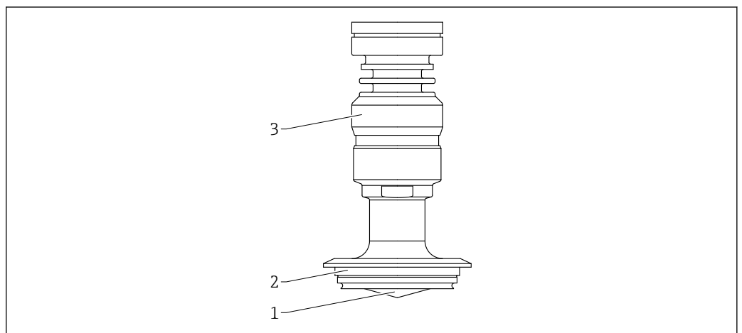
▣ 60 Material; soporte para montaje enrasado de la antena con revestimiento, PEEK, 40 mm (1,5 in), tubo Varivent N DN65-162
