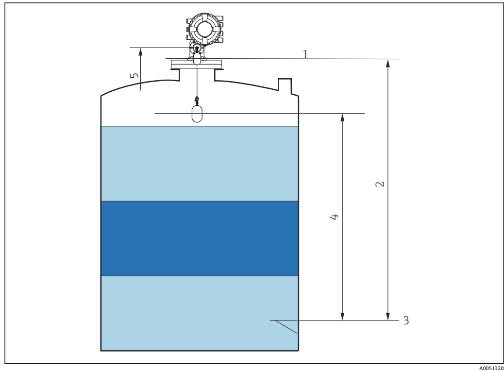
図 24 液面計測スタンバイゲージコマンドの実行時に液面上昇を待機するディスプレイサ
