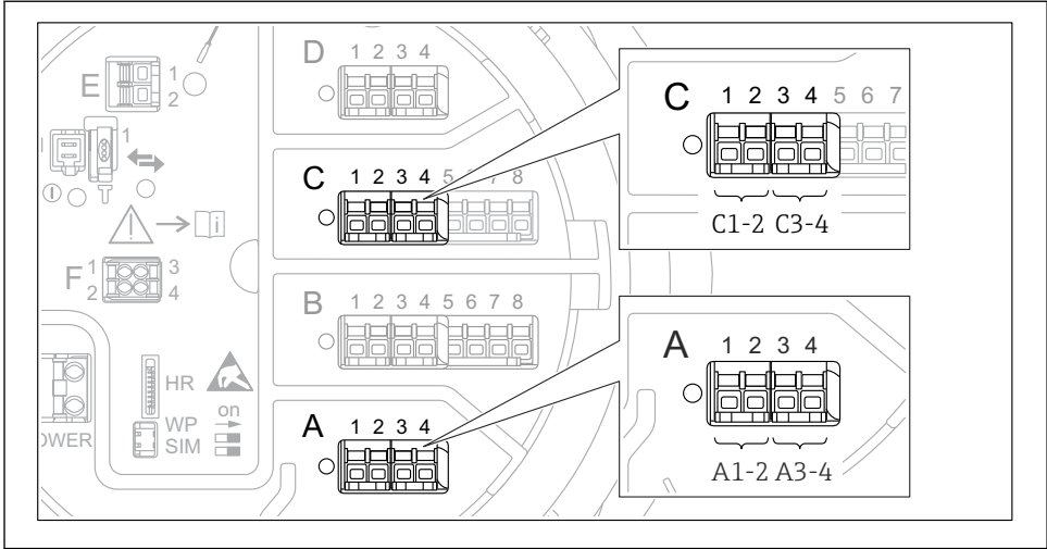
35 Mulige steder for de digitale I/O-modulene (eksempler), bestillingskoden definerer antallet og plasseringen av digitale inngangsmoduler.
