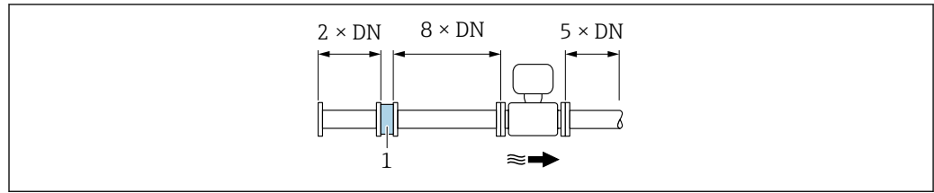
1 Стабилизатор потока
