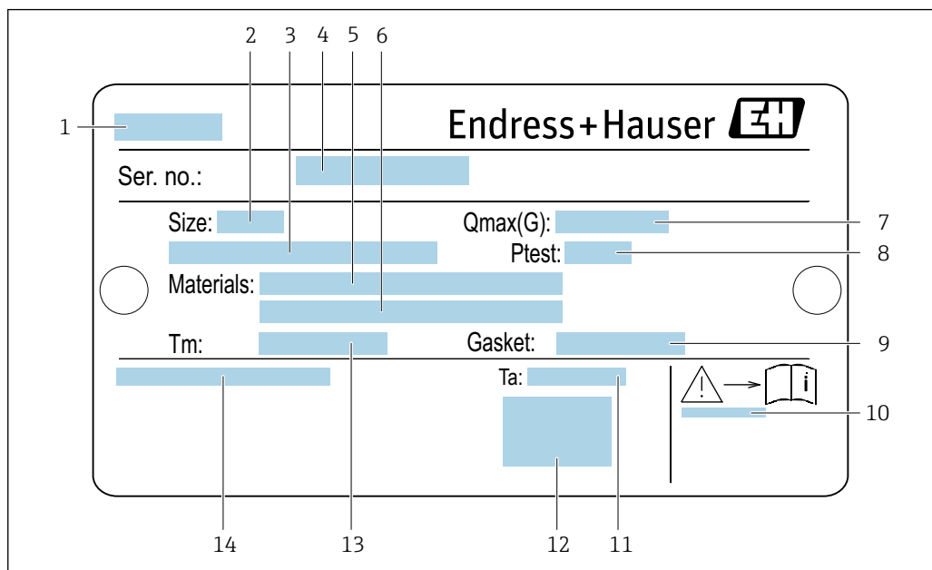
1 Пример заводской таблички датчика
