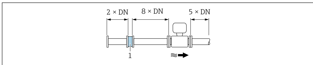
1 Стабилизатор потока
