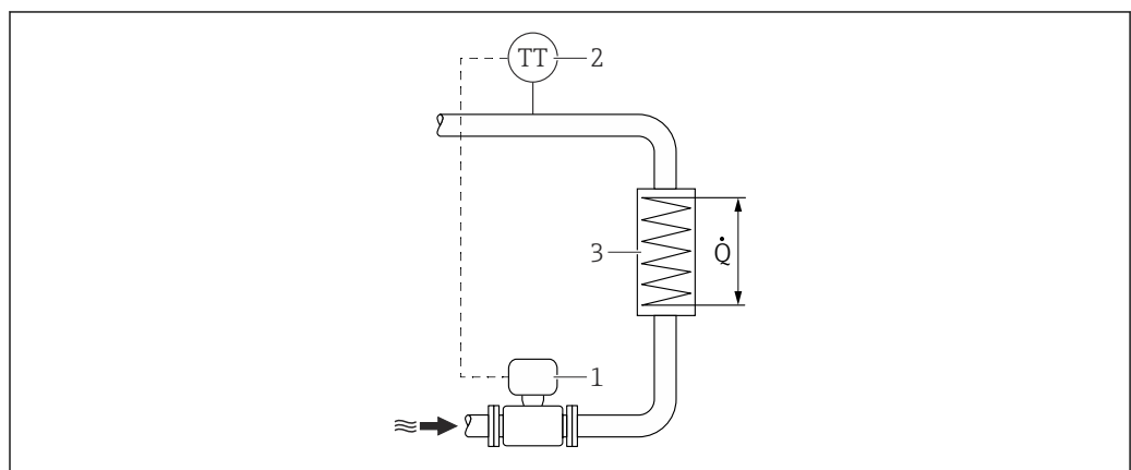
5 Схема измерения изменения количества теплоты для насыщенного пара и воды
