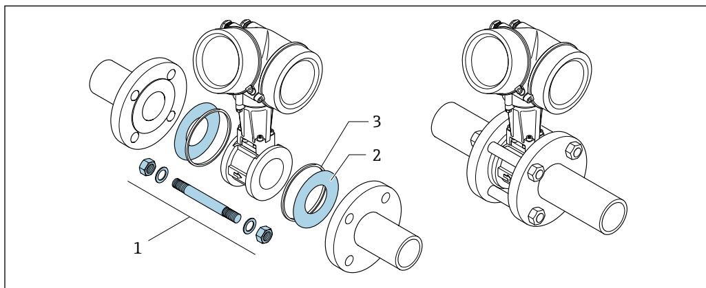
6 Монтажный комплект для бесфланцевого исполнения
