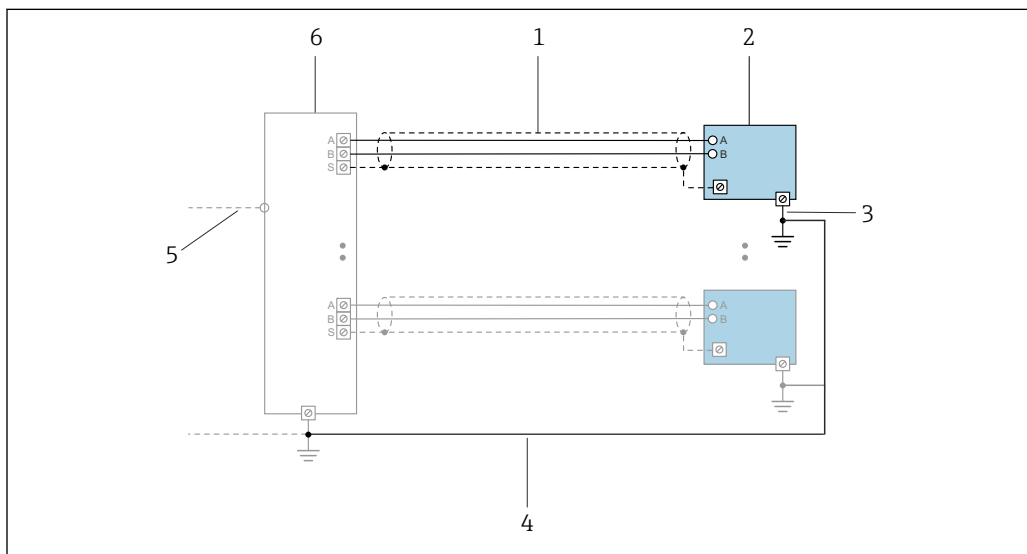
9 Пример подключения для PROFINET с Ethernet-APL
