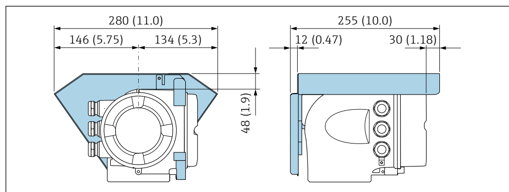
☞ 7 Unità ingegneristica, mm (in)
