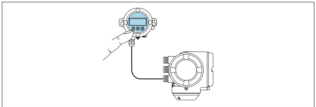
☞ 40 通过远传显示单元 DKX001 操作
