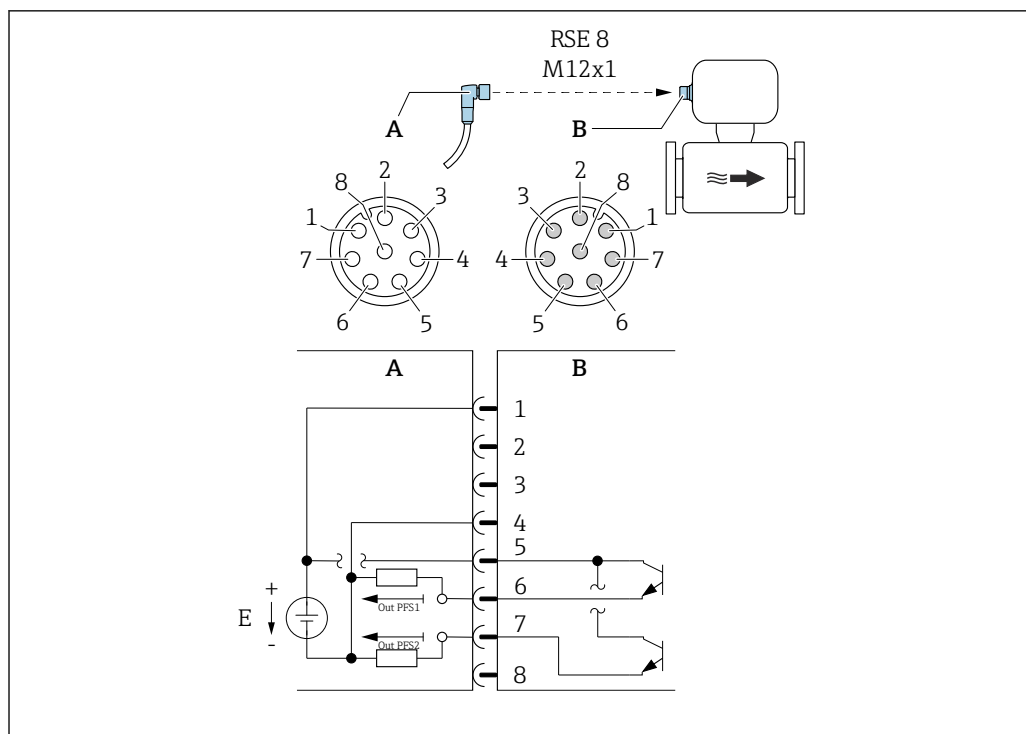
图 6 连接仪表
