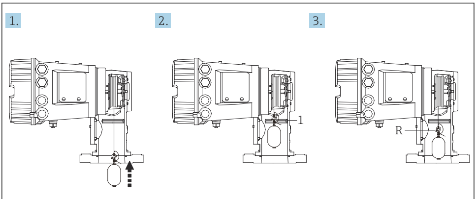
図 28 リファレンス校正シーケンス
