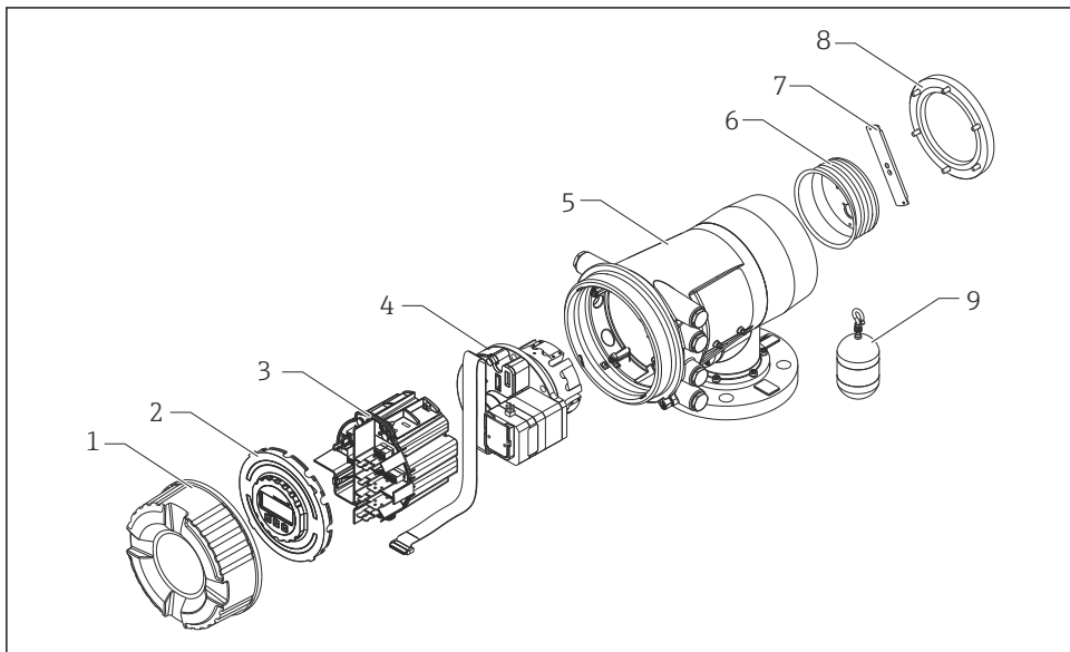
図 1 プロサーボ NMS80 の構成
