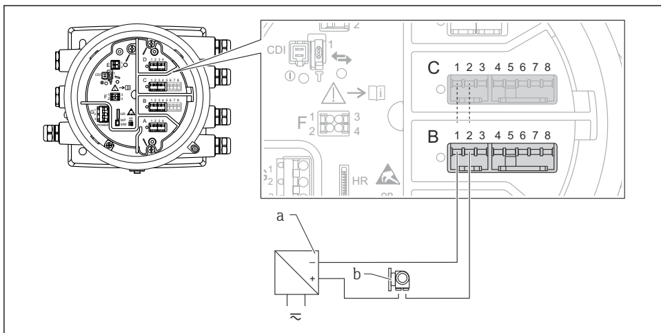
図 14 入力モードのアナログ I/O モジュールのパッシブ使用
