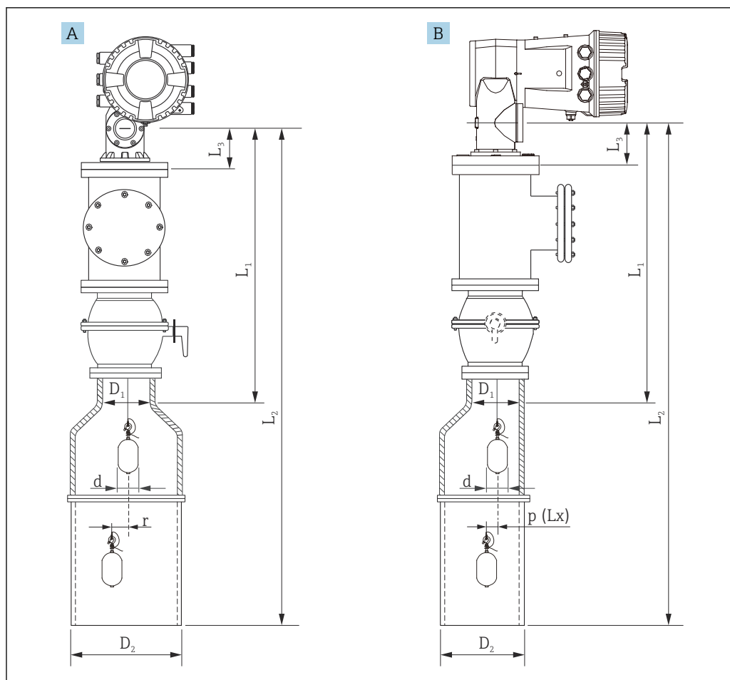
図 15 偏芯スティールウェルへの取付け
