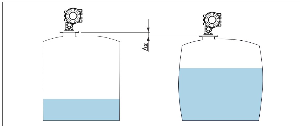
図 25 タンク基準高さの移動 \Delta x は、液体の静水圧によって生じるタンクシェルの膨張が原因で発生します。
