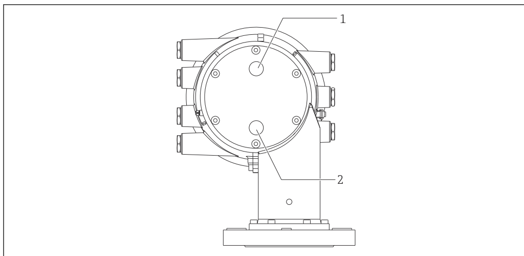
図 32 洗浄ノズルおよびガスパージノズル用の穴
