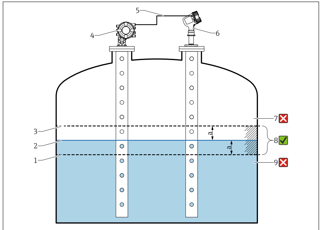
図 26 プロサーボ NMS8x を使用したアプリケーション事例
