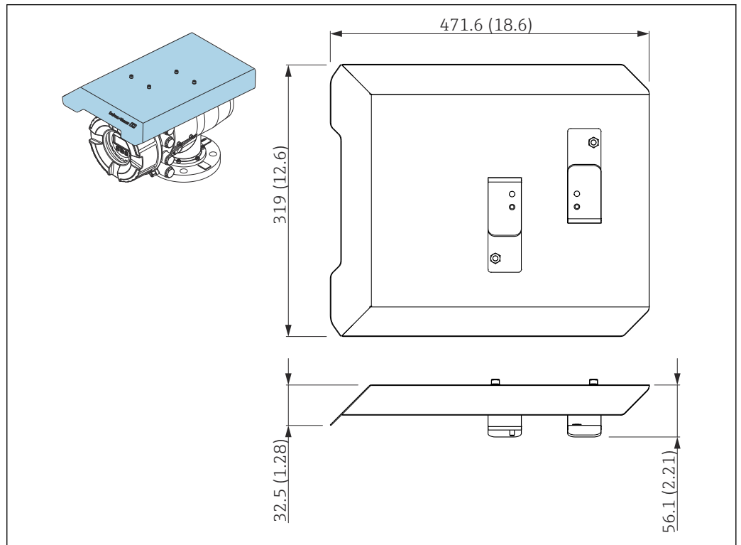
☐ 28 日除けカバー、寸法 : mm (in)
