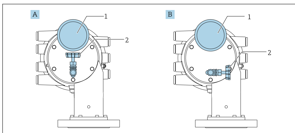
図 29 リリースバルブおよび圧力計の取付位置
