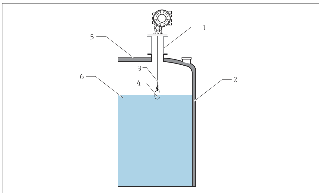
図 19 プロセスシーリング
