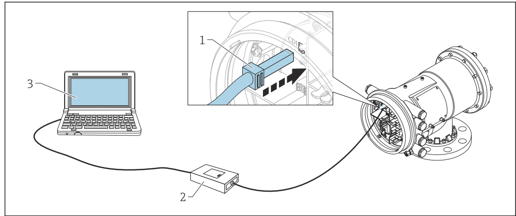
図 40 サービスインタフェース経由の操作
