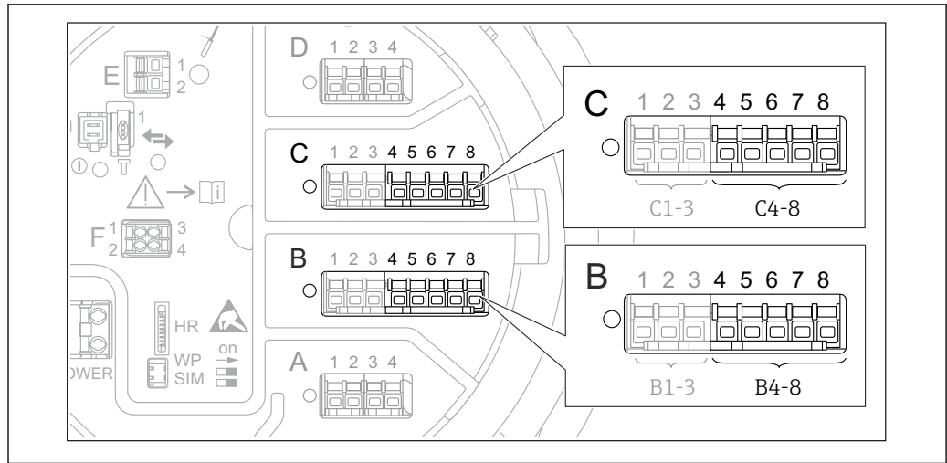
図 65 アナログ I/O モジュールの使用可能な端子。測温抵抗体を接続できます。機器のオーダーコードは、実際に存在するモジュールを示します → 図 47。
