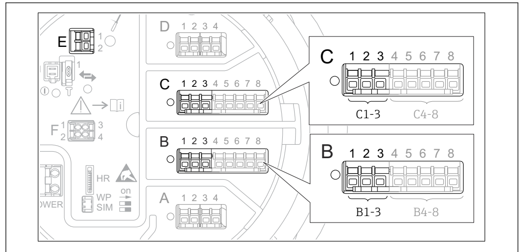
図 60 HART ループに使用可能な端子
