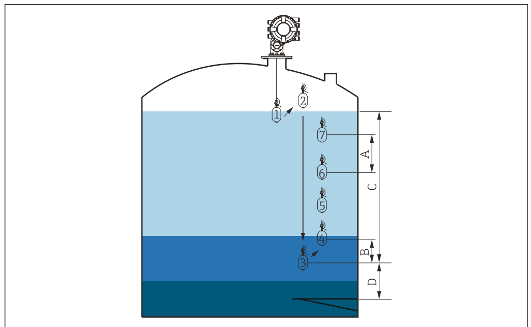
図 59 マニュアルプロファイルの移動（数字はディスプレイの移動順序を示します）
