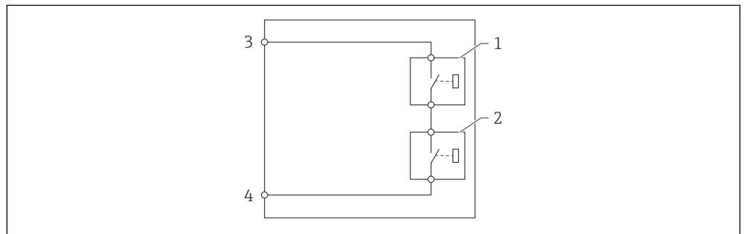
図 95 デジタル出力の 2 つのリレー
