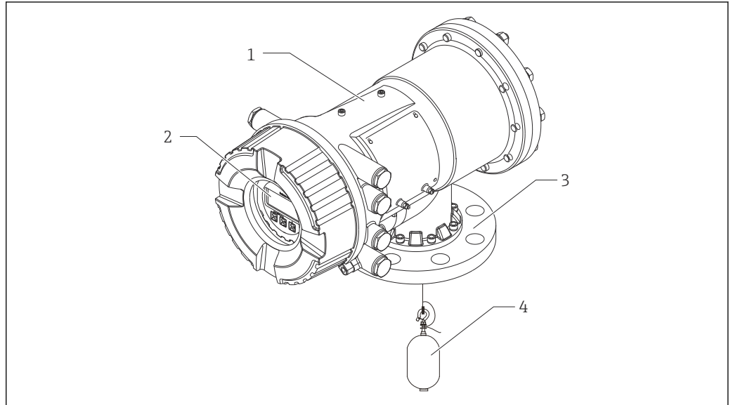
図 1 プロサーボ NMS81 の構成
