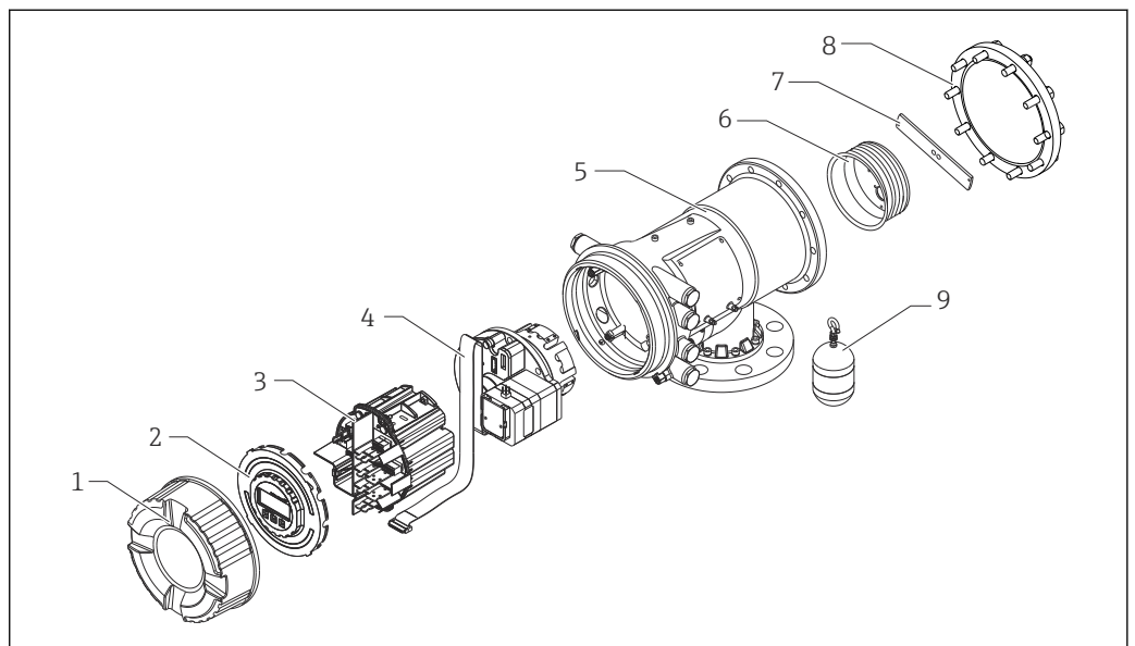
図 2 プロサーボ NMS81 の構成
