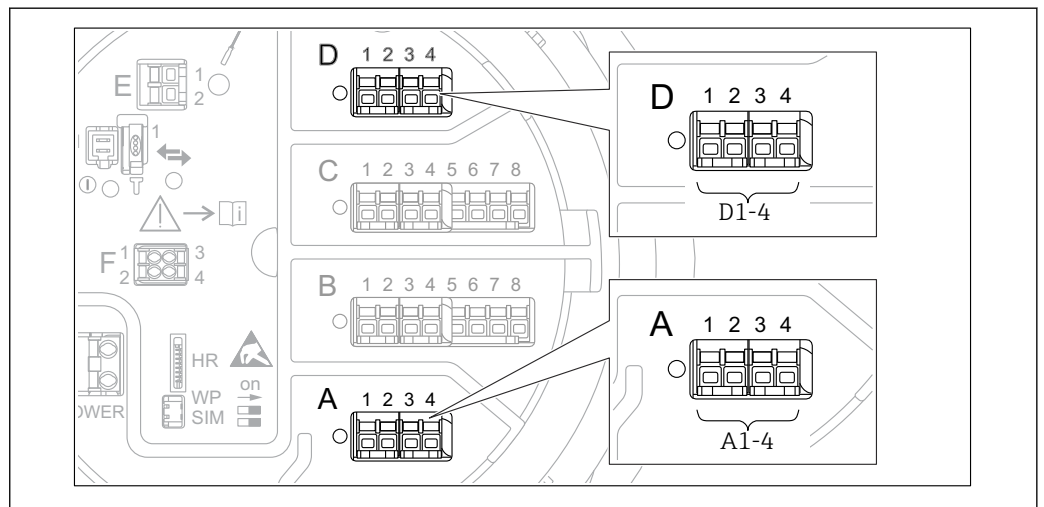
図 77 WM550 モジュールの使用可能な端子 (例)。機器バージョンに応じて、WM550 モジュールがスロット B または C に対応する場合があります → 図 47。
