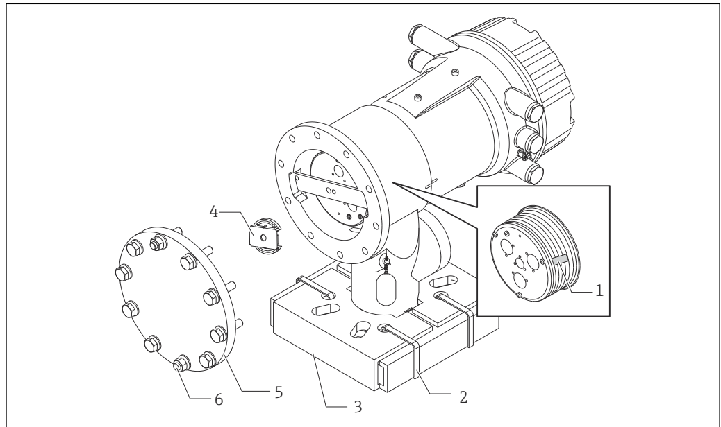
図 16 梱包材の取外し
