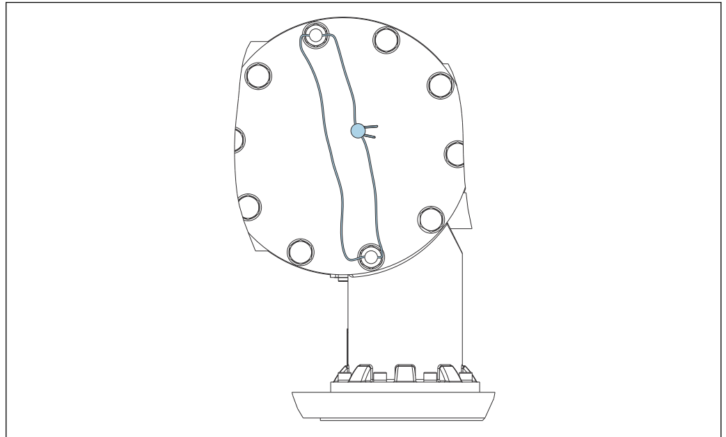
図 37 後部カバーのシーリング (例 : NMS81/NMS83)
