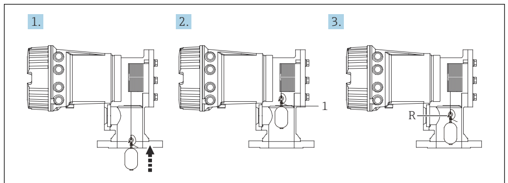
図 46 リファレンス校正シーケンス
