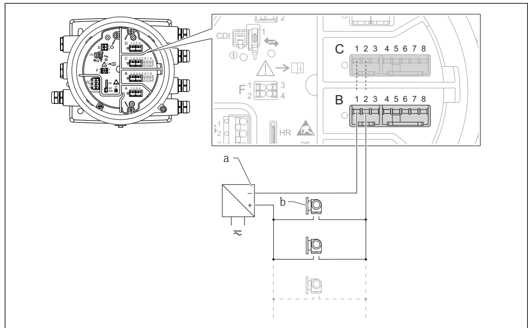
図 25 HART マスタモードのアナログ I/O モジュールのパスシブ使用
