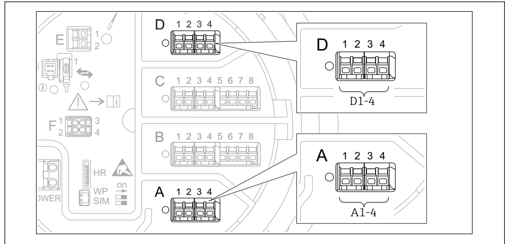
図 75 Modbus モジュールの使用可能な端子 (例)。機器バージョンに応じて、Modbus モジュールがスロット B または C に対応する場合があります → 図 47。
