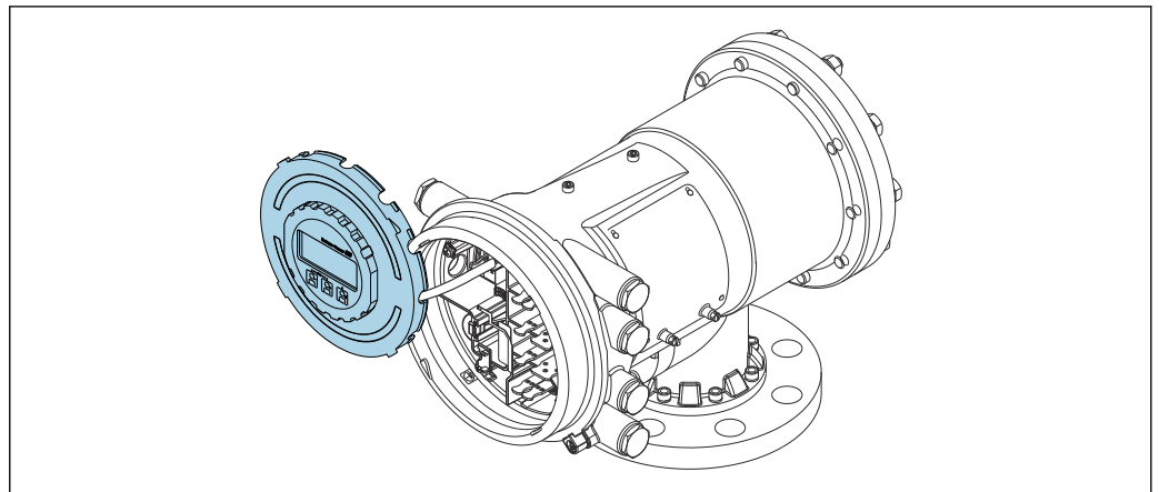
図 38 NMS81 : 端子室の縁に差し込まれた表示モジュール
