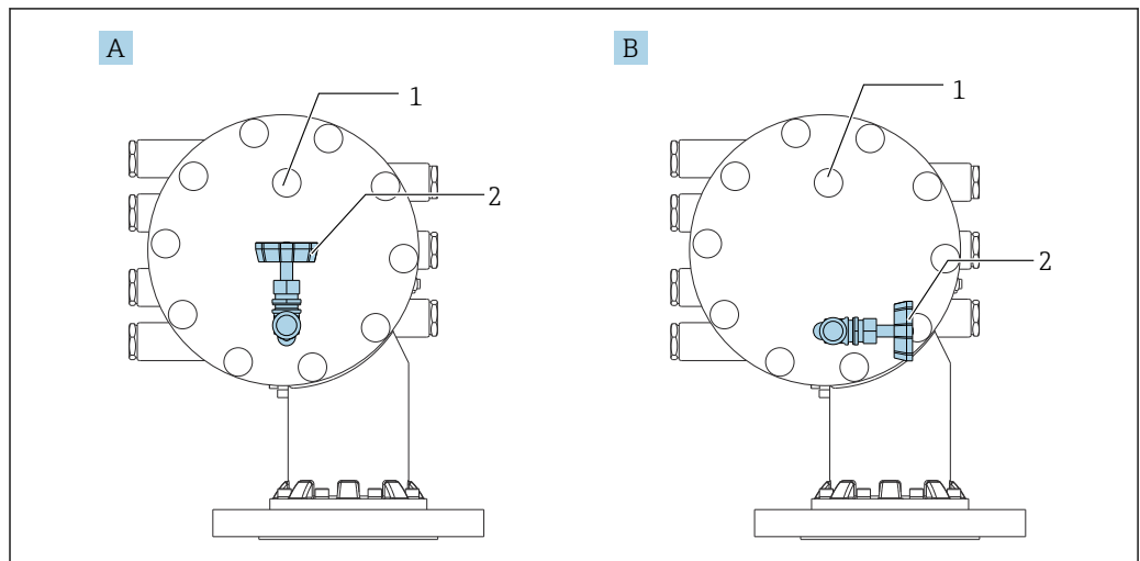
図 87 洗浄ノズルとリリーフバルブ
