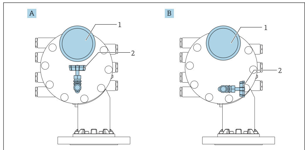
図 83 リリーフバルブおよび圧力計の取付位置
