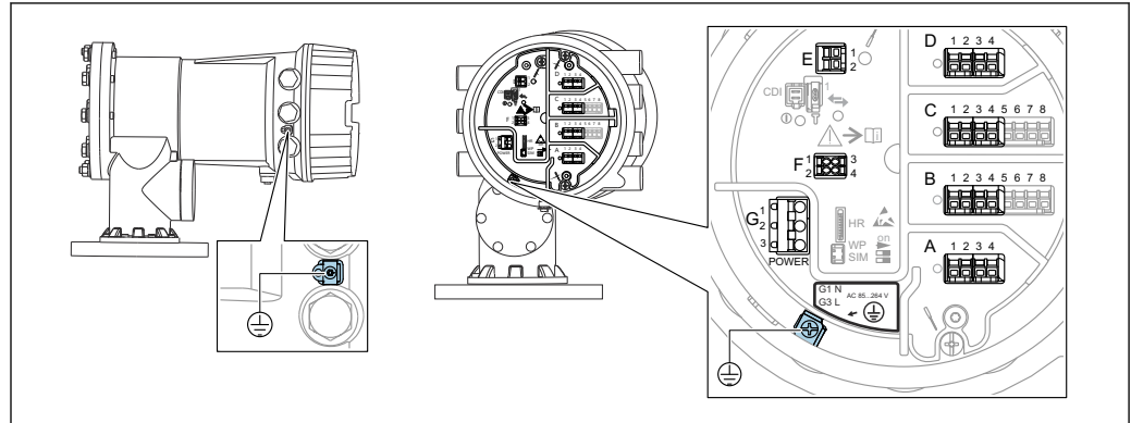
図 19 端子室（標準例）および接地端子
