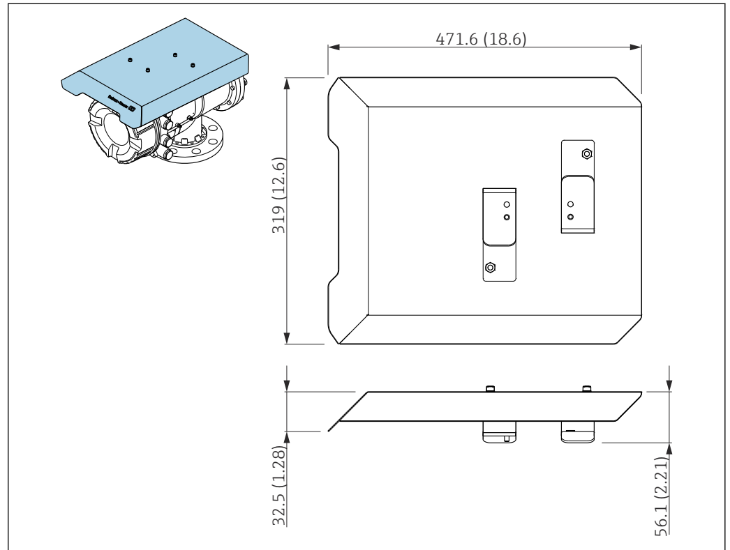
☒ 82 日除けカバー、寸法：mm (in)
