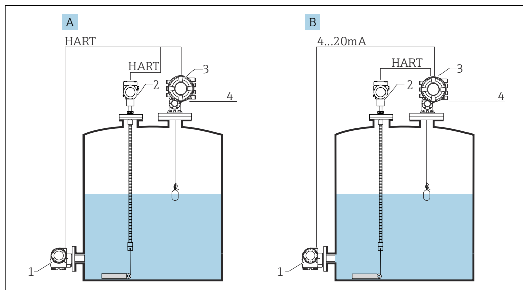
図 2 NMS80/NMS81 の計測システム
