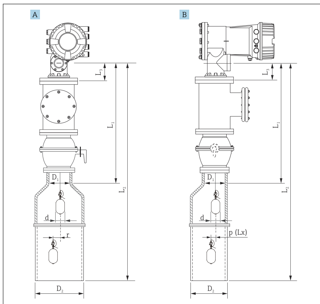
図 15 偏芯スティールウェルへの取付け
