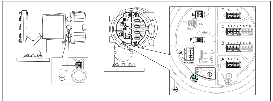
図 11 端子室（標準例）および接地端子
