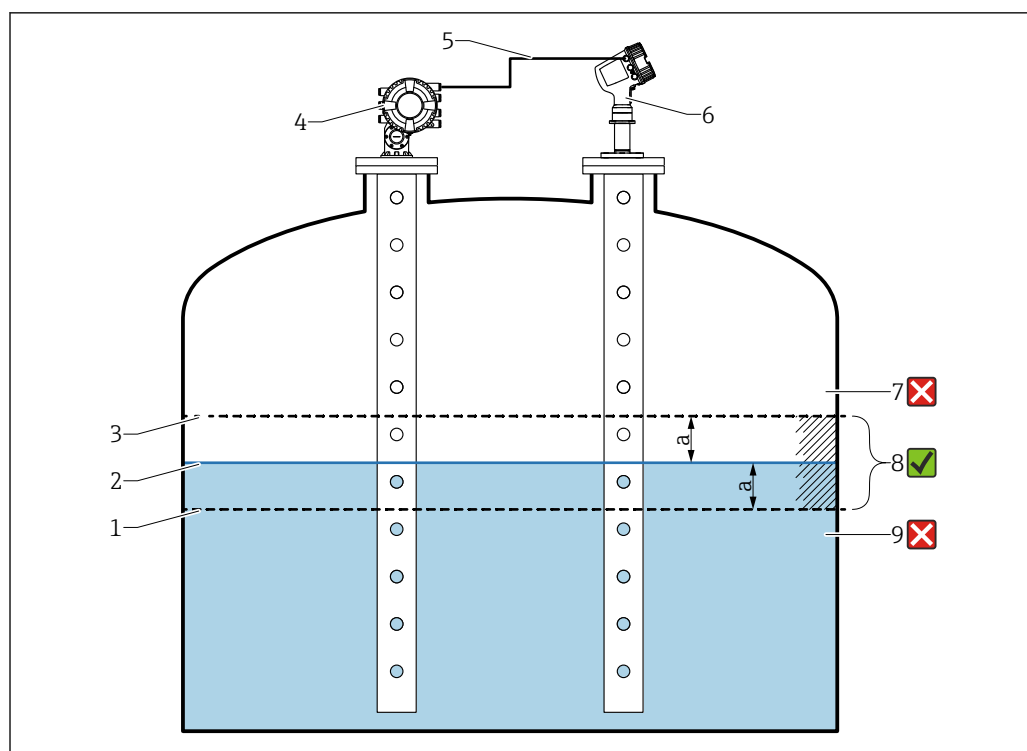
図 26 プロサーボ NMS8x を使用したアプリケーション事例
