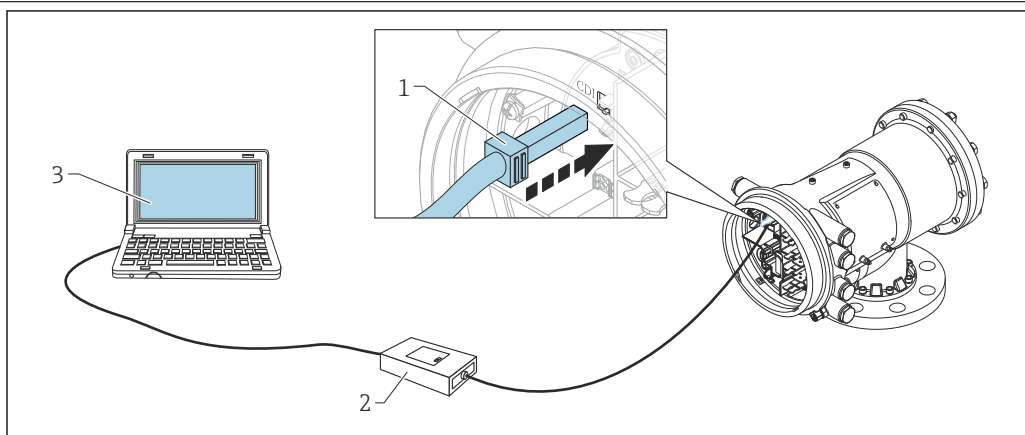
図 24 サービスインタフェース経由の操作
