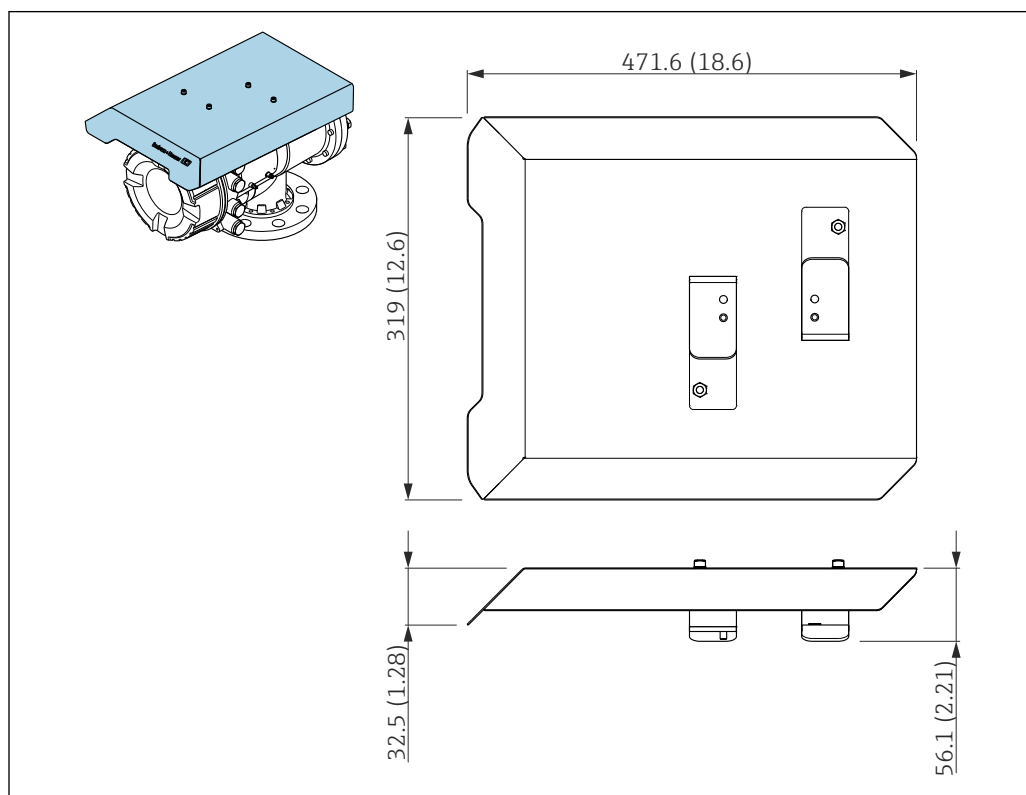
■ 28 日除けカバー、寸法：mm (in)
