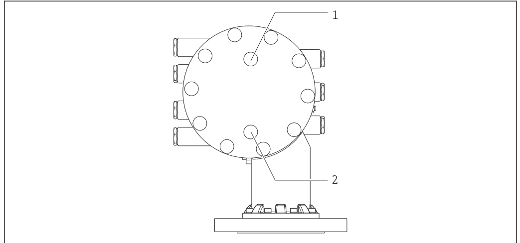
図 32 洗浄ノズルおよびガスパージノズル用の穴
