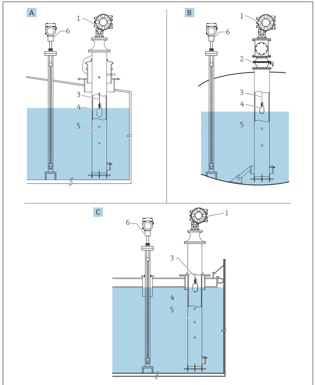
図 3 一般的なタンクの設置
