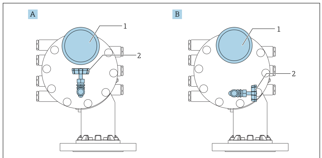
図 29 リリースバルブおよび圧力計の取付位置
