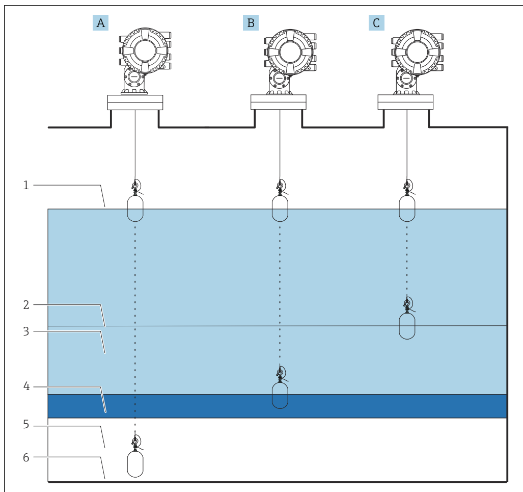
図 5 密度プロファイル測定
