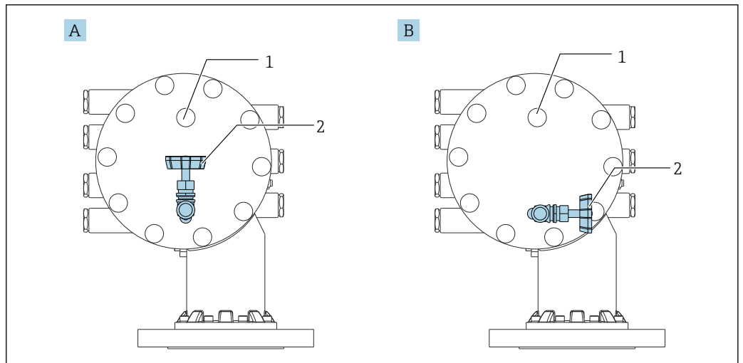
図 33 洗浄ノズルとリリースバルブ
