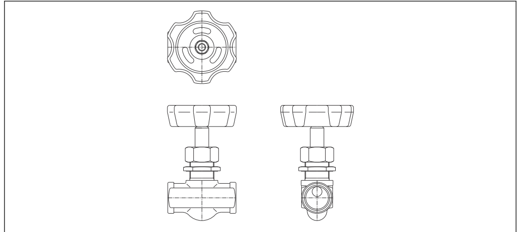
図 77 リリーフバルブ
