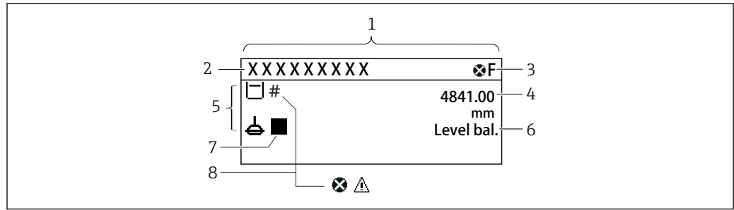
図 24 標準画面の一般的な表示（測定値表示部）
