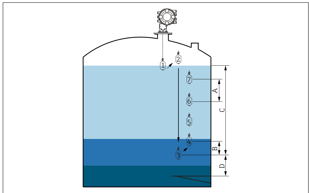
図 52 マニュアルプロファイルの移動（数字はディスプレイ上の移動順序を示します）
