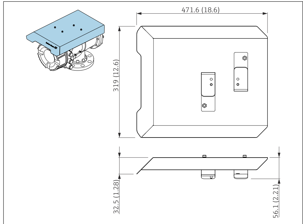
図 75 日除けカバー、寸法：mm (in)
