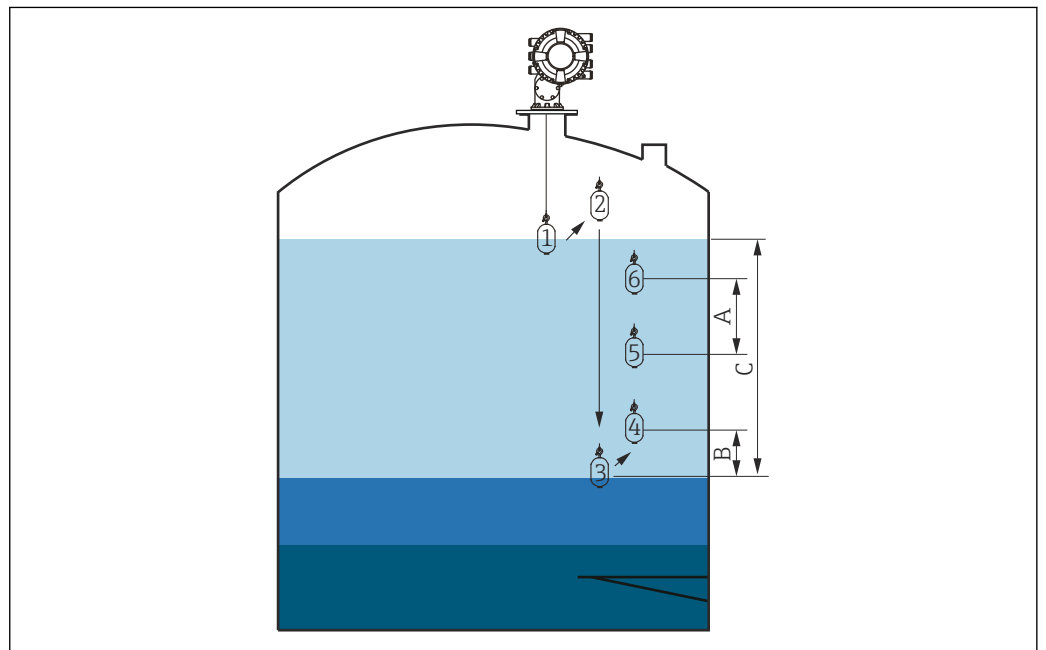
図 51 界面プロフィールの移動（数字はディスプレイサの移動順序を示します）
