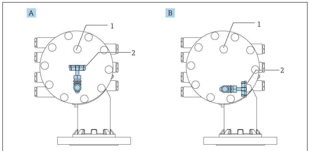
図 80 洗浄ノズルとリリーフバルブ
