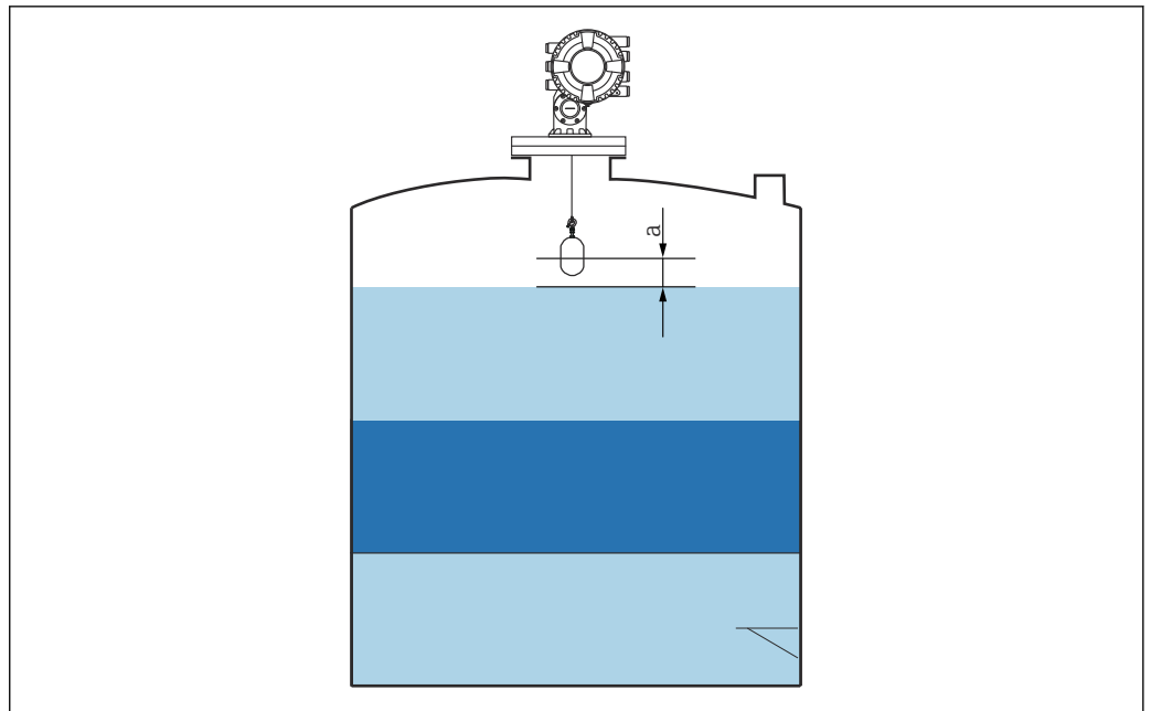
83 a : オフセットスタンバイ距離
