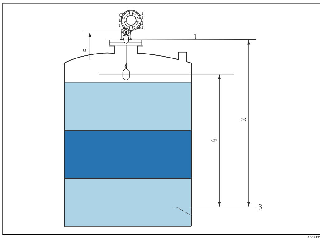
図 82 液面計測スタンバイゲージコマンドの実行時に液面上昇を待機するディスプレイサ
