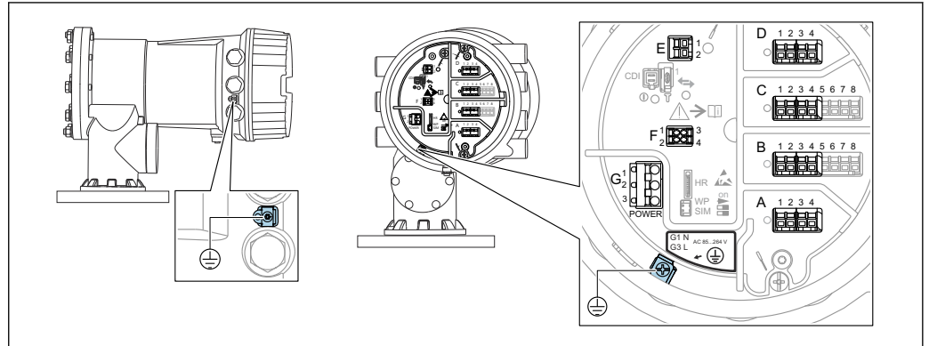
図 12 端子室（標準例）および接地端子
