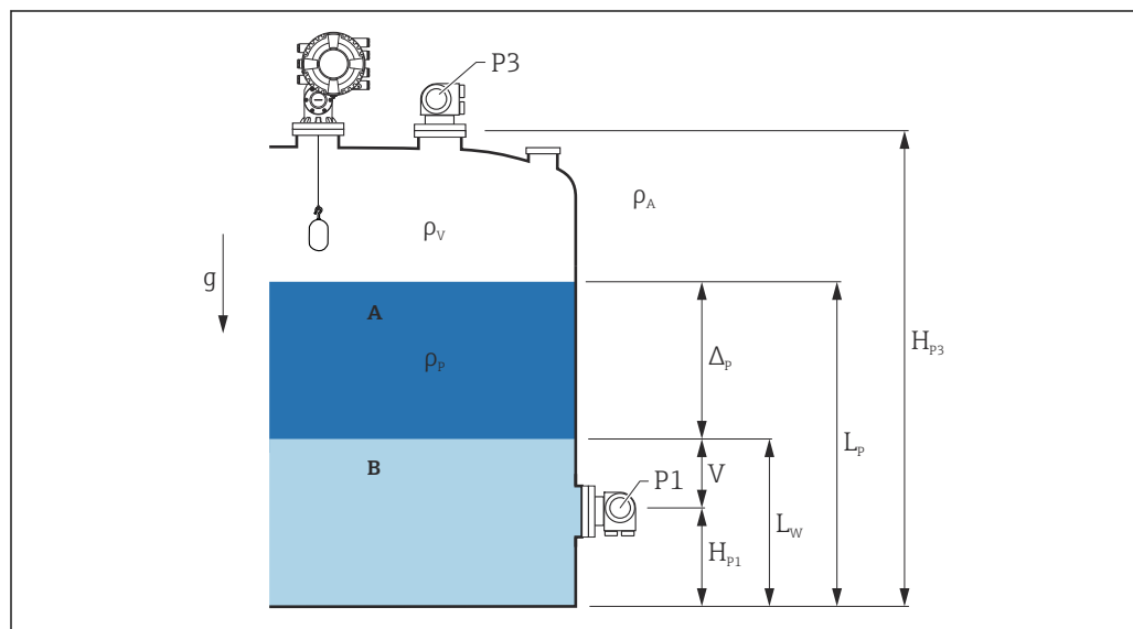
図 93 HTMS パラメータ
