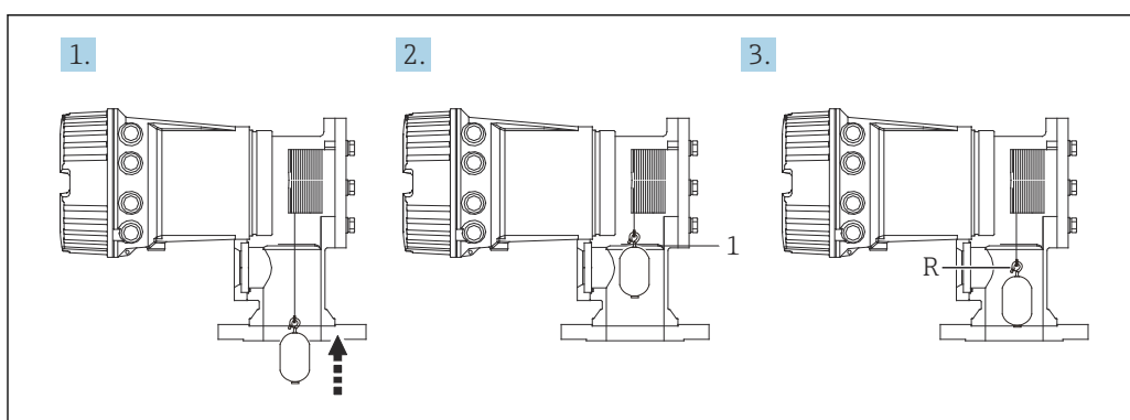
図 39 リファレンス校正シーケンス
