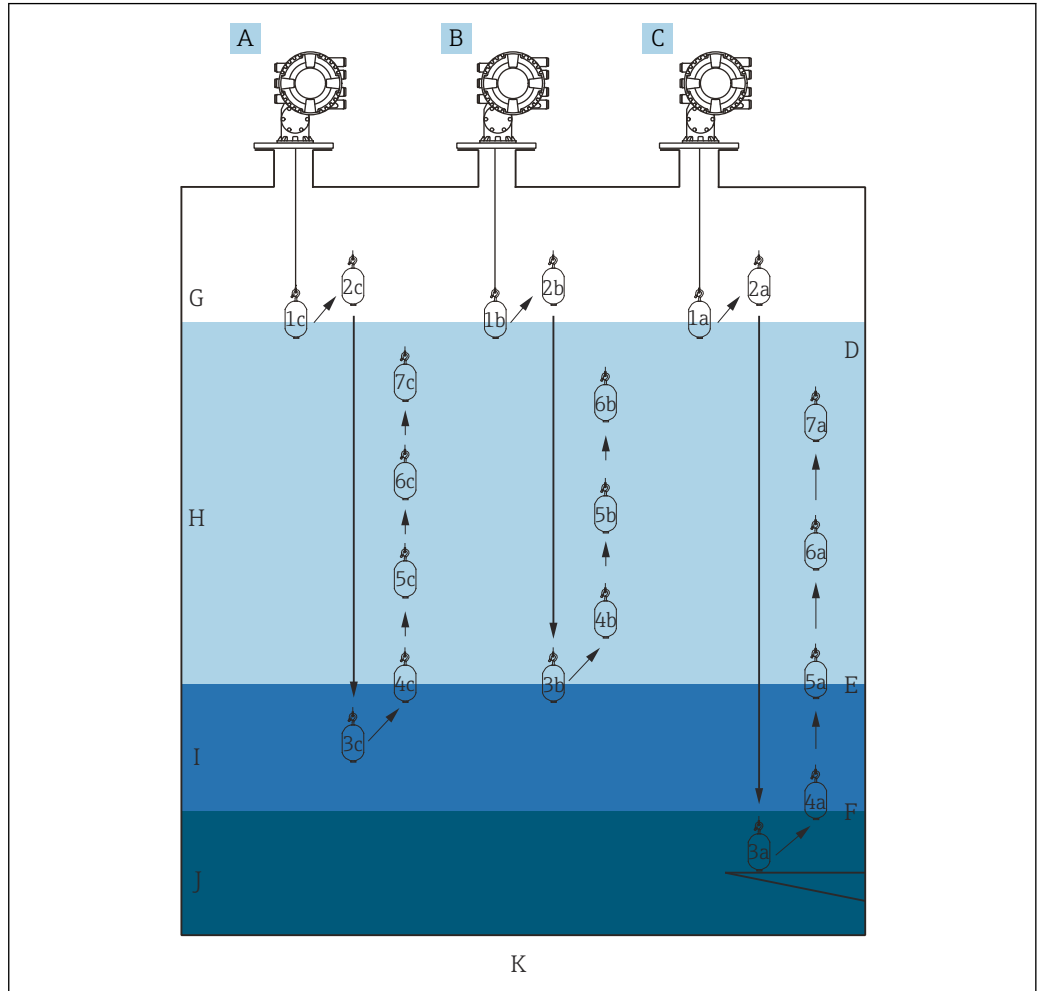
図 49 プロファイル密度の概要 (1a、2a、3a... はディスプレイサの移動順序を示します)
