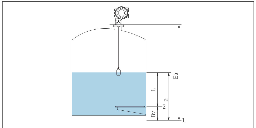
46 非開放タンク (NMS83)
