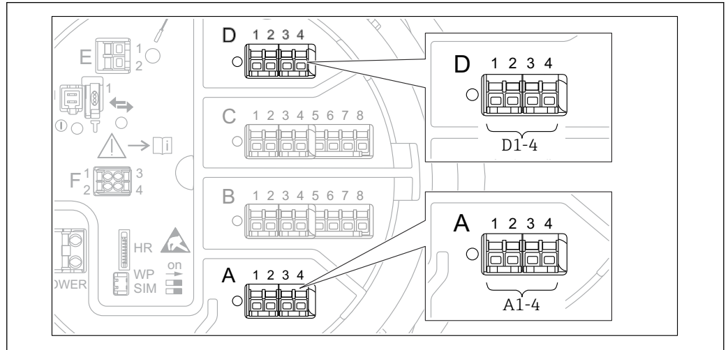
図 68 Modbus モジュールの使用可能な端子 (例)。機器バージョンに応じて、Modbus モジュールがスロット B または C に対応する場合があります → 38。
