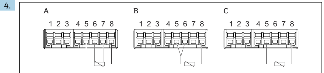
図 59 測温抵抗体の接続タイプ
