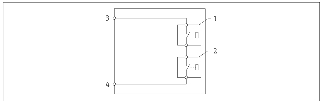
図 88 デジタル出力の 2 つのリレー
