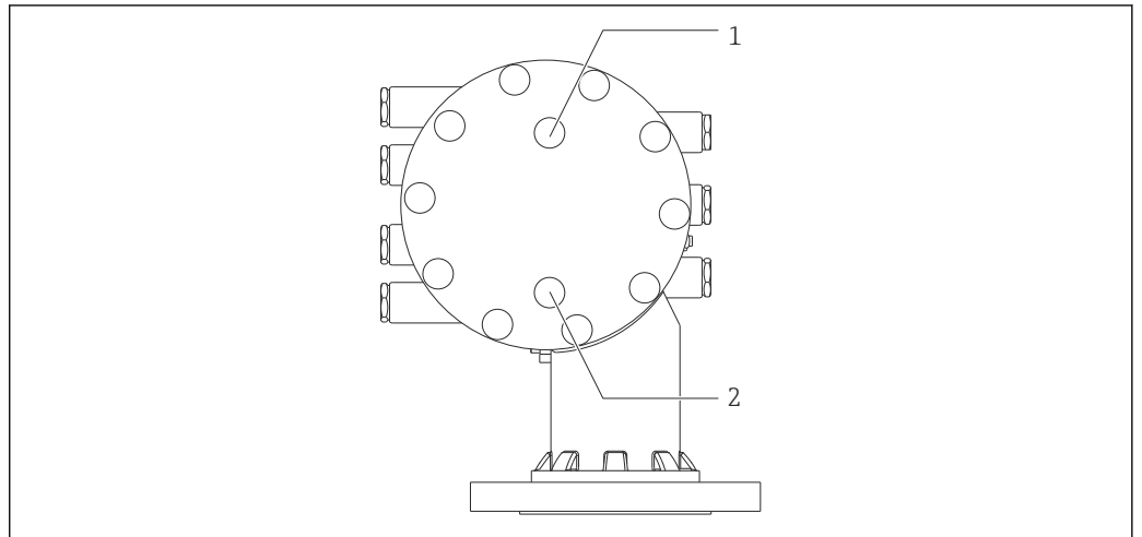
図 79 洗浄ノズルおよびガスパージノズル用の穴
