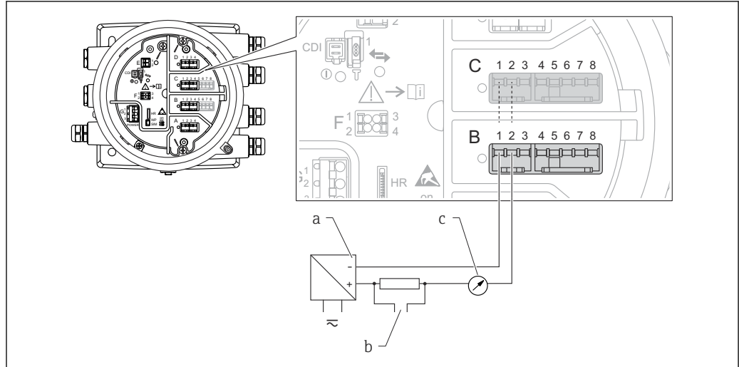
図 16 出力モードのアナログ I/O モジュールのパッシブ使用
