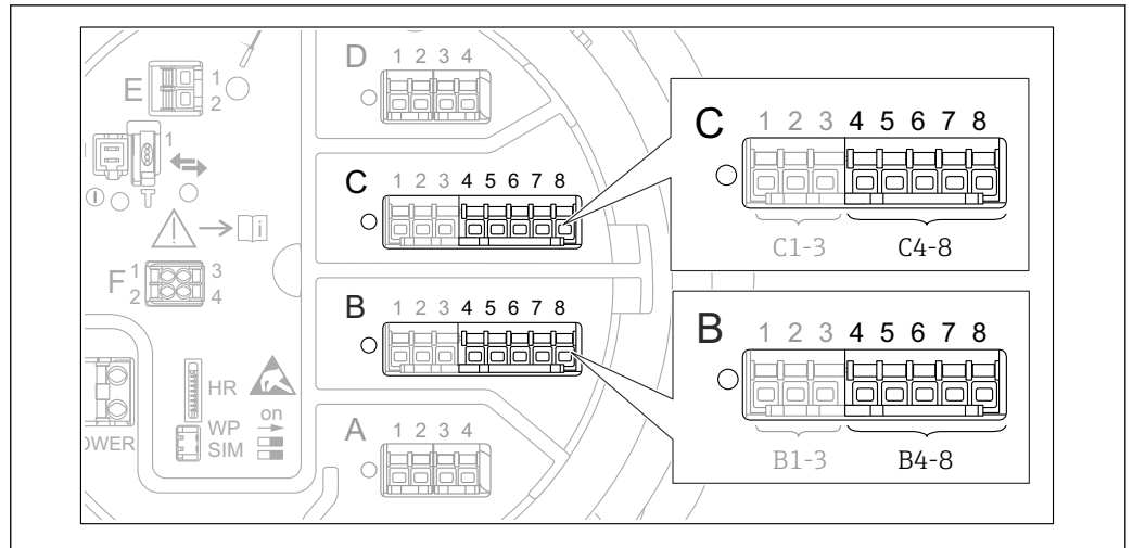
図 58 アナログ I/O モジュールの使用可能な端子。測温抵抗体を接続できます。機器のオーダーコードは、実際に存在するモジュールを示します → 図 38。
