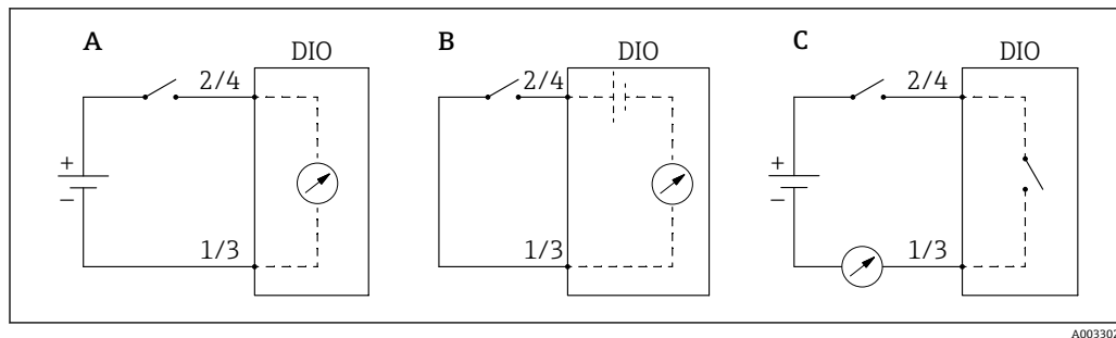
図 87 デジタル I/O モジュールの操作モード
