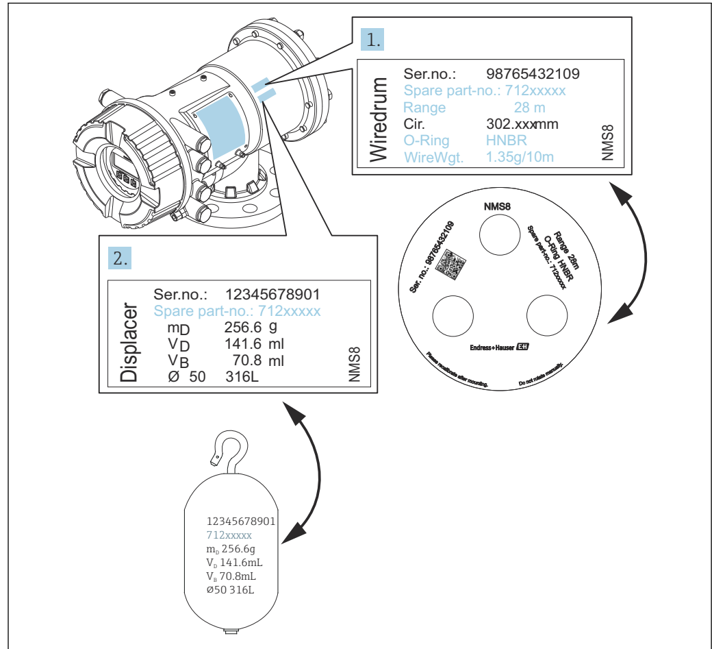
11 ディスプレーサ・ワイヤドラムの確認
