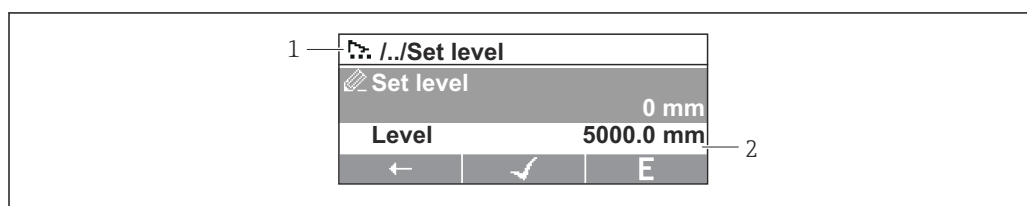
図 26 表示モジュールのウィザード画面
