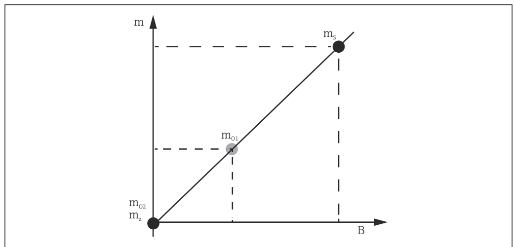
図 38 センサ校正のコンセプト
