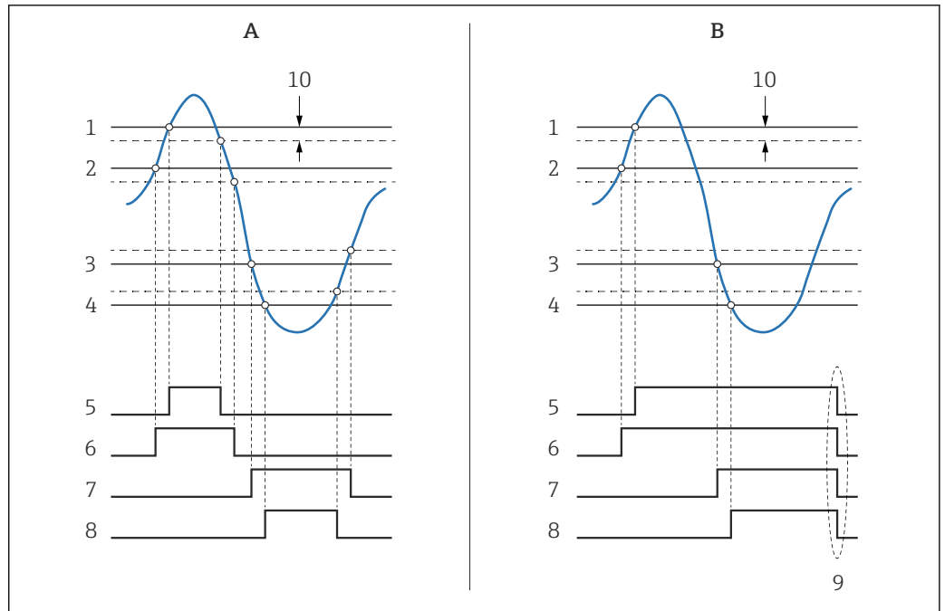
図 95 リミット評価の原理
