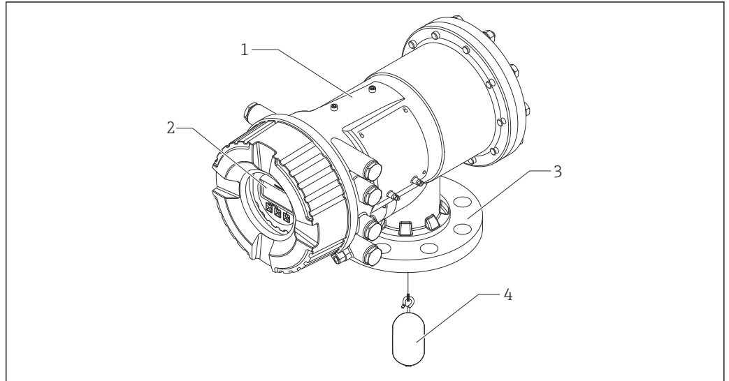
図 1 プロサーボ NMS83 の構成
