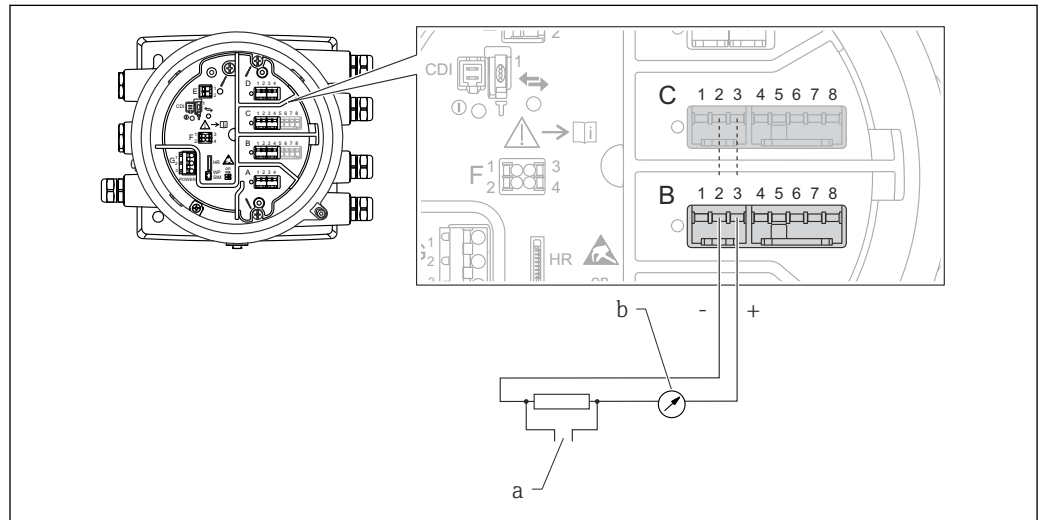
図 19 出力モードのアナログ I/O モジュールのアクティブ使用
