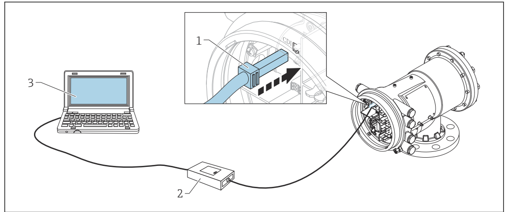
図 33 サービスインタフェース経由の操作
