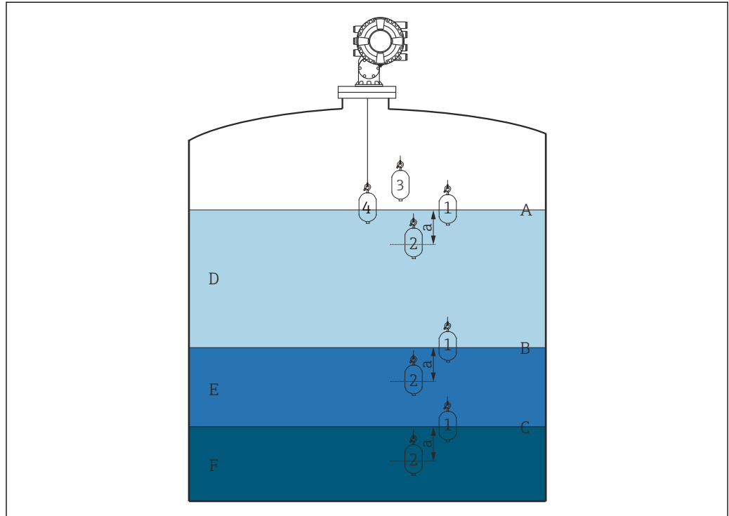
図 48 スポット密度 (数字はディスプレイサの移動順序を示します)
