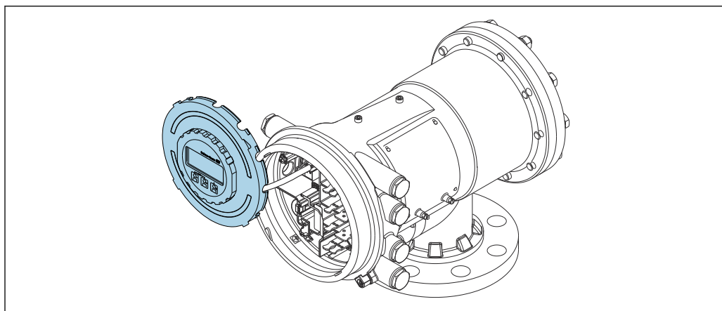
図 31 NMS83 : 端子室の縁に差し込まれた表示モジュール
