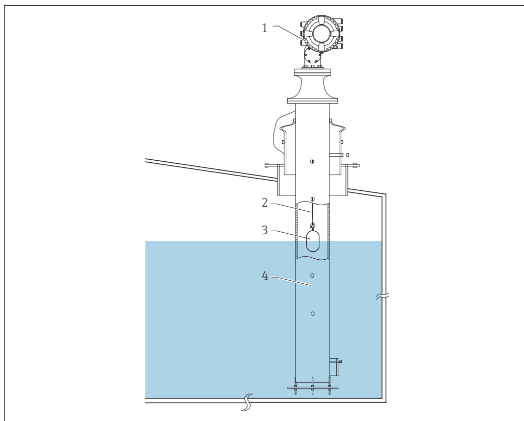
図 4 一般的なタンクの設置 1
