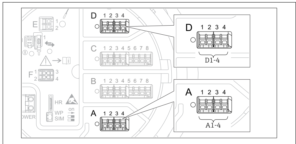
図 70 WM550 モジュールの使用可能な端子 (例)。機器バージョンに応じて、WM550 モジュールがスロット B または C に対応する場合があります → 38。
