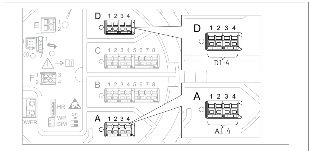
図 69 V1 モジュールの使用可能な端子 (例)。機器バージョンに応じて、V1 モジュールがスロット B または C に対応する場合があります → 38。
