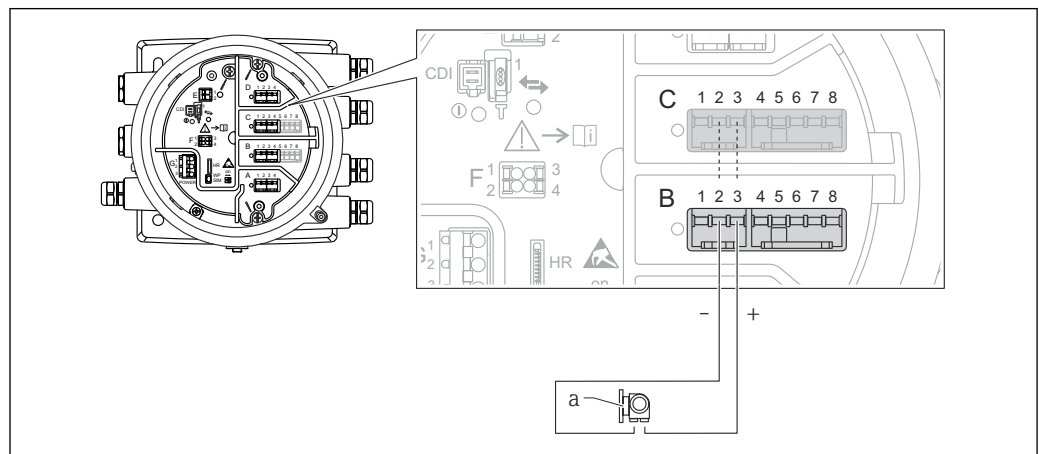
図 20 入力モードのアナログ I/O モジュールのアクティブ使用
