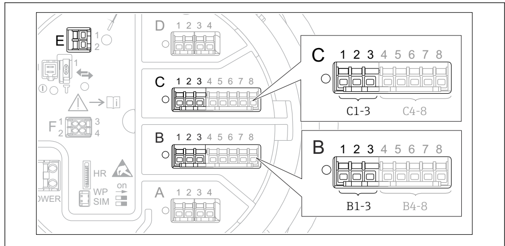
図 53 HART ループに使用可能な端子
