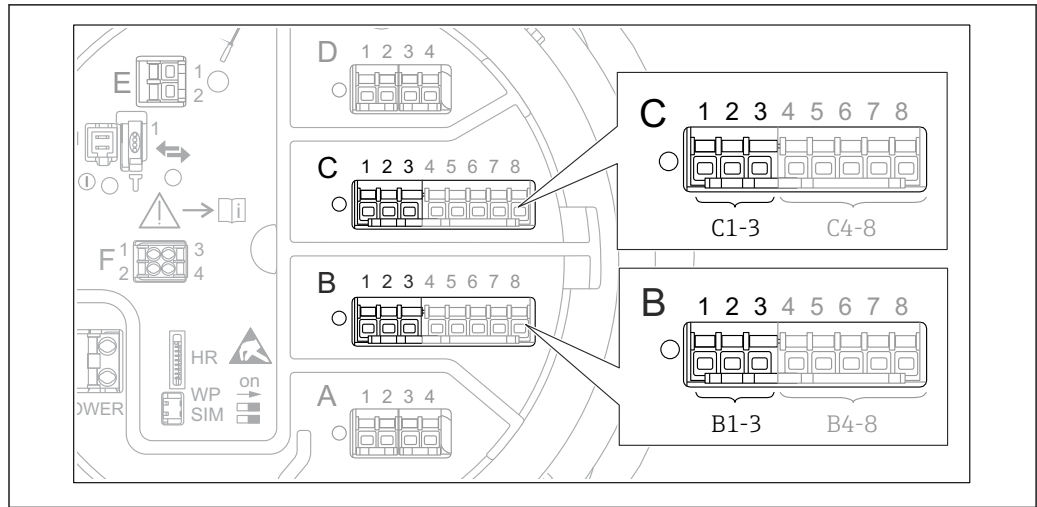
図 56 アナログ I/O モジュールの使用可能な端子。4~20 mA 入力として使用できます。機器のオーダーコードは、実際に存在するモジュールを示します → 図 38。
