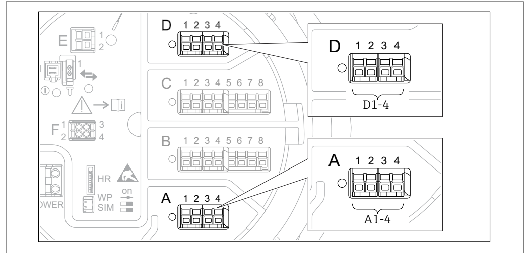
89 機器バージョンに応じて、「Modbus」、「V1」、「WM550」モジュール（例）がスロット B または C に対応する場合があります。
