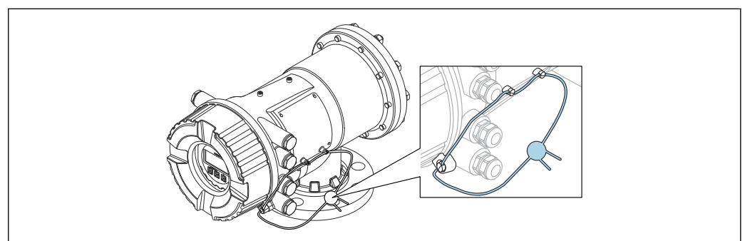
☒ 29 端子部（上部）のカバーのシーリング
