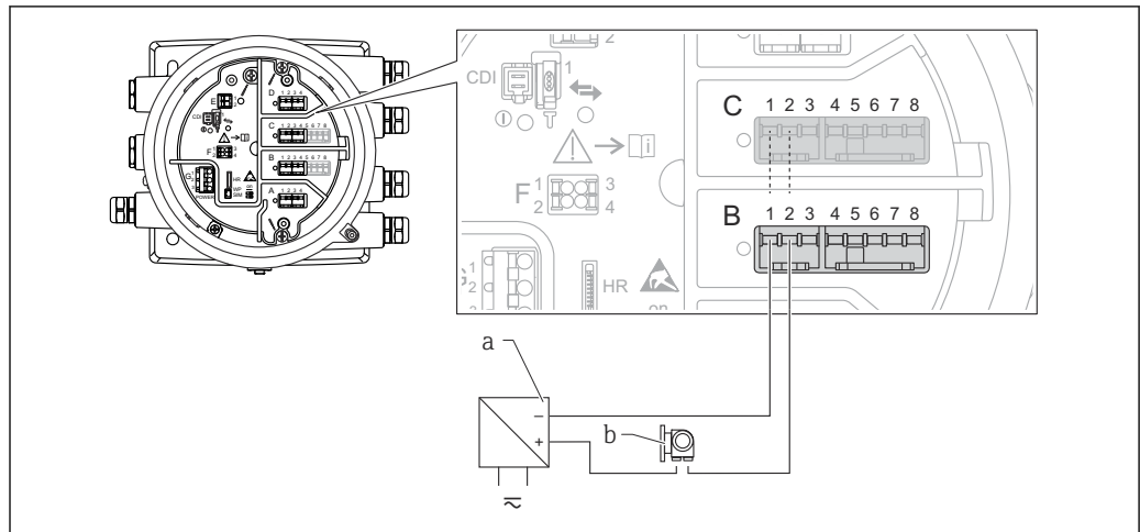
図 17 入力モードのアナログ I/O モジュールのパッシブ使用
