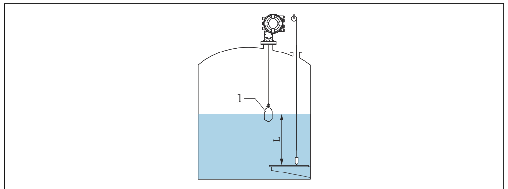
図 44 開放タンク（液体あり）のレベルの設定
