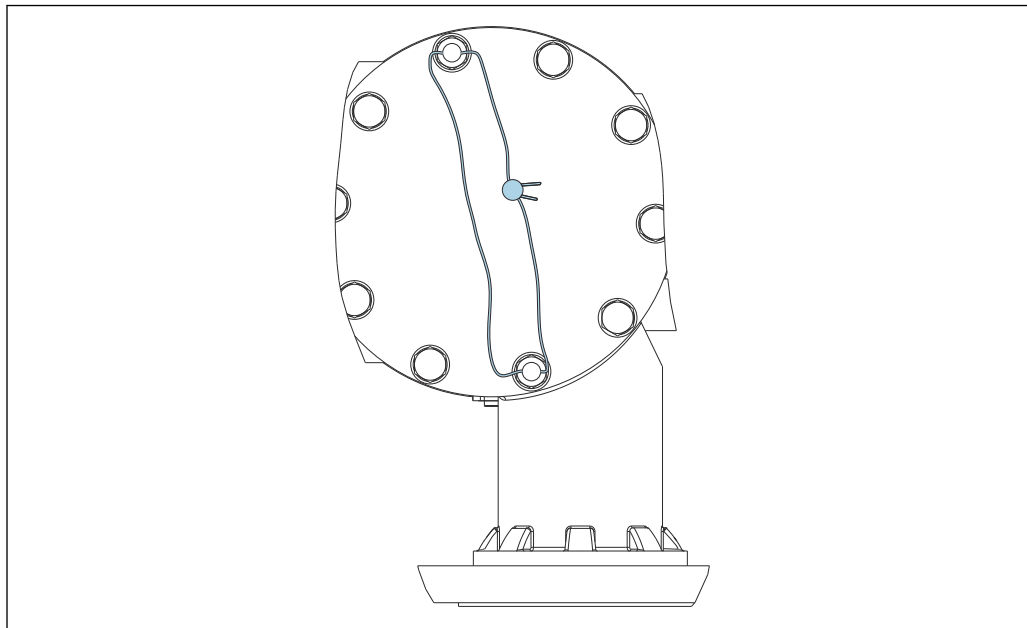
図 30 後部カバーのシーリング (例 : NMS81/NMS83)
