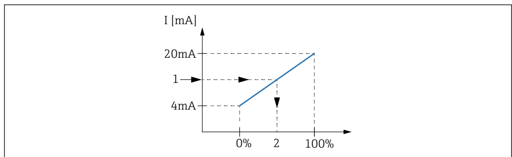
図 57 プロセス変数への 4~20 mA 入力のスケーリング
