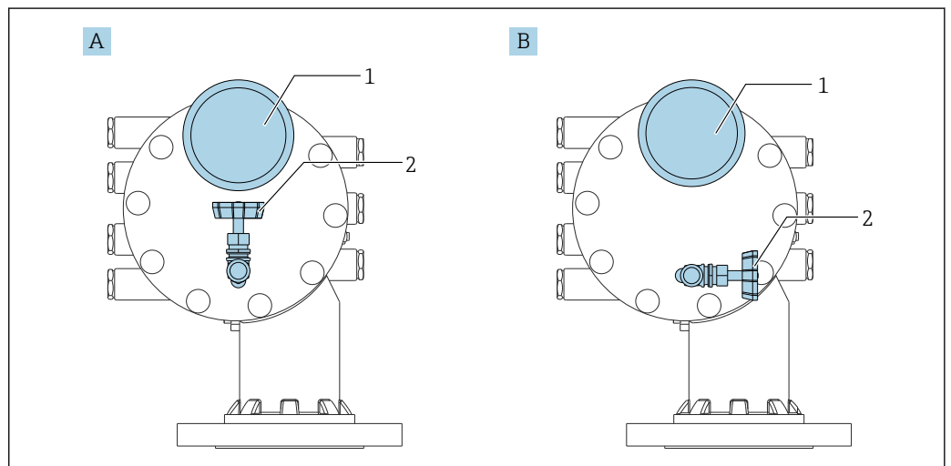
図 76 リリーフバルブおよび圧力計の取付位置
