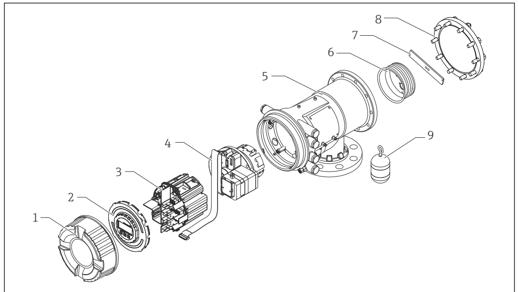
図 2 プロサーボ NMS83 の構成
