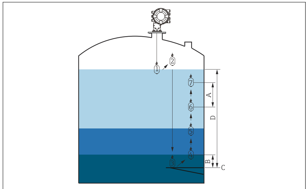
図 50 タンクプロフィールの移動（数字はディスプレイ上の移動順序を示します）
