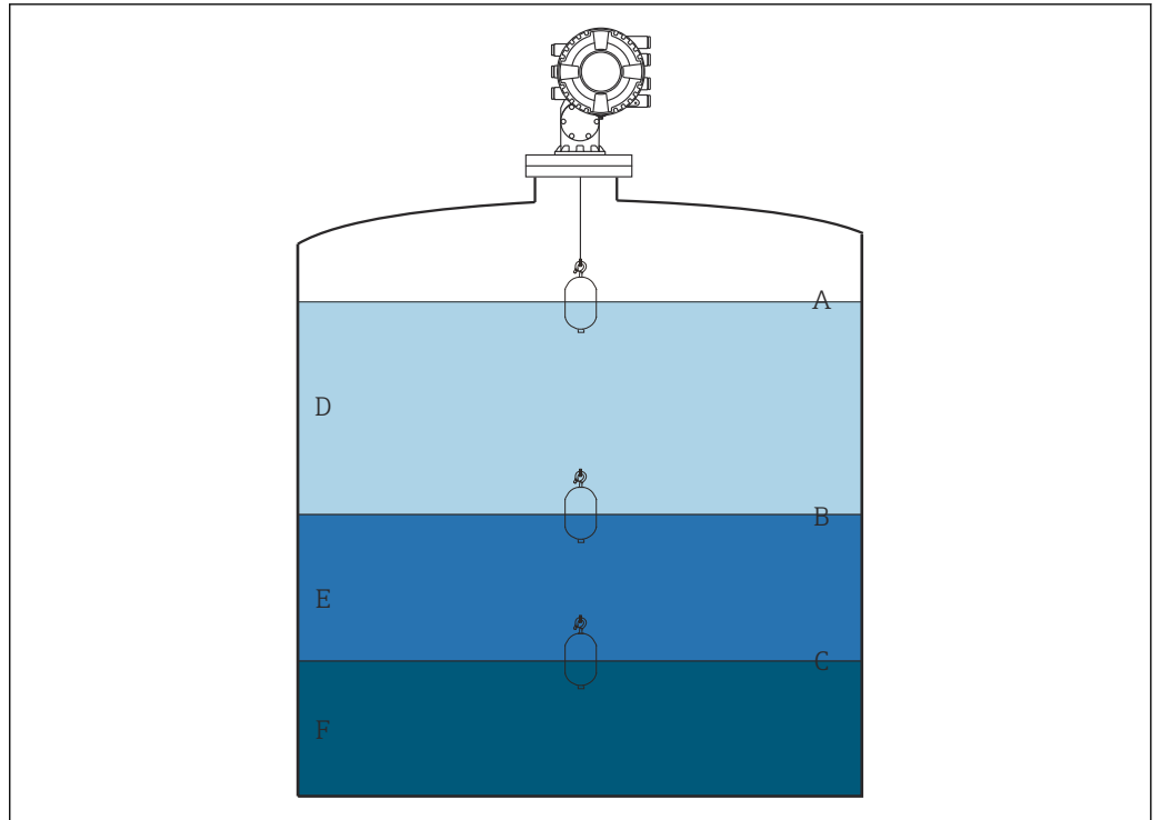
図 42 タンクの設定
