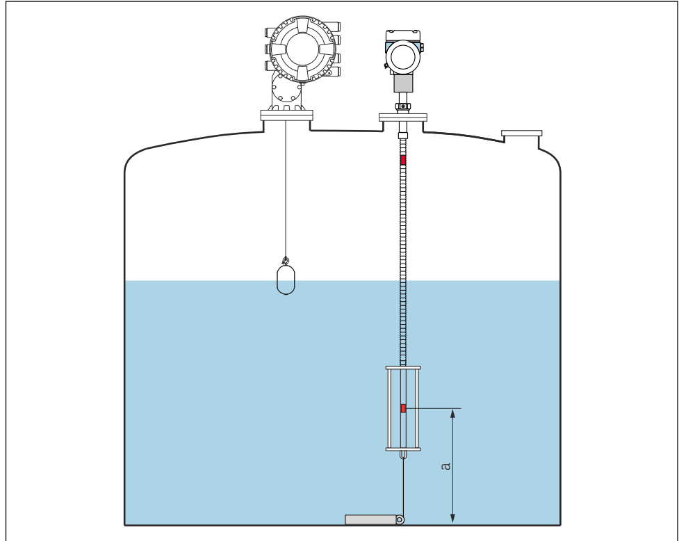
図 54 Prothermo NMT53x : ボトム温度素子の位置
