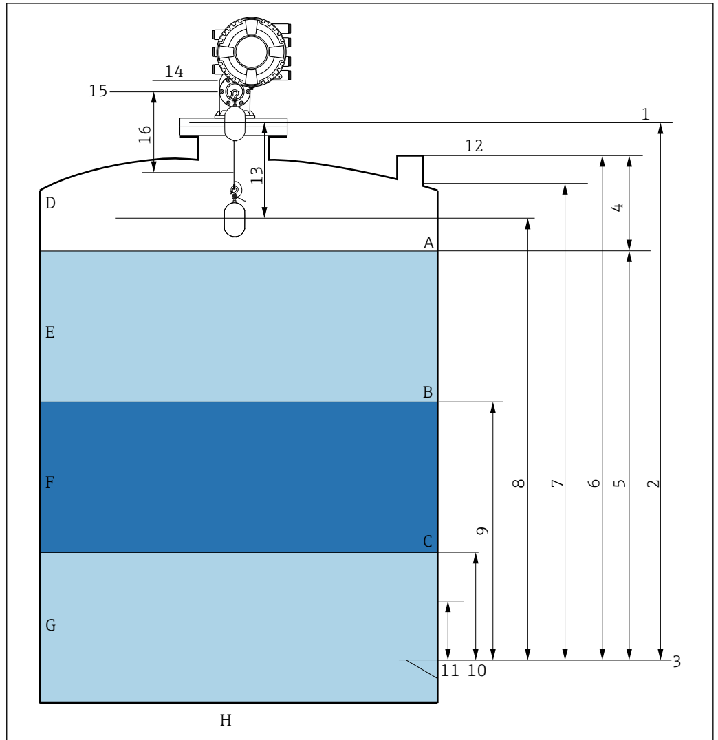
図 35 NMS8x の設置に関連する用語 (例 : NMS81)
