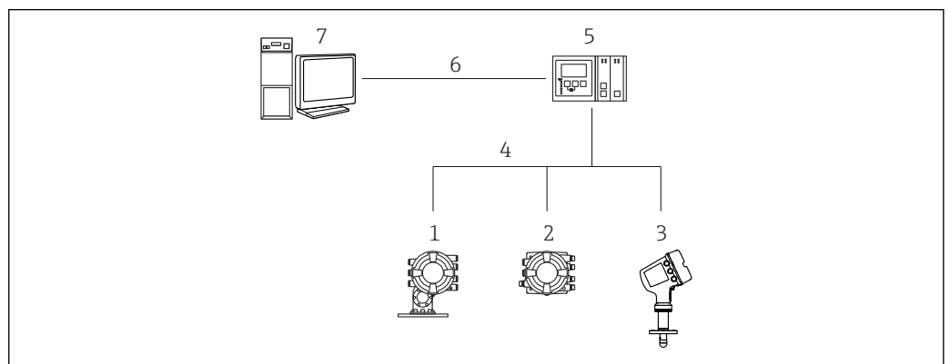
図 34 Tankvision Tank Scanner NXA820 経由でタンクゲージ機器を FieldCare に接続
