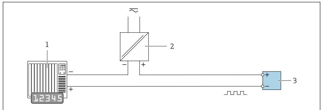
☑ 11 接线实例：脉冲/频率输出（无源信号）
