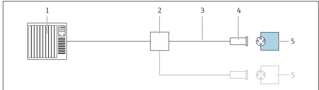
图 8 接线实例: EtherNet/IP
