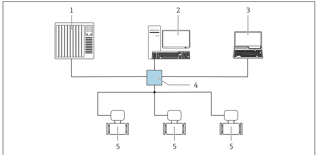
图 20 通过 EtherNet/IP 网络进行远程操作：星形拓扑结构
