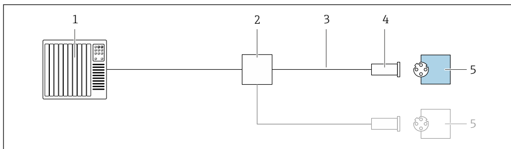
8 Exemplo de conexão para EtherNet/IP
