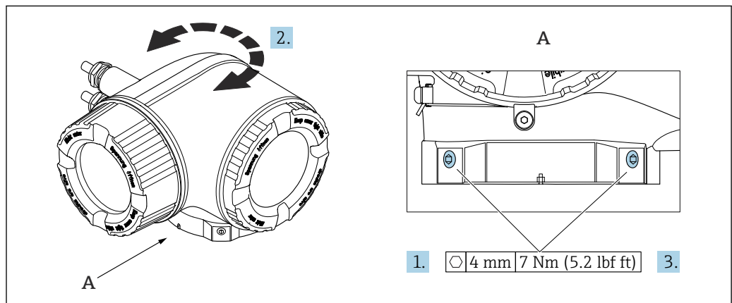
图 6 防爆型外壳
