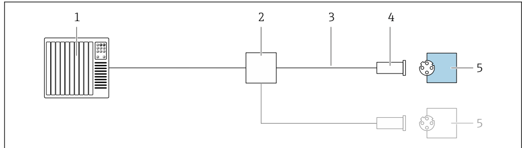
图 8 接线实例: PROFINET
