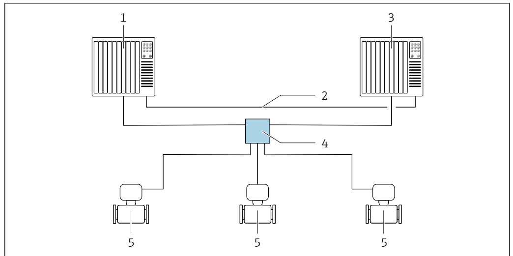
图 25 S2 系统冗余布局实例：星形拓扑结构
