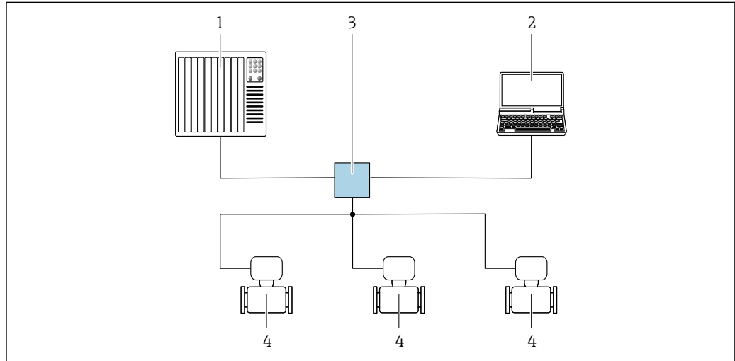
图 21 通过 PROFINET 网络进行远程操作：星形拓扑结构
