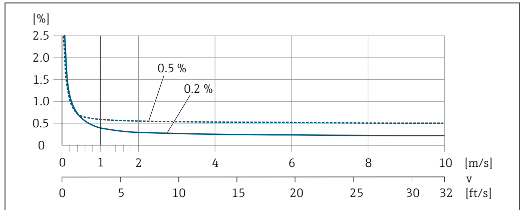
图 32 最大测量误差 (% o.r.)
