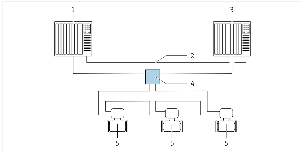
图 24 S2 系统冗余布局实例：环形拓扑结构
