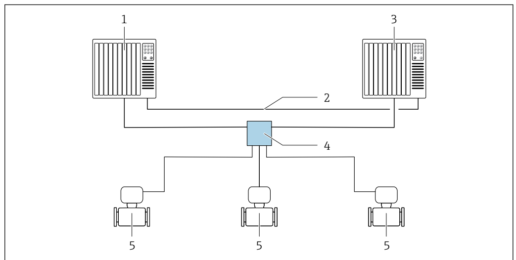
▣ 25 Exemplo do layout de um sistema redundante (S2): topologia estrela
