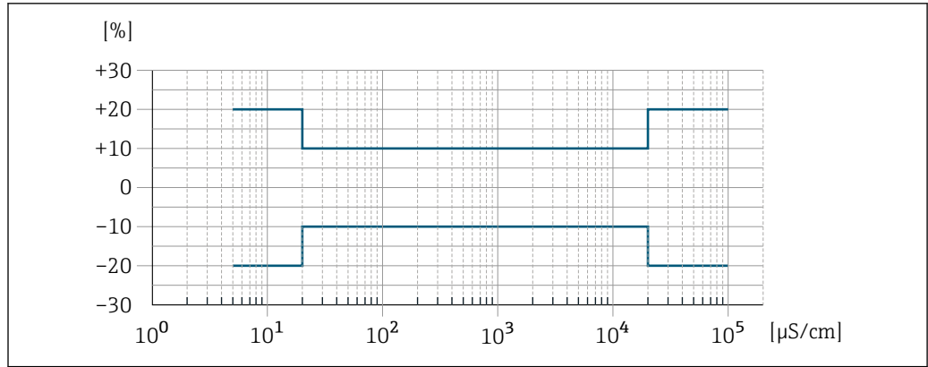
33 Erro de medição (padrão)
