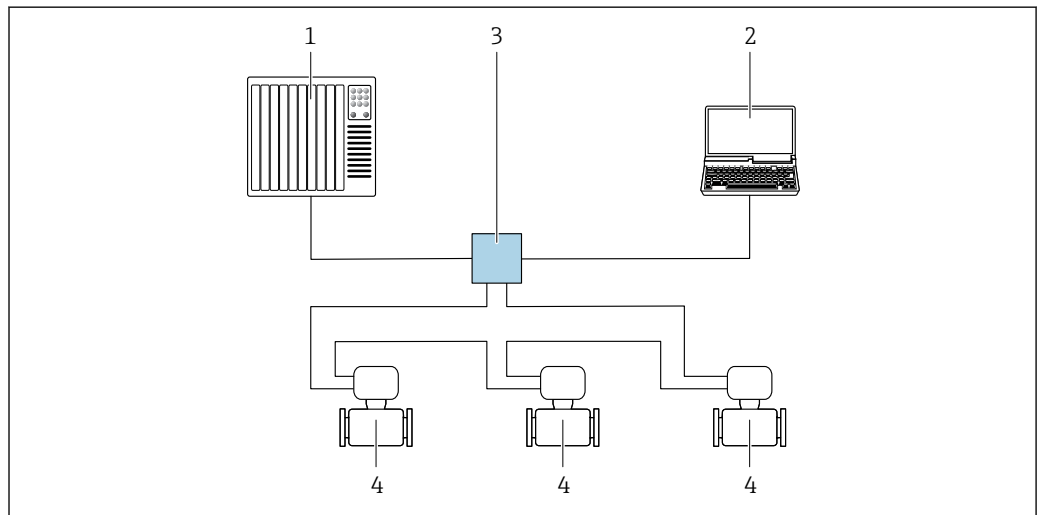
22 Opções para operação remota através da rede PROFIBUS: topologia em anel
