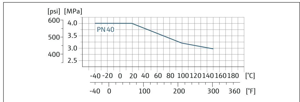
図 28 プロセス接続材質：ステンレス 1.4404 (SUS F316L 相当)
