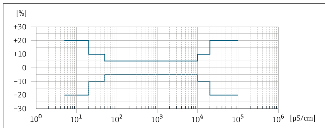
図 25 測定誤差（オプション：「校正済導電率測定」のオーダーコード、オプション CW）
