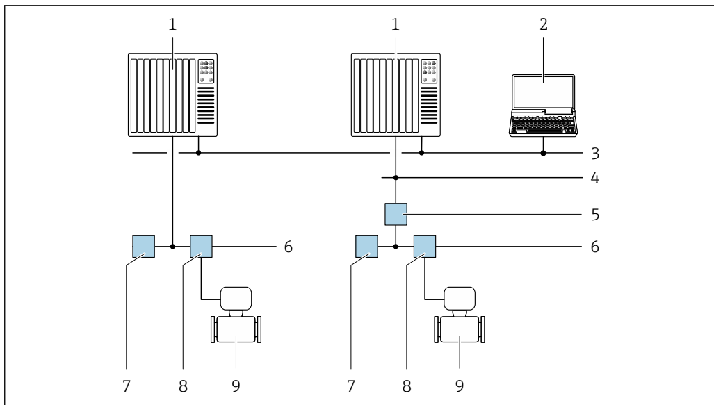
図 63 FOUNDATION フィールドバスネットワークを介したリモート操作のオプション
