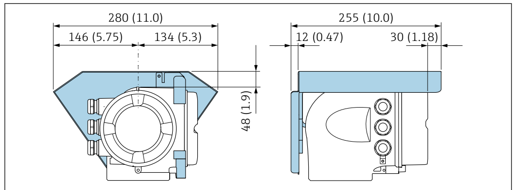
26 単位 mm (in)
