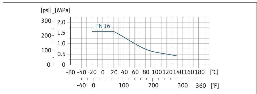
図 29 プロセス接続材質：PVDF
