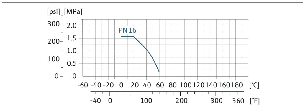
30 プロセス接続材質：PVC-U
