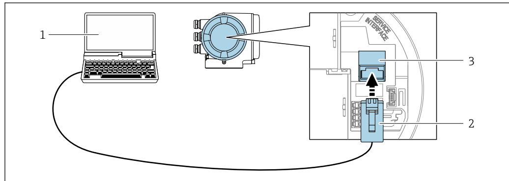
図 72 サービスインタフェース (CDI-RJ45) 経由の接続
