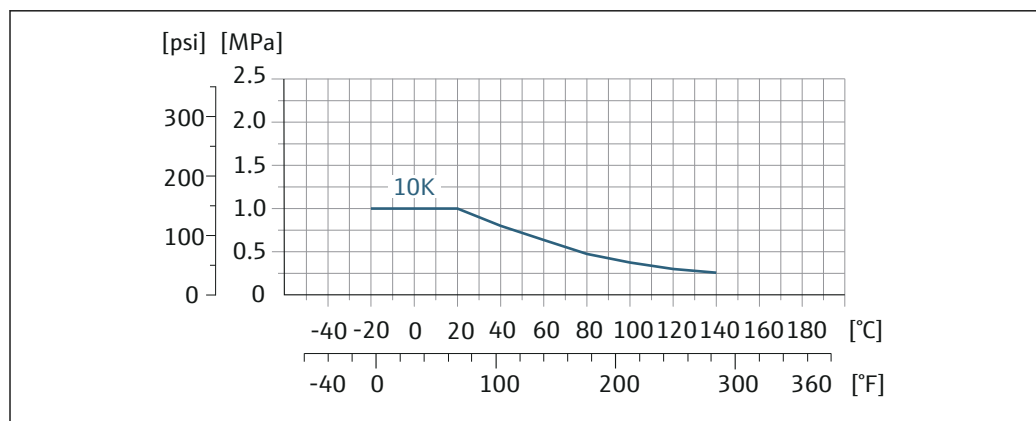
図 34 プロセス接続材質 : PVDF
