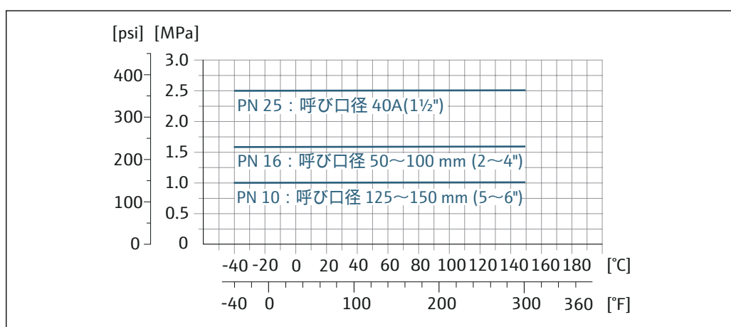
図 41 プロセス接続材質 : ステンレス 1.4404 (SUS F316L 相当)
