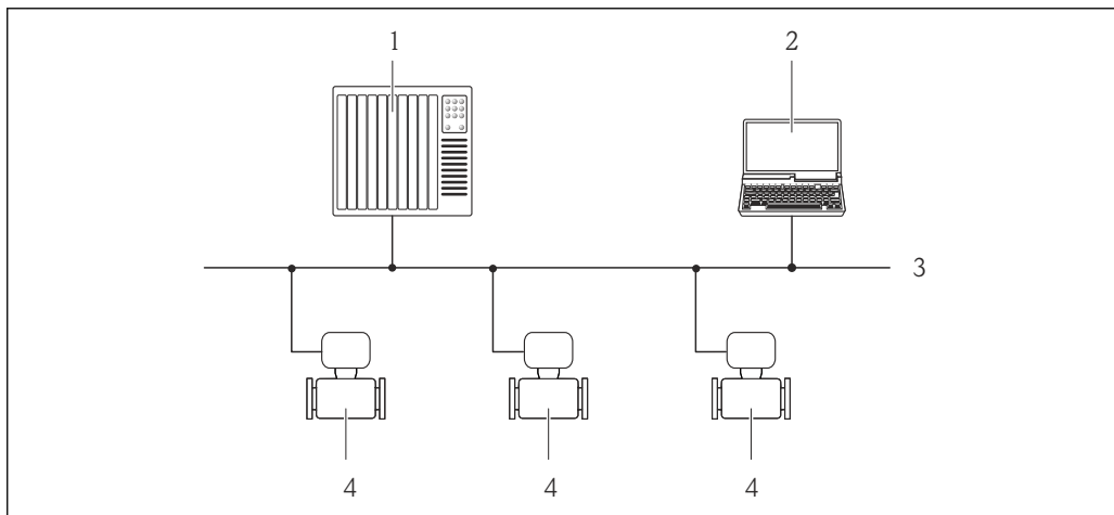
図 64 PROFIBUS DP ネットワークを介したリモート操作のオプション
