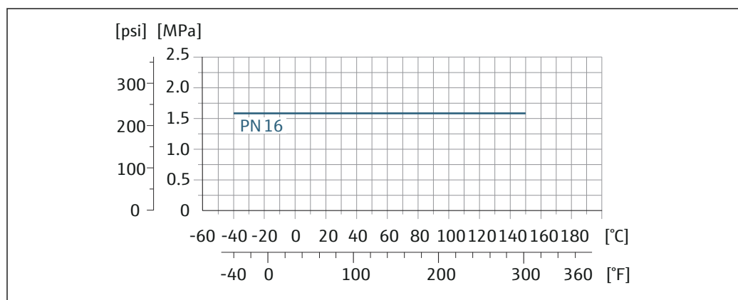
図 35 プロセス接続材質 : ステンレス 1.4404 (SUS F316L 相当)
