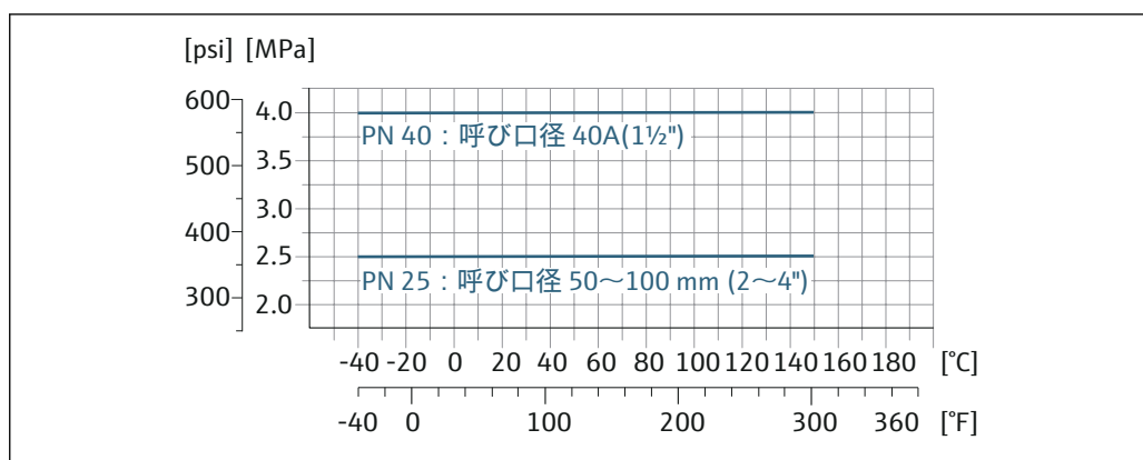
図 40 プロセス接続材質 : ステンレス 1.4404 (SUS F316L 相当)
