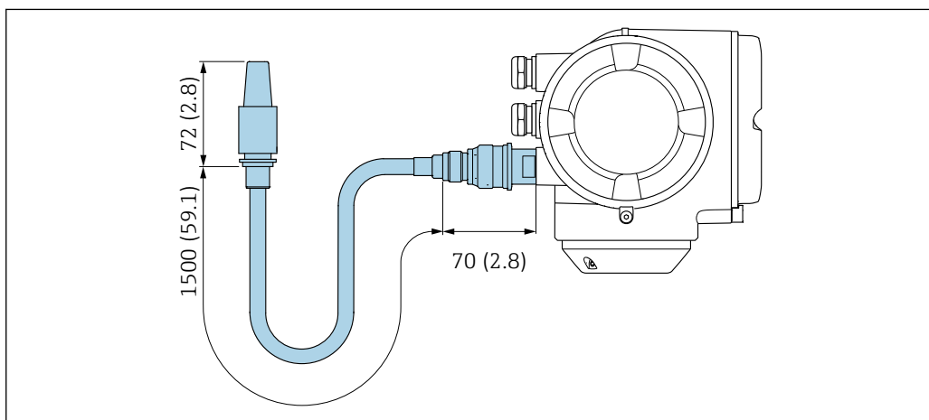
図 50 単位 mm (in)
