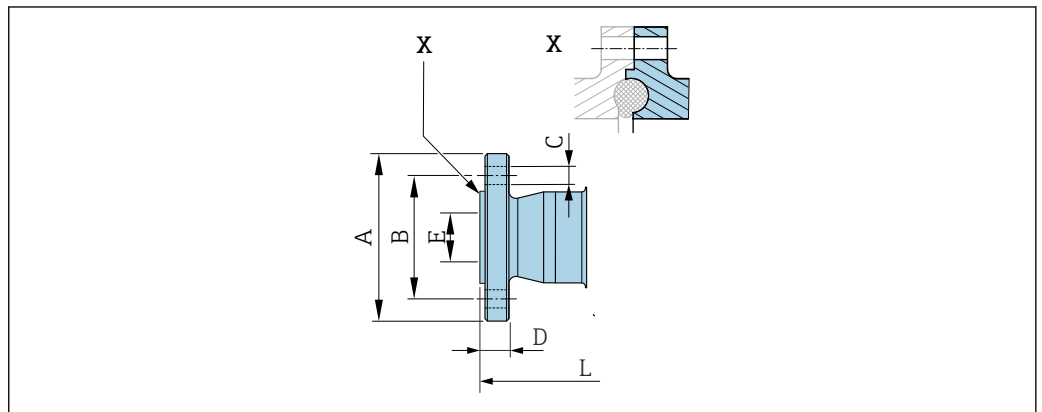
図 45 Xの詳細：非対称型プロセス接続；青色部分が供給されます。
