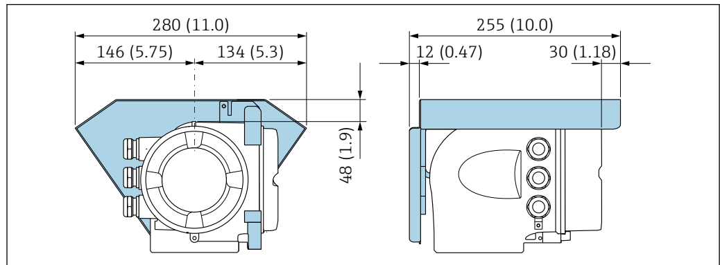
図 47 単位 mm (in)
