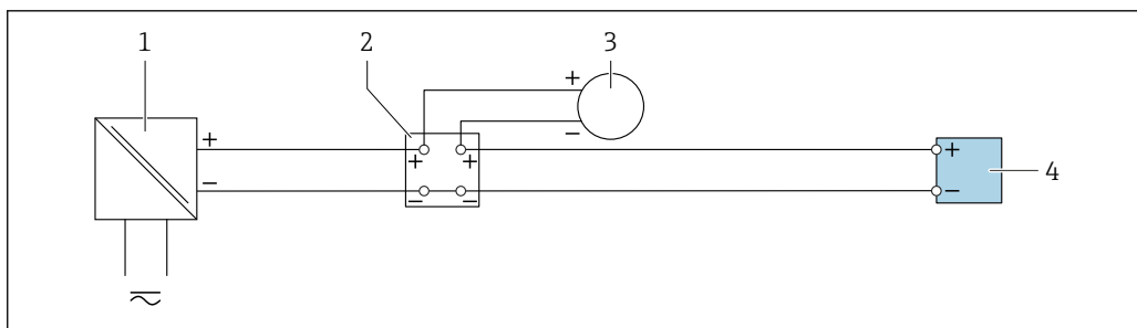
☐ 21 4~20 mA 電流入力の接続例
