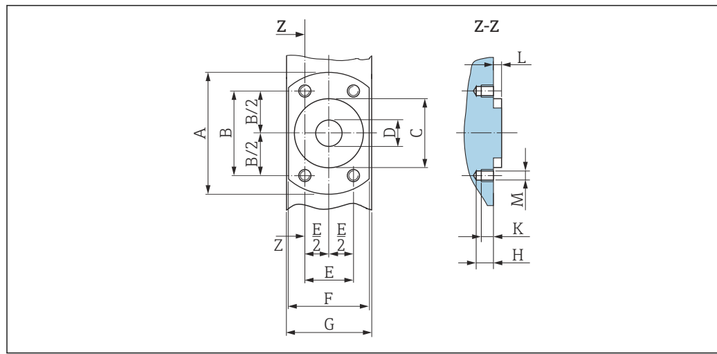
図 43 プロセス接続なしの正面図
