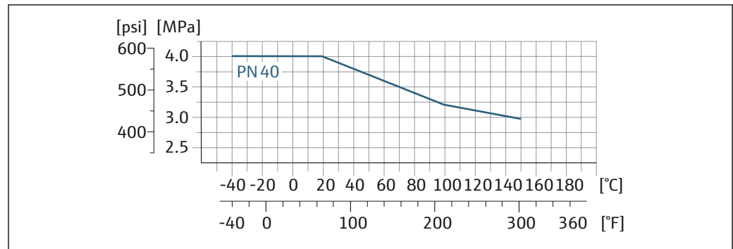
図 27 プロセス接続材質：ステンレス 1.4404 (SUS F316L 相当)
