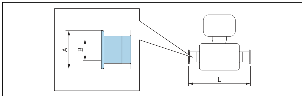
図 57 ASME BPE 準拠の配管接続に最適なサニタリクランプアダプタ接続 (レデュース)
