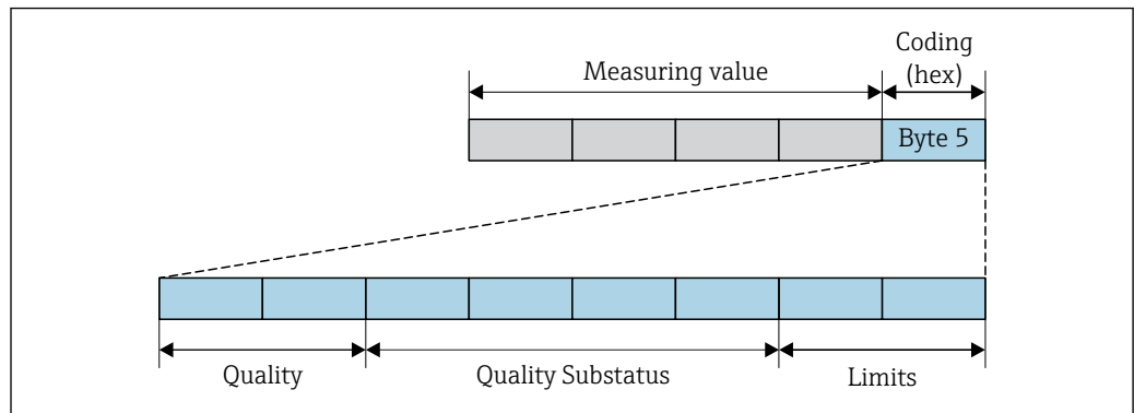
27 Struttura del byte di codifica
