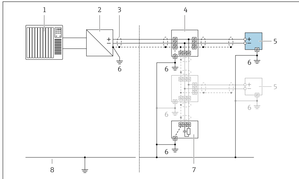
7 Esempio di collegamento per PROFIBUS PA
