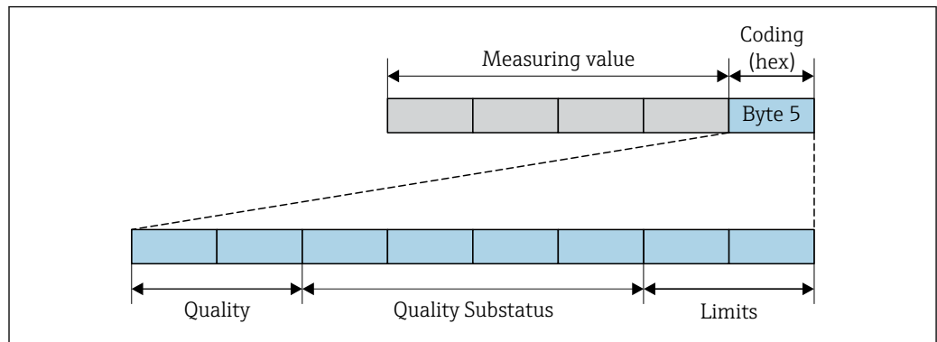
Fig. 27 Estrutura do byte de codificação
