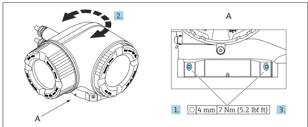
图 6 防爆型外壳
