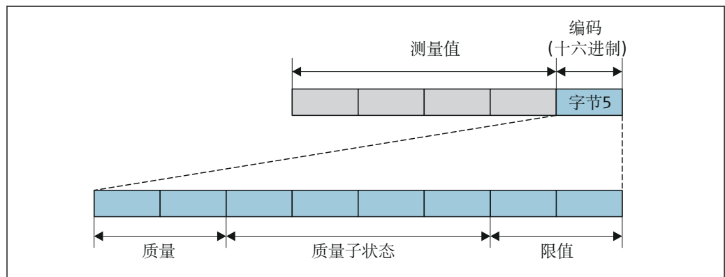
图 27 编码字节结构
