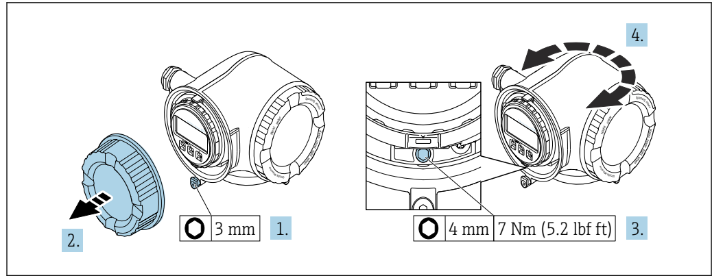
图 5 非防爆型外壳
