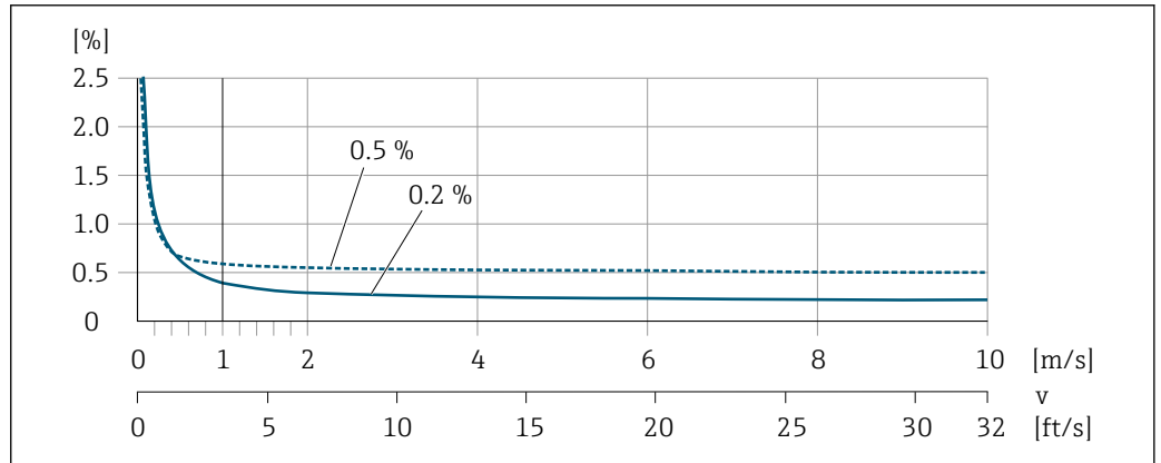
图 41 最大测量误差 (% o.r.)
