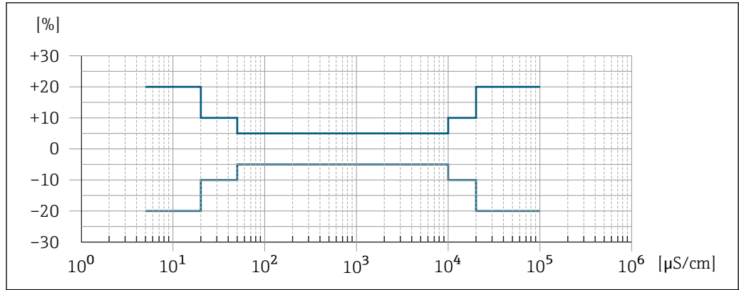
图 47 测量误差 (可选: 订购选项“电导率测量标定”, 选型代号 CW)
