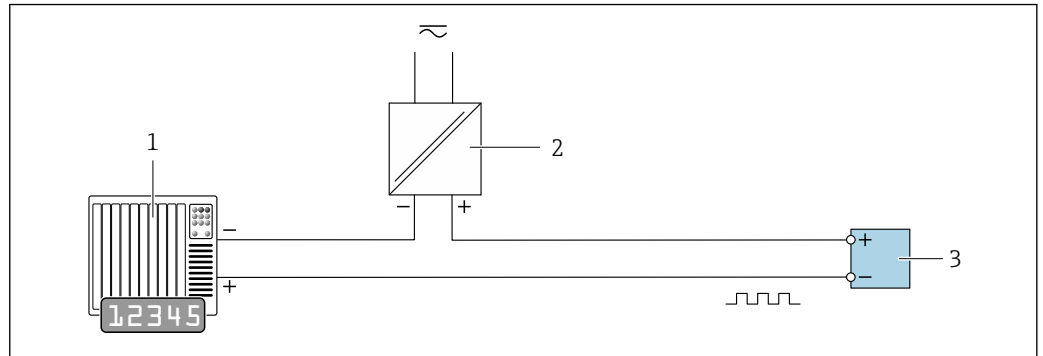
图 23 接线示例：脉冲/频率输出（无源信号）
