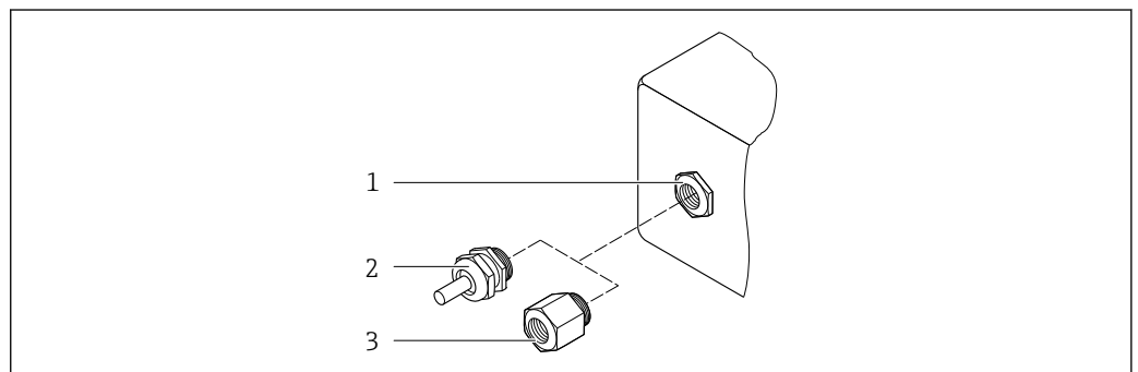
图 50 允许的电缆入口/缆塞
