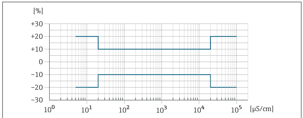
46 测量误差 (标准)
