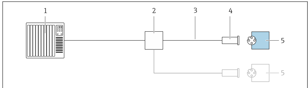
图 18 接线实例: EtherNet/IP
