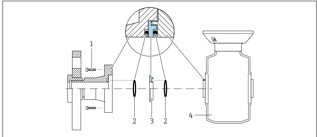
图 9 安装接地环
