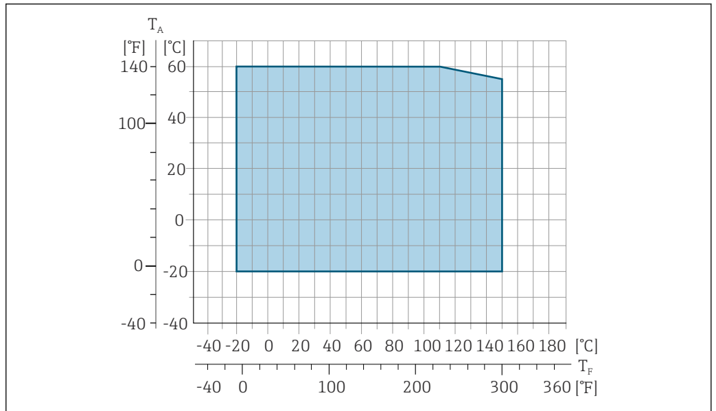
图 44 Promag 500 (模拟)
