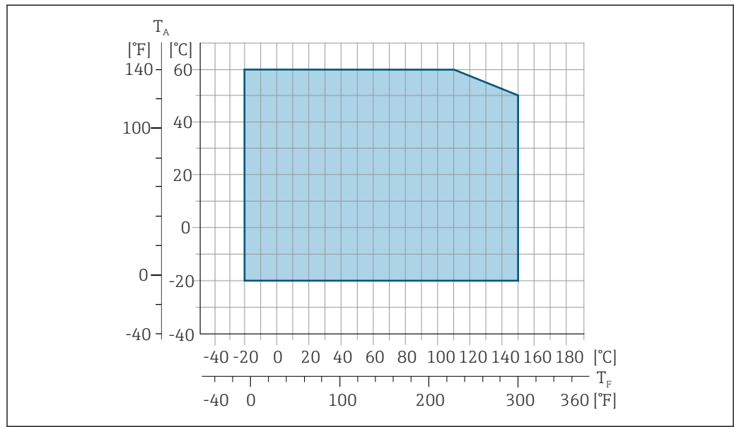
图 43 Promag 500 (数字)
