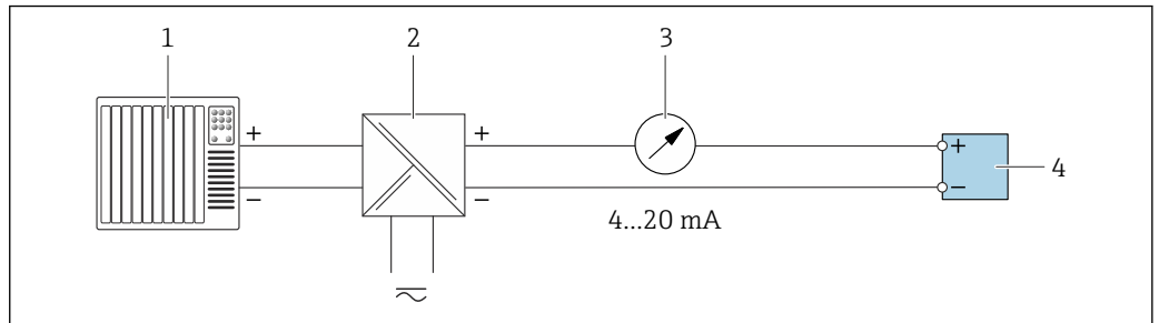
20 接线实例: 4...20 mA 电流输出 (无源信号)
