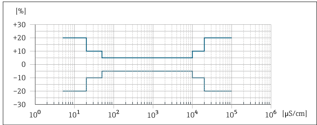
图 42 测量误差 (可选: 订购选项“电导率测量标定”, 选型代号 CW)
