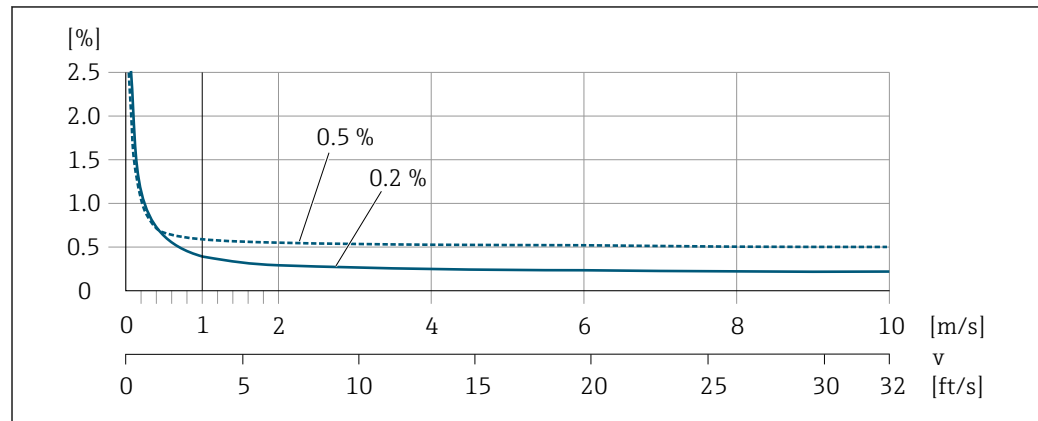
42 Errore di misura massimo in % v.i.
