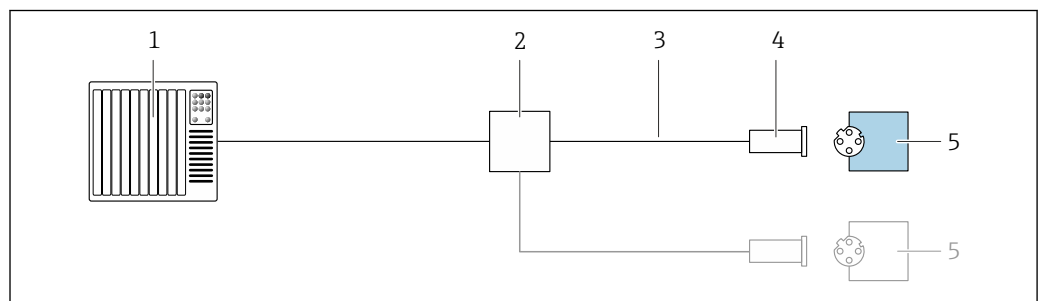
17 Esempio di collegamento per PROFINET
