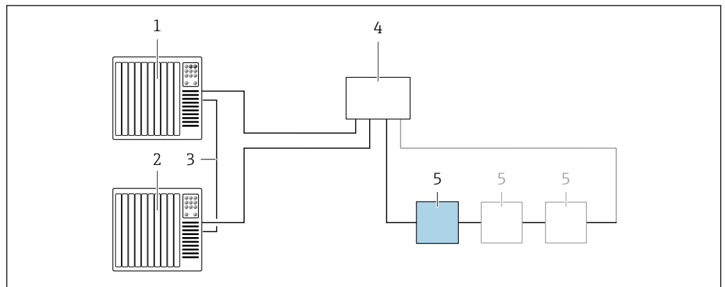
18 Esempio di connessione per ridondanza di sistema S2
