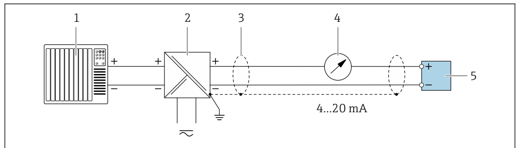
20 Ejemplo de conexión de una salida de corriente de 4 a 20 mA HART (pasiva)
