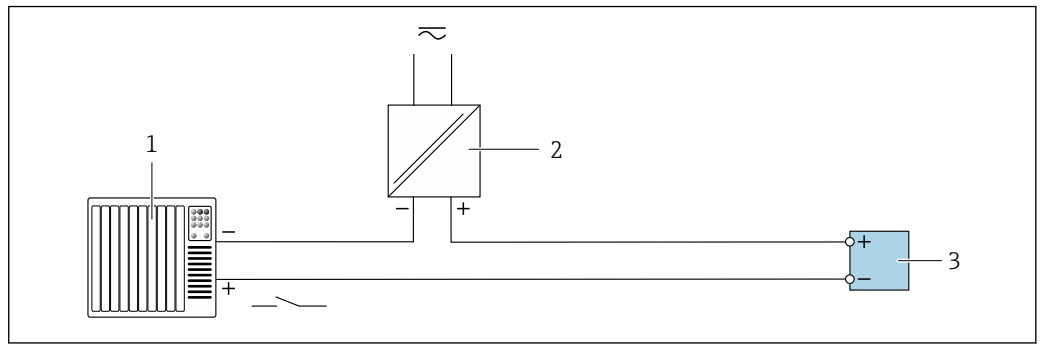
30 Ejemplo de conexión de una entrada de estado
