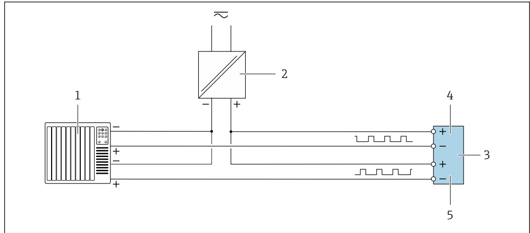
27 Ejemplo de conexión de una doble salida de pulsos (pasiva)
