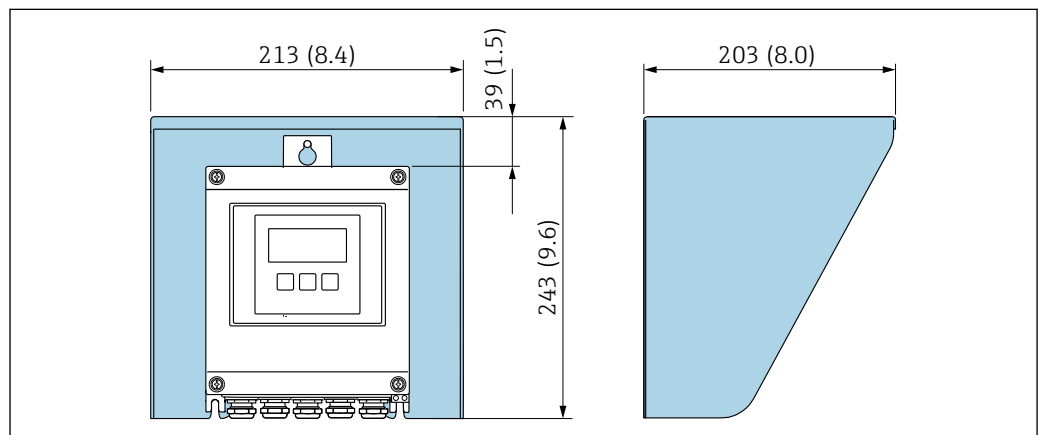
图 10 Proline 500（数字）变送器的防护罩的外形尺寸图；单位：mm (in)
