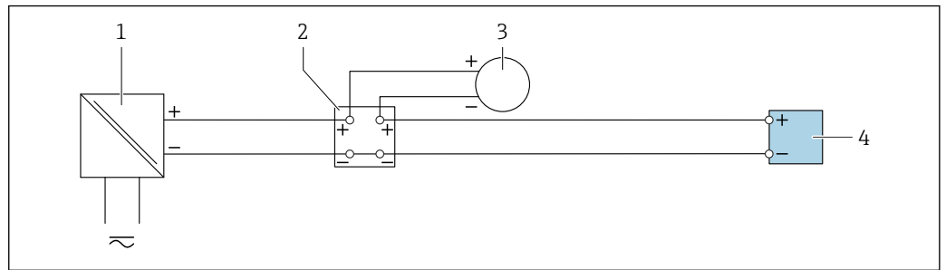
图 29 接线实例：4...20 mA 电流输入
