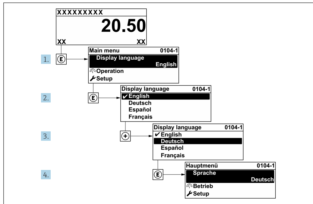
图 39 现场显示示意图
