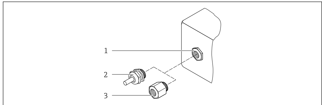
图 48 允许的电缆入口/缆塞
