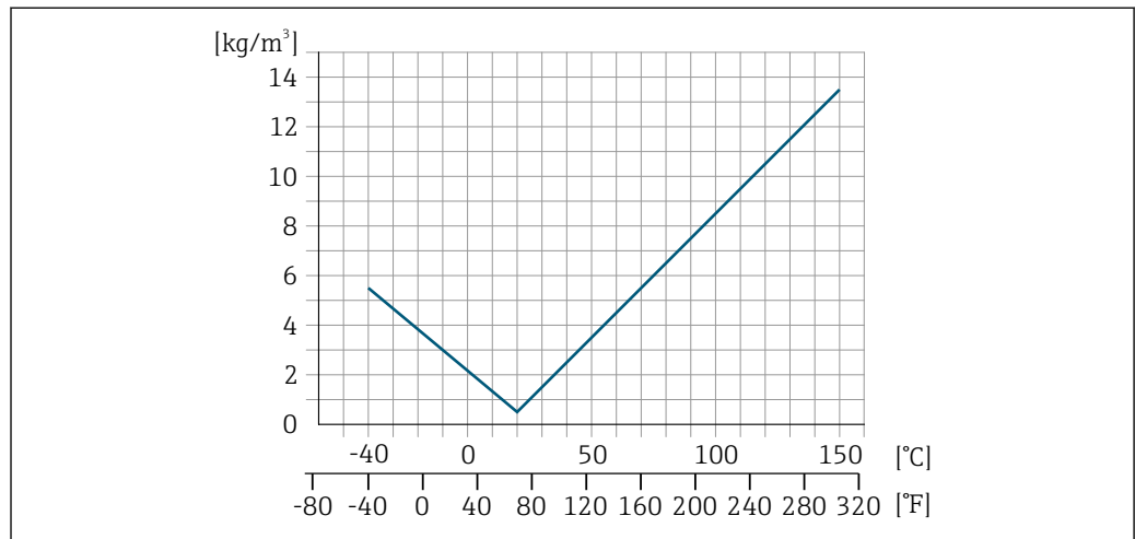
图 47 现场密度校正，例如在+20 °C (+68 °F)时
