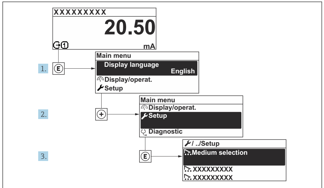
图 40 “设置”菜单菜单路径（现场显示单元）
