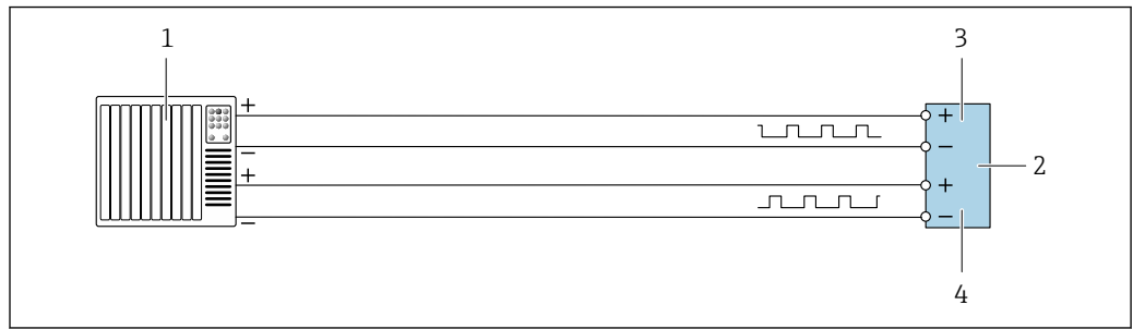
图 26 接线实例：双脉冲输出（有源信号）
