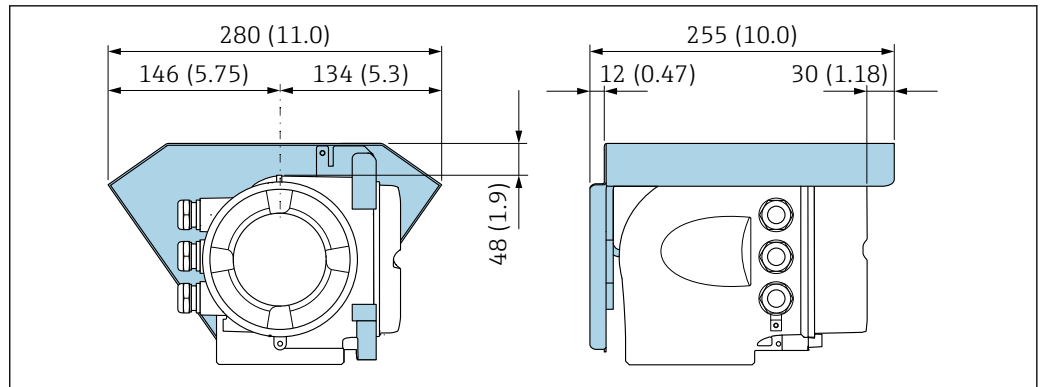
图 11 Proline 500 变送器的防护罩的外形尺寸图；单位：mm (in)
