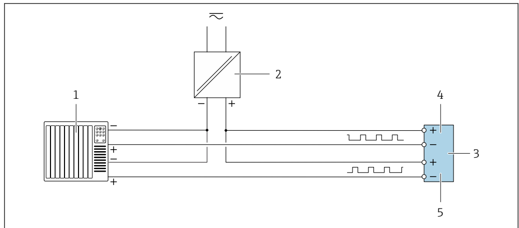
图 27 接线实例：双脉冲输出（无源信号）
