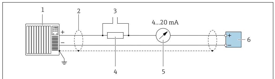
图 19 4...20 mA HART 电流输出 (有源) 的接线图
