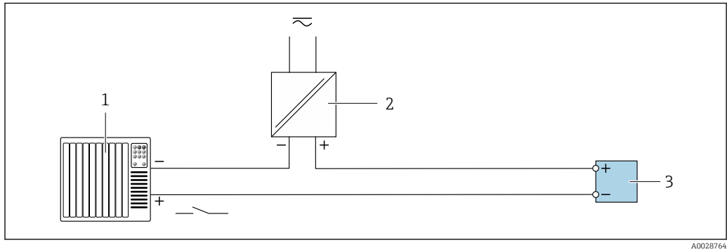
30 Exemplo de conexão para entrada de status
