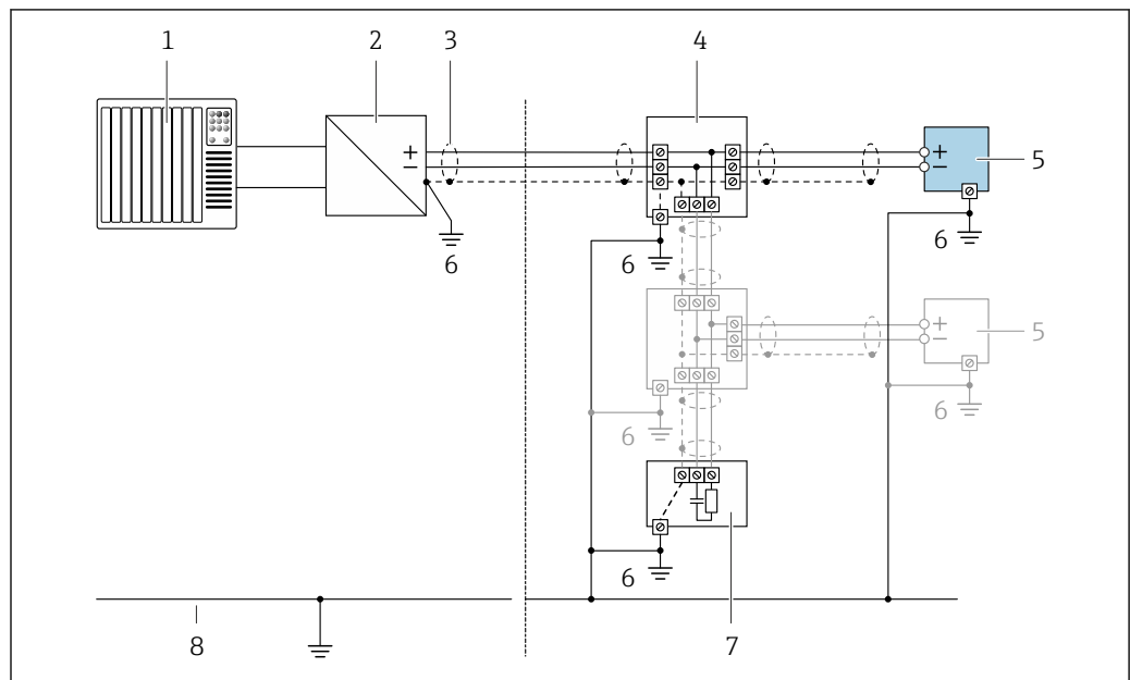
图 17 PROFIBUS PA 的接线实例
