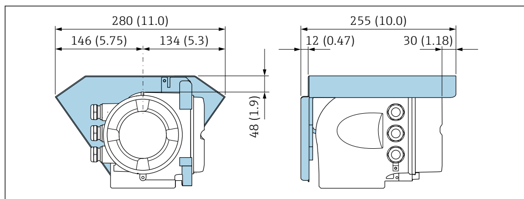
11 Tampa de proteção contra tempo para Proline 500; unidade de engenharia mm (pol.)
