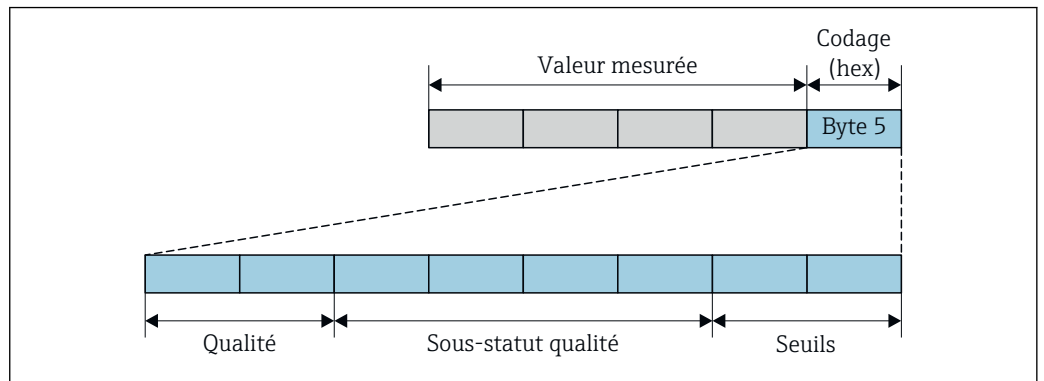
40 Structure de l'octet de codage
