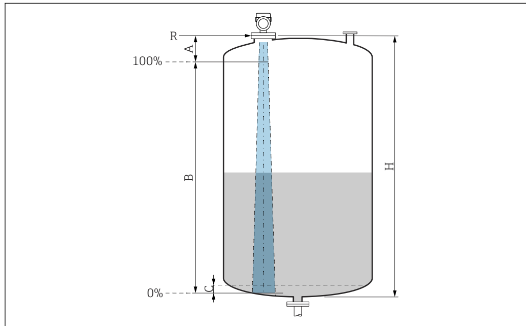
图 21 有效测量范围
