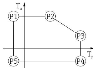
▣ 58 316L 外壳, 卫生型; 过程温度: -60 ... +150 °C (-76 ... +302 °F)
