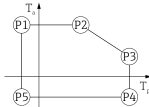
图 54 316L 外壳, 卫生型; 过程温度范围: -20 ... +150 °C (-4 ... +302 °F)
