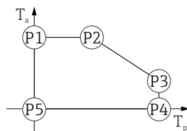
图 37 塑料外壳; 过程温度: 0 ... +200 °C (+32 ... +392 °F), 针对 CSA C/US 认证型仪表
