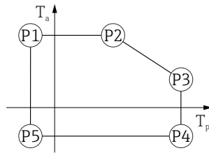
▣ 51 316L 外壳; 过程温度: -40 ... +450 °C (-40 ... +842 °F)
