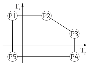
▣ 52 316L 外壳; 过程温度: -60 ... +150 °C (-76 ... +302 °F)
