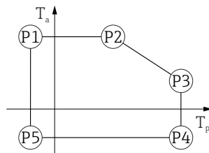
▣ 46 316L 外壳；过程温度范围：-20 ... +150 °C (-4 ... +302 °F)
