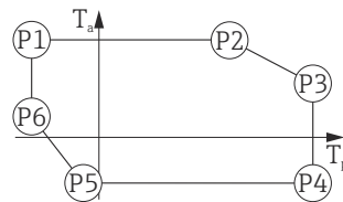
图 36 塑料外壳; 过程温度: -196 ... +200 °C (-320 ... +392 °F)
