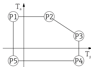
▣ 34 塑料外壳; 过程温度: -60 ... +150 °C (-76 ... +302 °F)
