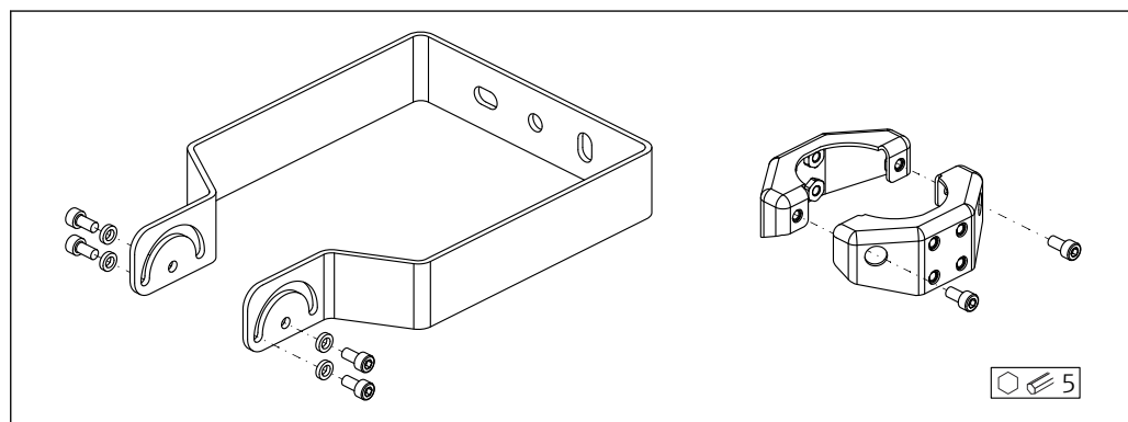
23 Fornitura; staffa di montaggio regolabile FMR6xB
