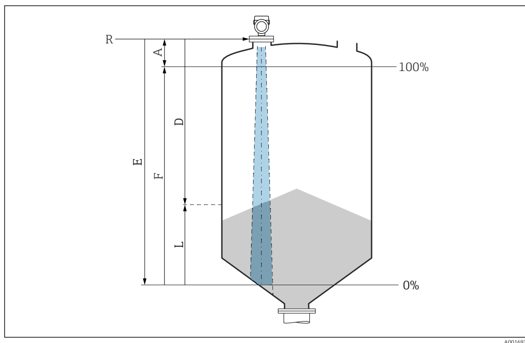
13 Parametri di configurazione per la misura di livello nei solidi sfusi
