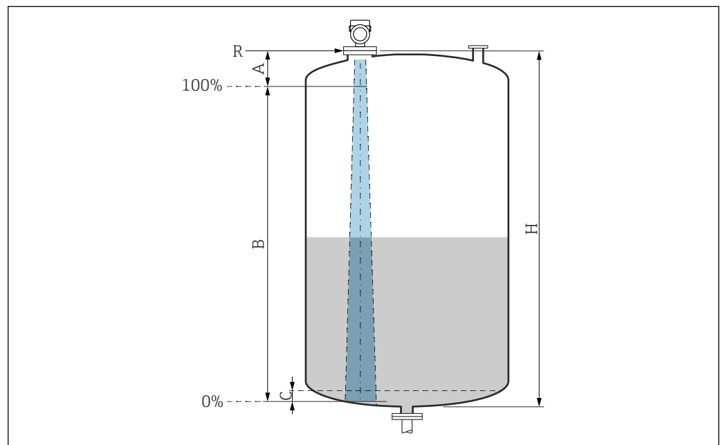
图 24 有效测量范围
