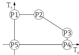
图 26 塑料外壳; 过程温度范围: 0 \dots +150 \text{ }^\circ\text{C} ( +32 \dots +302 \text{ }^\circ\text{F} ), 适用 CSA C/US 认证型仪表
