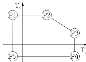
图 27 塑料外壳; 过程温度范围: -20 \dots +200 \text{ }^\circ\text{C} ( -4 \dots +392 \text{ }^\circ\text{F} )
