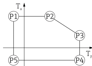
☐ 39 铝外壳, 带涂层; 过程温度范围: -40 ... +80 °C (-40 ... +176 °F)
