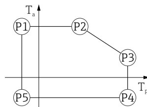
▣ 45 316L 外壳; 过程温度范围: -40 ... +80 °C (-40 ... +176 °F)
