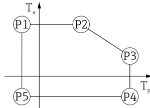
▣ 44 316L 外壳, 卫生型; 过程温度范围: -40 ... +80 °C (-40 ... +176 °F)
