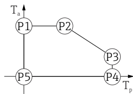
▣ 33 塑料外壳; 过程温度: 0 ... +450 °C (+32 ... +842 °F), 针对 CSA C/US 认证型仪表
