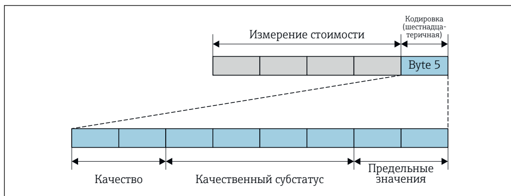
15 Структура байта состояния
