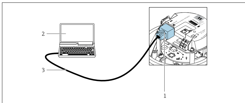
19 Подключение для кода заказа «Выход», опция R: PROFINET
