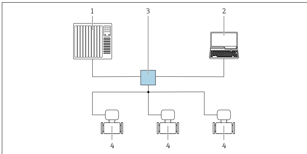
13 Варианты дистанционного управления через сеть PROFINET: топология «звезда»
