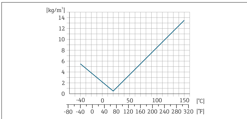
16 Калибровка по плотности на месте эксплуатации, в примере – при температуре +20 °C (+68 °F)
