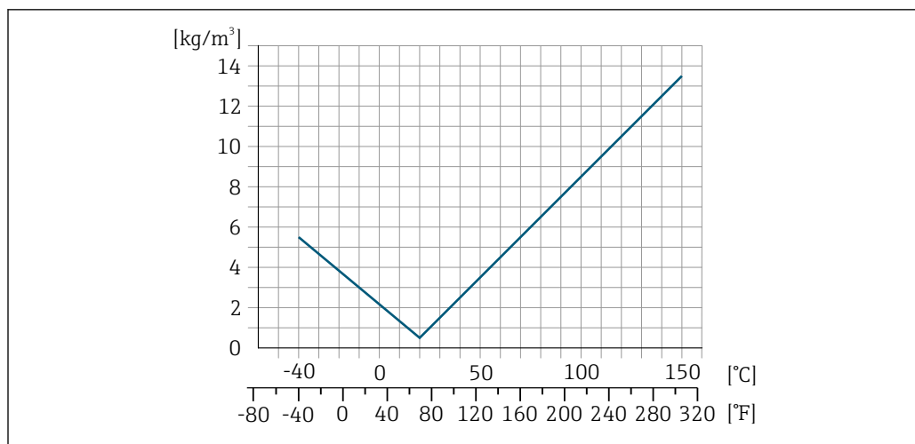
15 Калибровка по плотности на месте эксплуатации, в примере – при температуре +20 °C (+68 °F)
