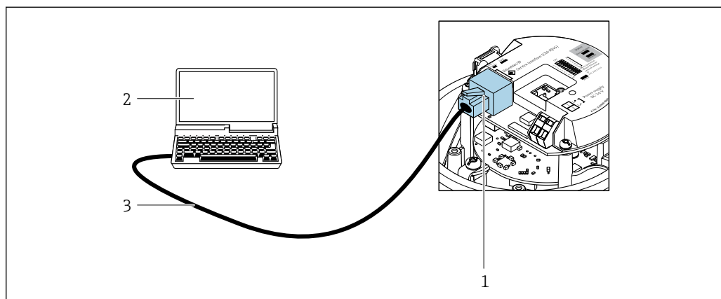
18 Подключение для кода заказа «Выход», опция N «Ethernet/IP»
