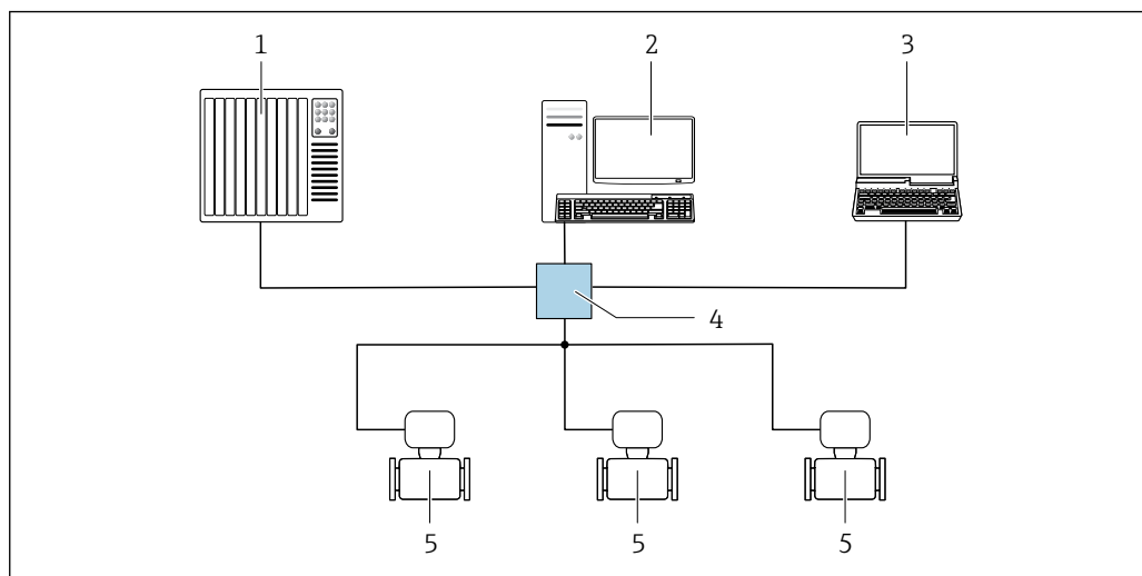
17 Варианты дистанционного управления через сеть EtherNet/IP: топология «звезда»
