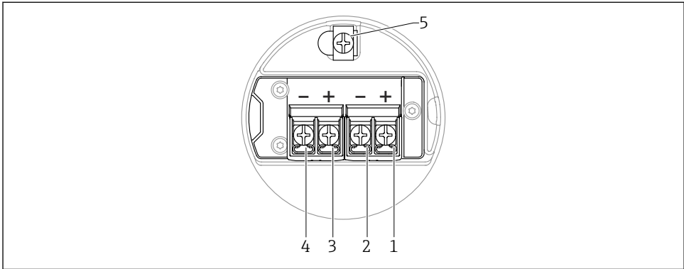
图 11 接线腔中的接线端子分配; 4 ... 20 mA HART, 开关量输出, 双腔室外壳
