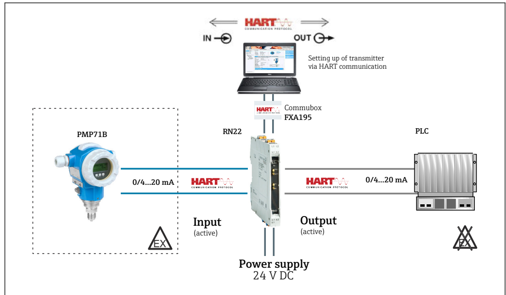
图 16 使用 RN22 有源安全栅/隔离器进行防爆危险区压力测量
