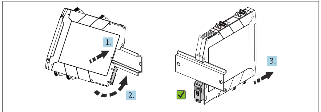
图 9 在 DIN 导轨上安装设备
