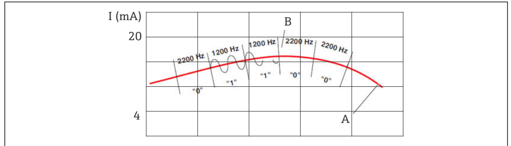
图 15 调制 HART 信号
