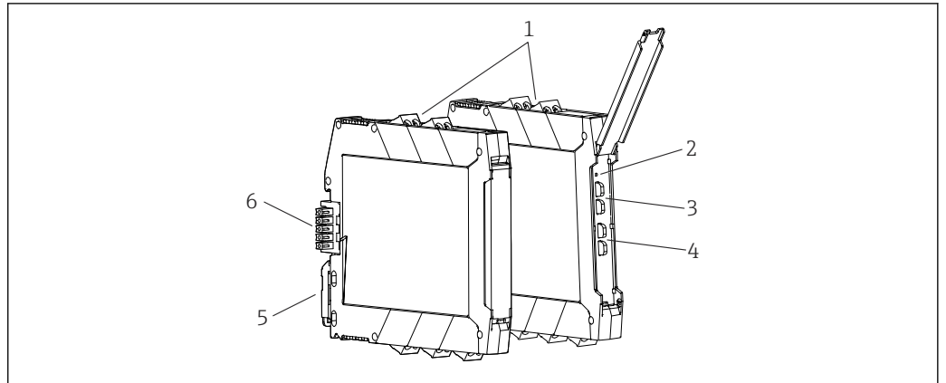
图 10 显示与操作部件
