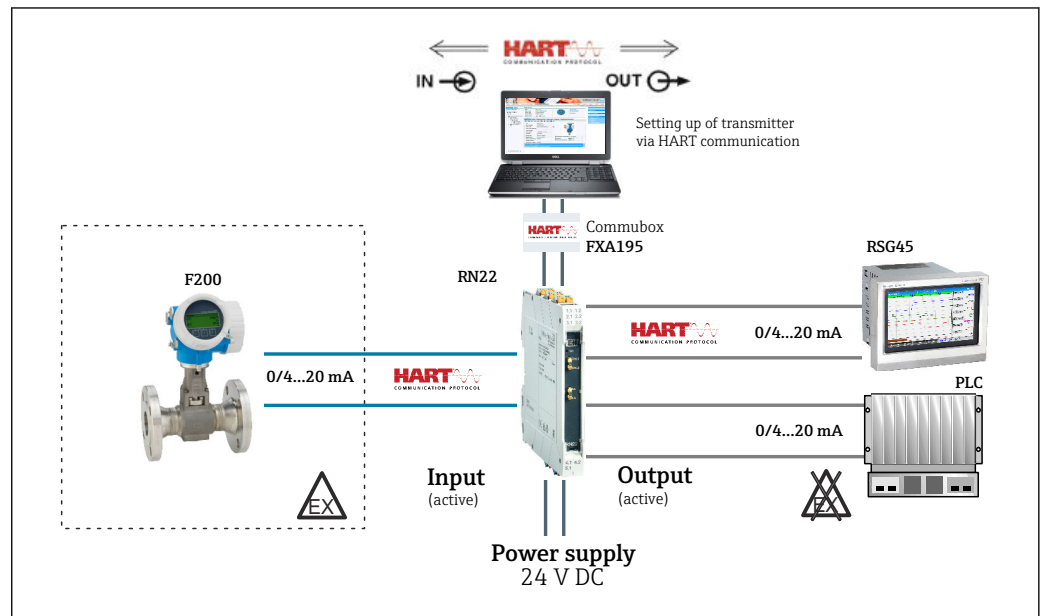
图 18 使用 RN22 信号倍增器进行防爆危险区流量测量
