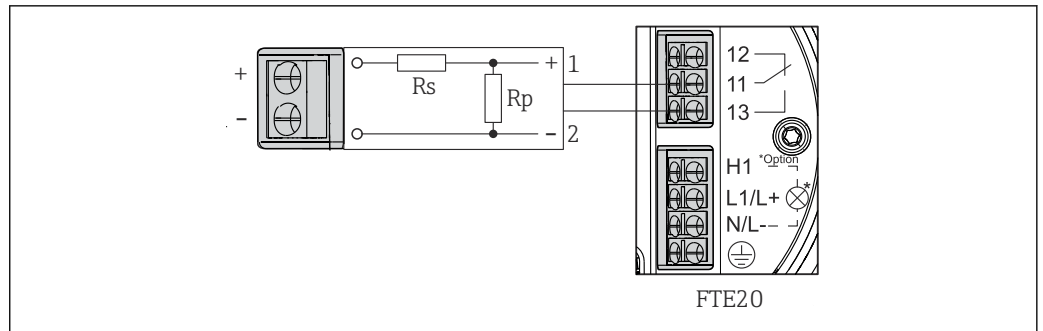
图 21 电阻回路，用于监测线路状态（短路和断路）
