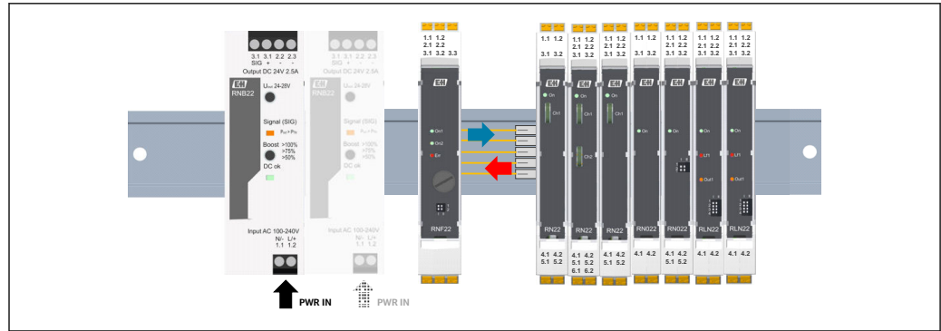
图 13 通过“可选的冗余”RNB22 系统电源和 RNF22 电源模块供电
