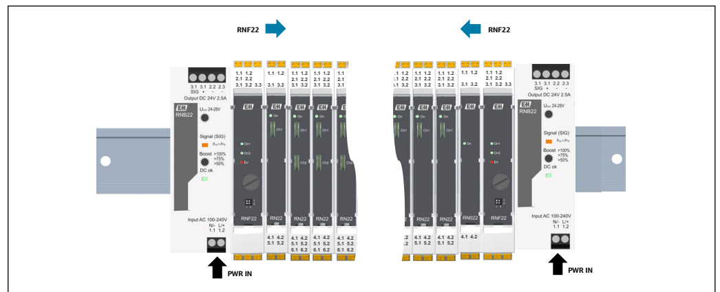
图 14 通过两个 RNF22 电源模块馈电的实例
