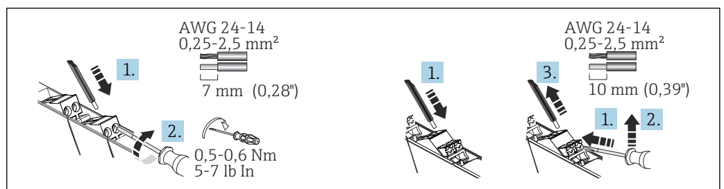
图 8 螺纹式接线端子 (左) 和直推式接线端子 (右) 电气连接图
