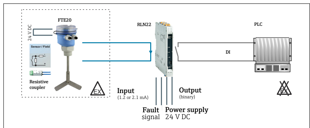
图 20 在防爆危险区对 FTE20 阻旋式物位开关进行 NAMUR 限定值检测，以及监测线路状态
