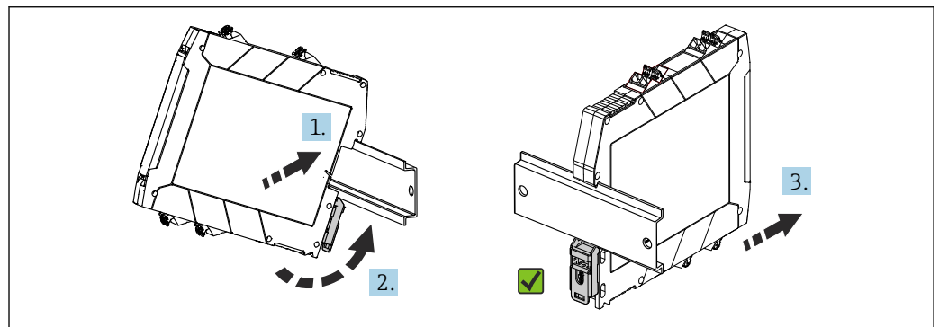
图 2 在 DIN 导轨上安装设备
