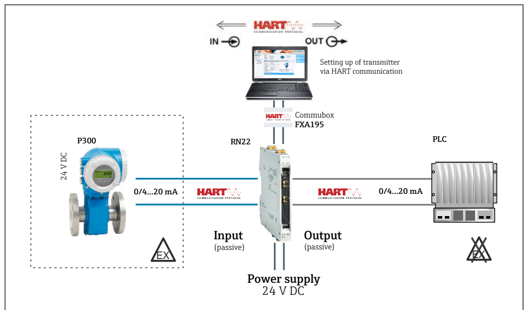
图 17 使用 RN22 有源安全栅/隔离器进行防爆危险区流量测量
