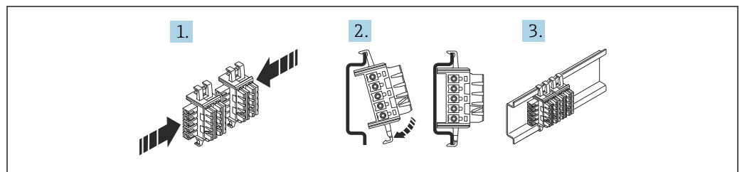
图 1 安装 DIN 导轨总线接头 12.5 mm (0.5 in)
