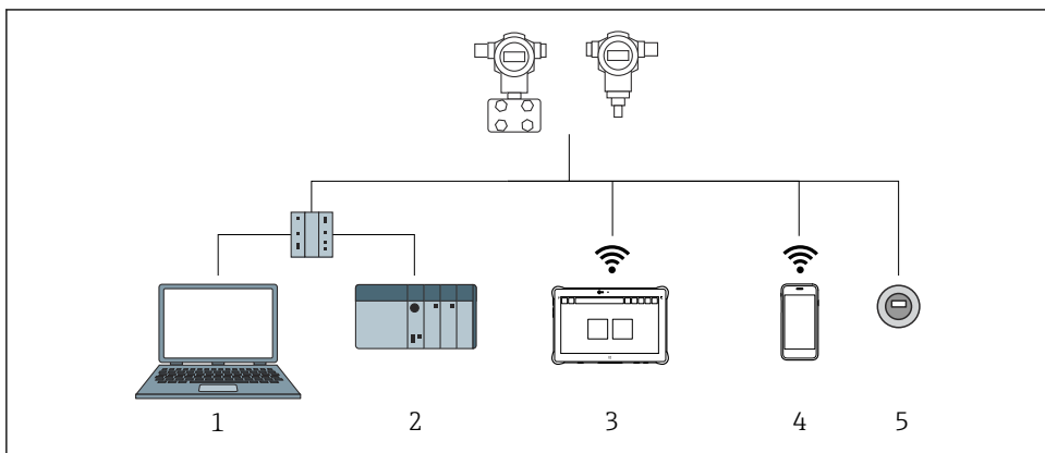
図 12 PROFINET プロトコル経由のリモート操作オプション
