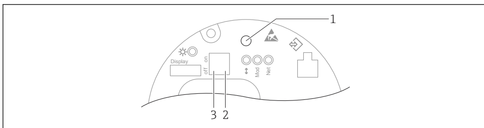
図 6 Ethernet-APL エレクトロニックインサート上の操作キーおよび DIP スイッチ
