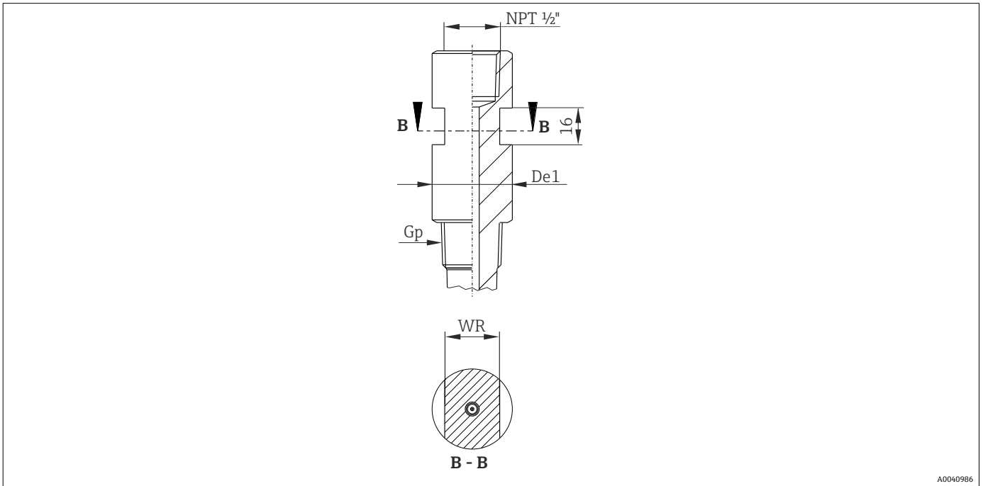
螺纹式保护套管的 De1 尺寸表, 单位: mm (in)
