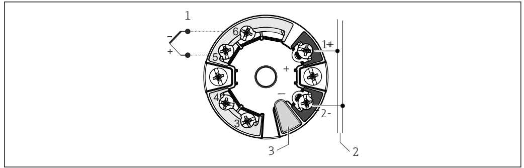
图 11 模块化变送器 iTHEMPT MT7x (单路传感器输入)
