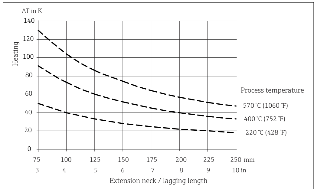
图 23 接线盒受热与过程温度的关系曲线。接线盒温度 = 环境温度 20 °C (68 °F) + ΔT
