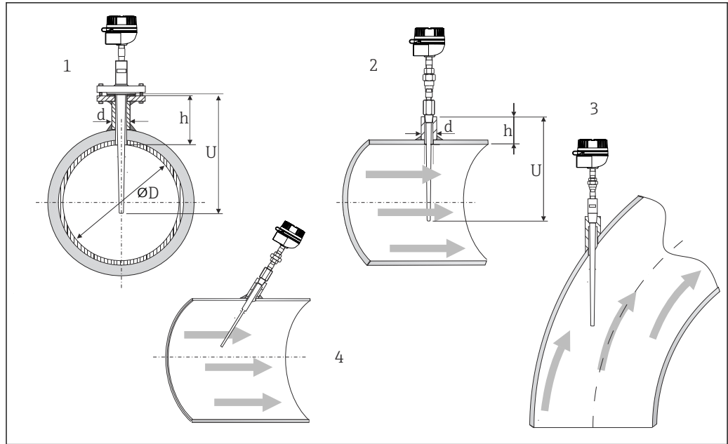
图 14 安装实例
