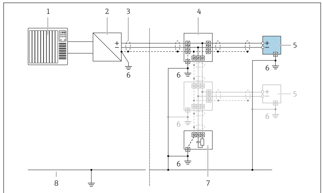
11 Exemplo de conexão para FOUNDATION Fieldbus
