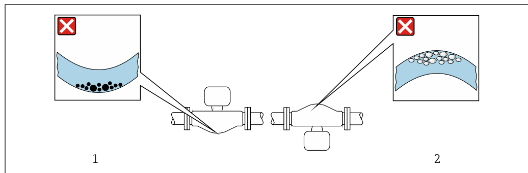
☑ 6 Position du capteur avec tube de mesure courbé
